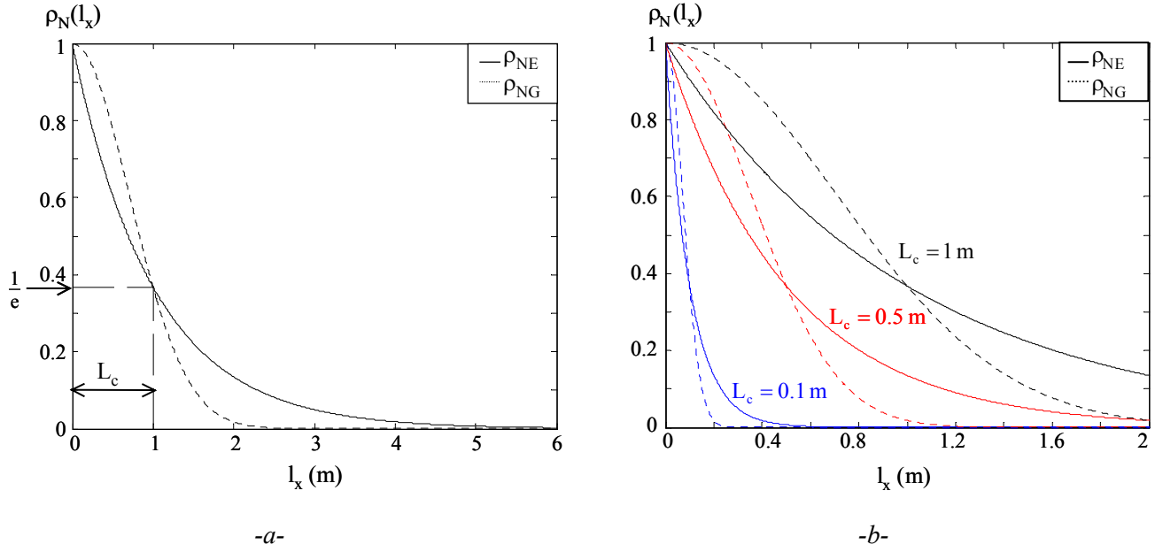
Figure II.4 Fonctions d'autocorrélation 1D gaussienne et exponentielle
