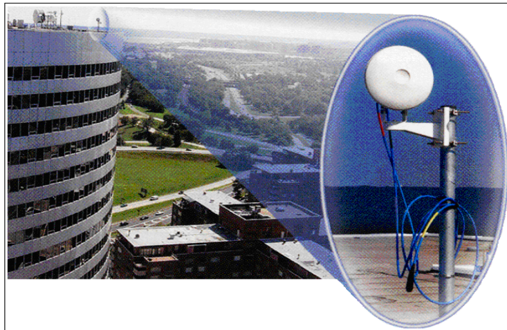
Figure 1.1 : Photographie d'une Station de Base (BTS) implantée au-dessus d'un toit d'immeuble et comportant une antenne dédiée à la Boucle Locale Radio 190 (BLR)
