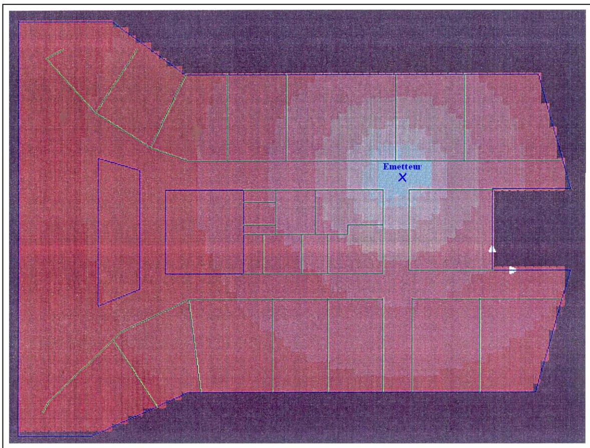
Figure 104 : Exemple de couverture de champ radioélectrique calculée avec un modèle en distance
