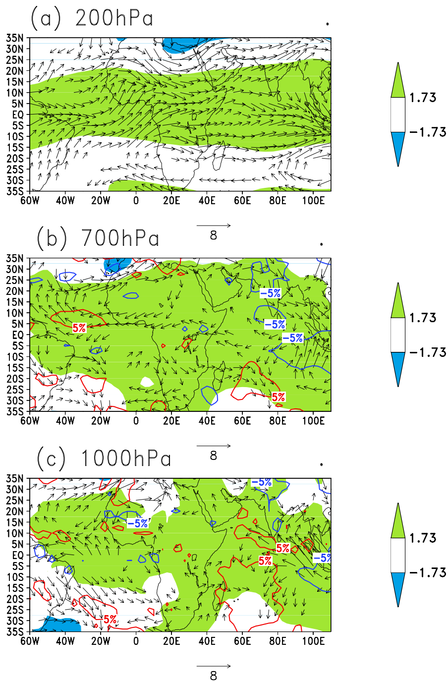
FIG. 8.7 – Composites "chaud-froid" de champs atmosphériques NCEP associés aux TSO du Pacifique équatorial oriental en juillet-septembre (1968-1997)
