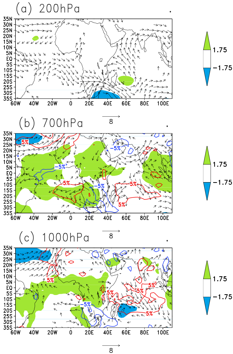
FIG. 8.21 – Composites "sec-humide" de champs atmosphériques NCEP associés aux précipitations en Afrique australe en janvier-mars (1968-1997)
