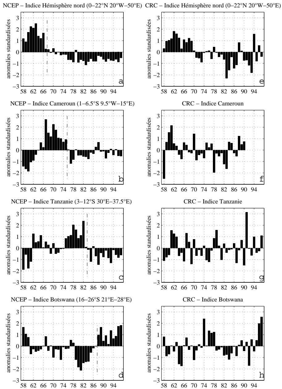
FIG. 4.3 – Indices régionaux de précipitations annuelles pour quatre espaces africains enregistrant une rupture d'homogénéité (1958-1997)
