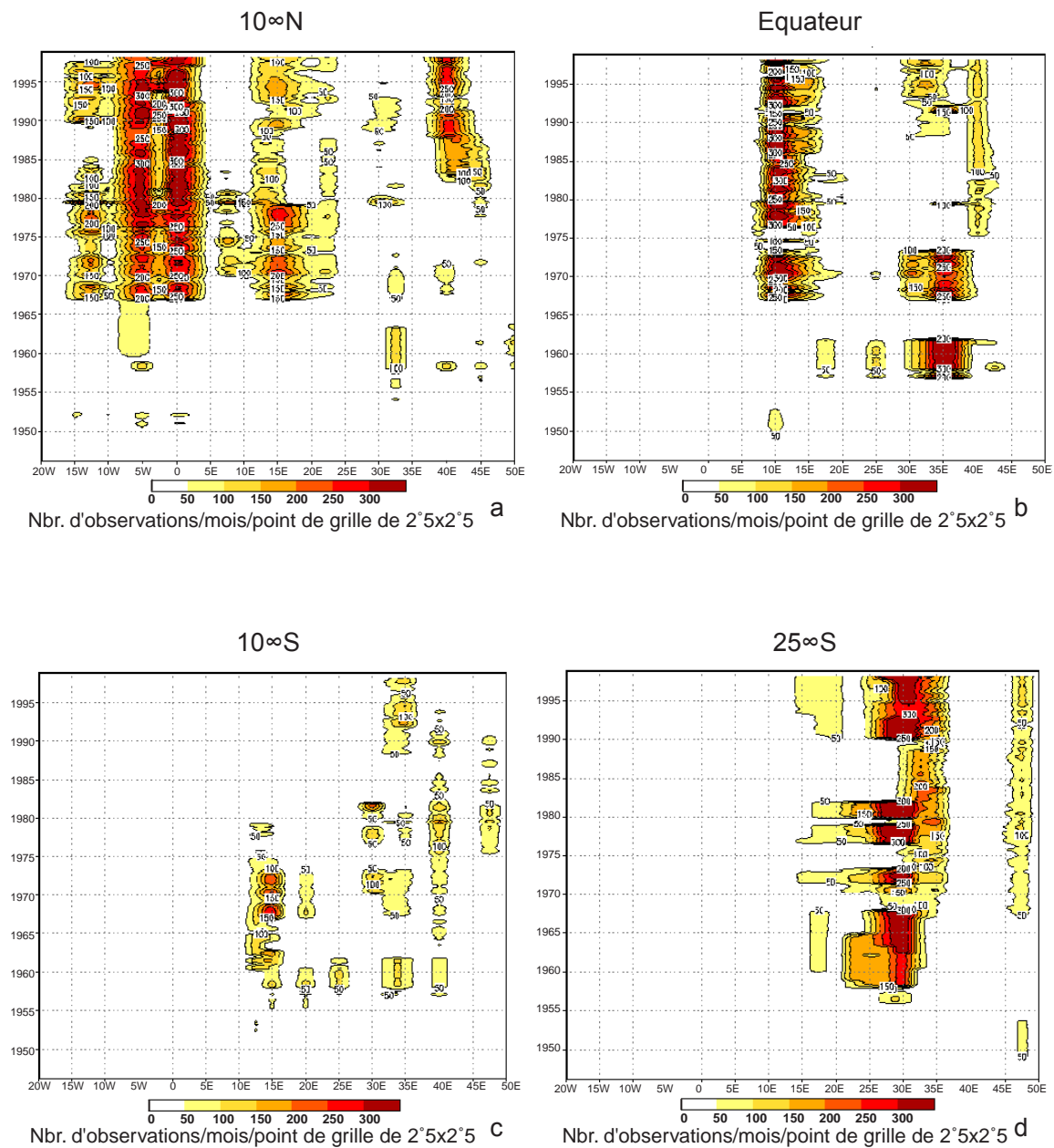
FIG. 5.10 – Densité des données en surface en Afrique tropicale intégrée dans le modèle du NCEP (1946-1998)
