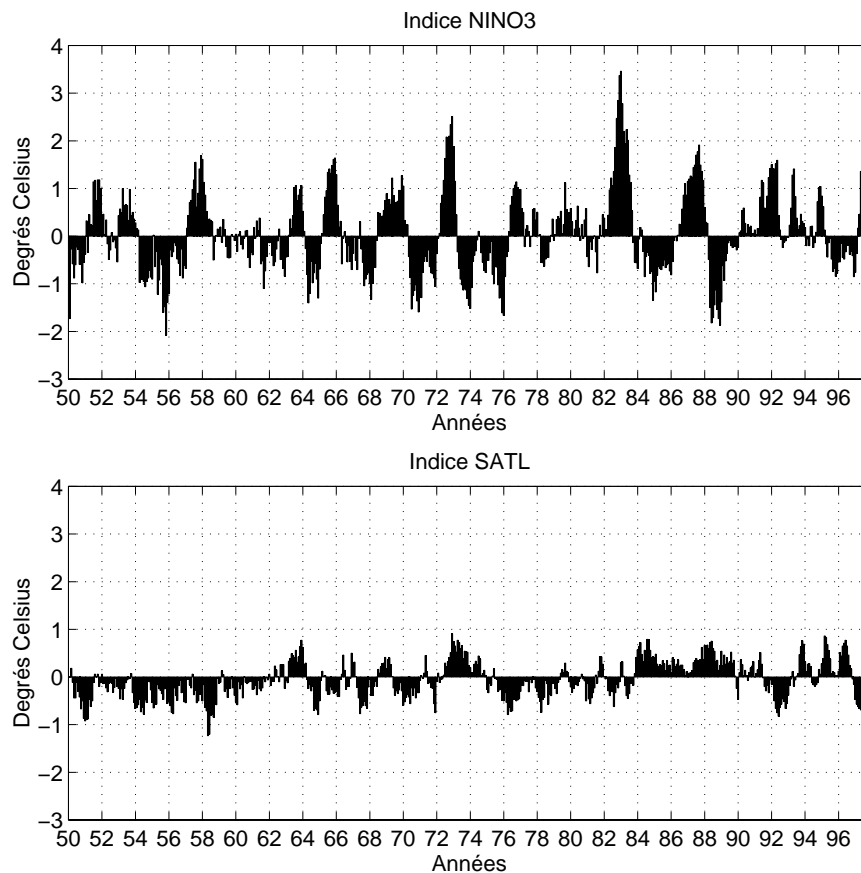
FIG. 2.3 – Variabilité interannuelle des deux indices de température de surface océanique (1950-1997)
