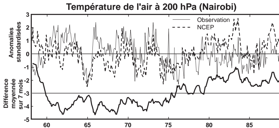
FIG. 5.14 – Température de l'air à 200 hPa à Nairobi (1958-1990)
