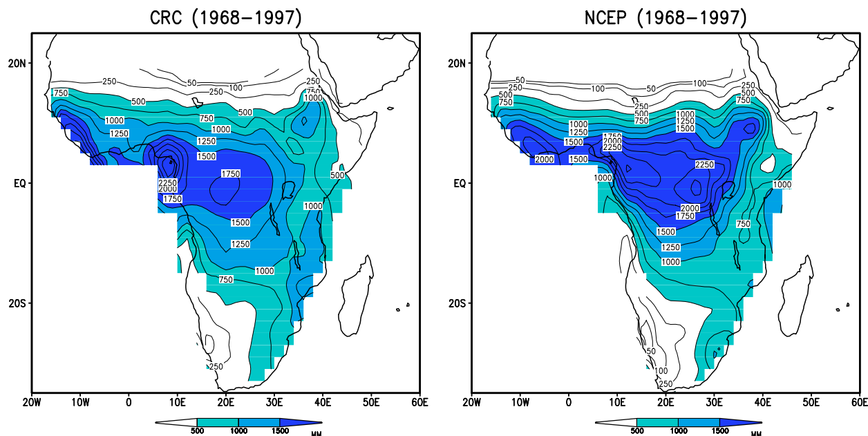
FIG. 4.4 – Précipitations moyennes annuelles CRC et NCEP en Afrique tropicale (1968-1997)
