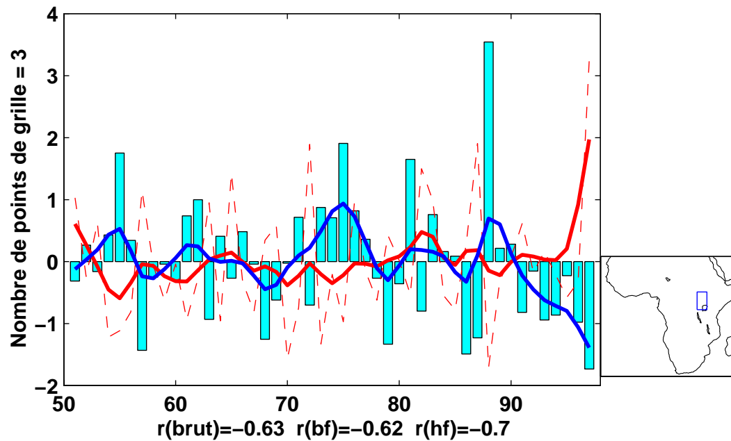
FIG. 7.7 – Anomalies standardisées des précipitations moyennées sur trois mois en Afrique orientale et de l'ENSO en juillet-septembre (1951-1997)
