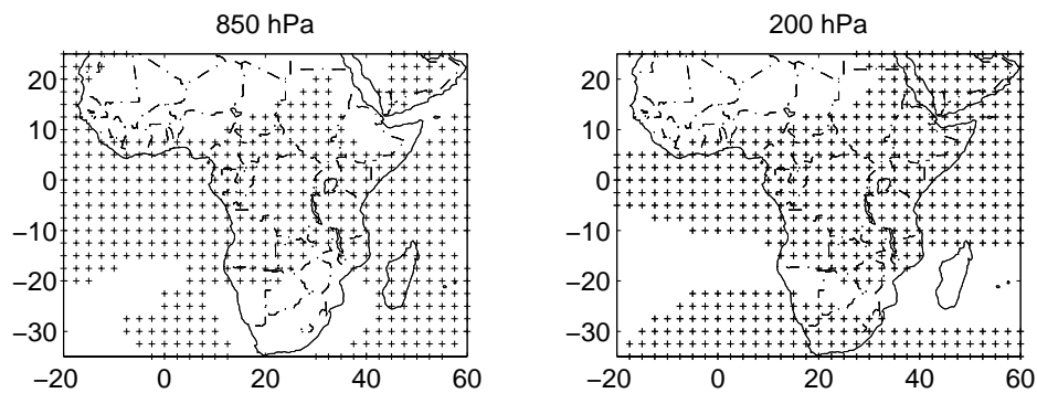
FIG. 5.4 – Localisation de la rupture de 1976/1977 dans la hauteur géopotentielle à 850 et 200 hPa
