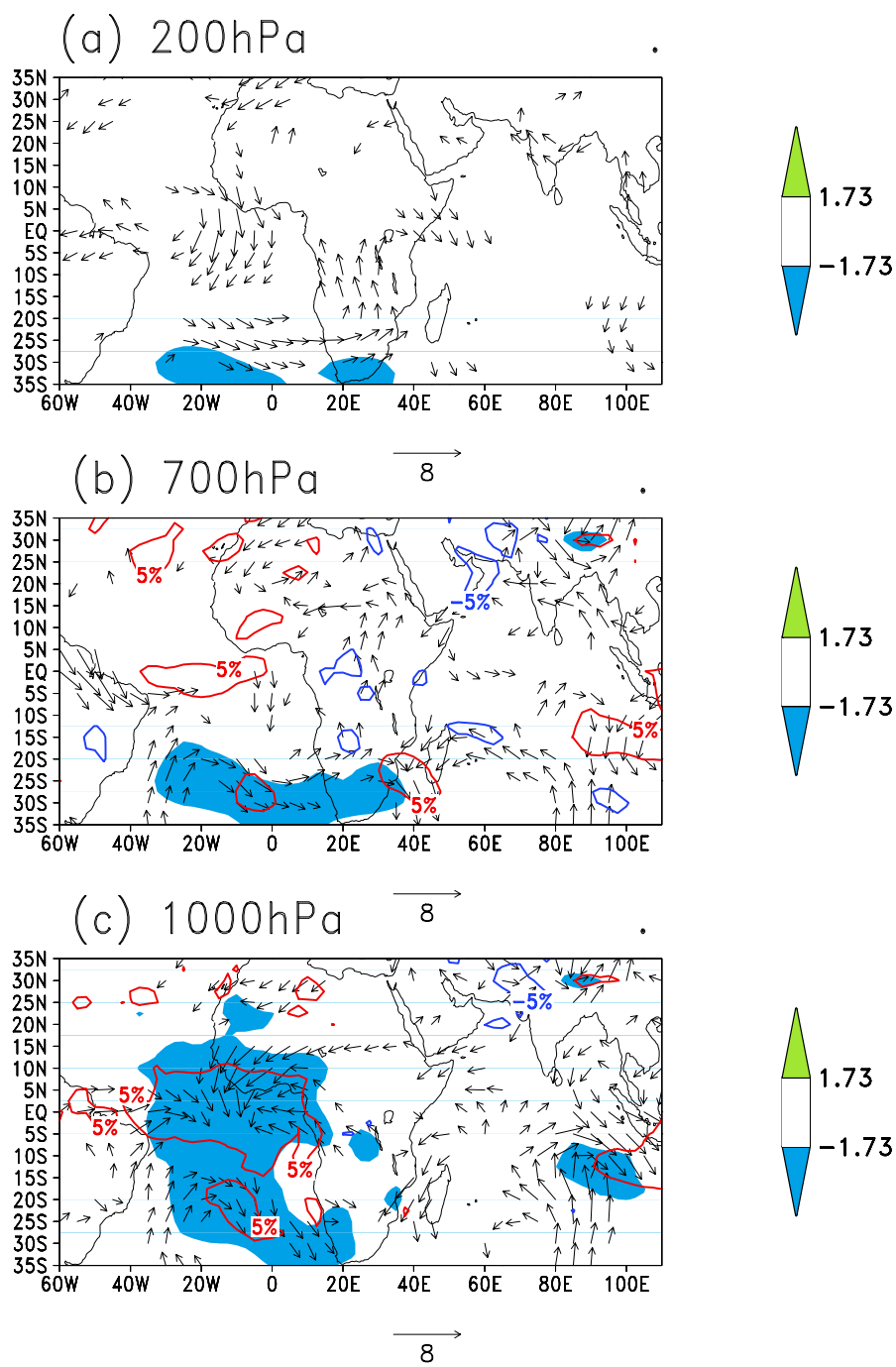
FIG. 8.10 – Composites "humide-sec" de champs atmosphériques NCEP associés aux précipitations dans la zone guinéenne en juillet-septembre (1968-1997)
