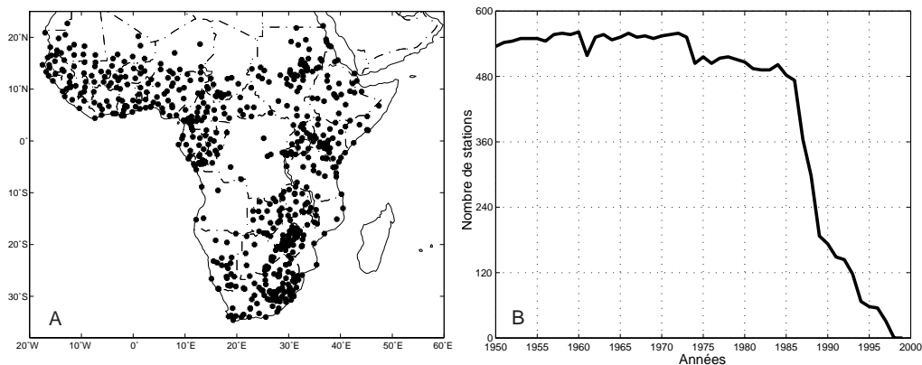
FIG. 2.1 – Base de données pluviométriques "CRC Afrique tropicale " (1951-1999)
