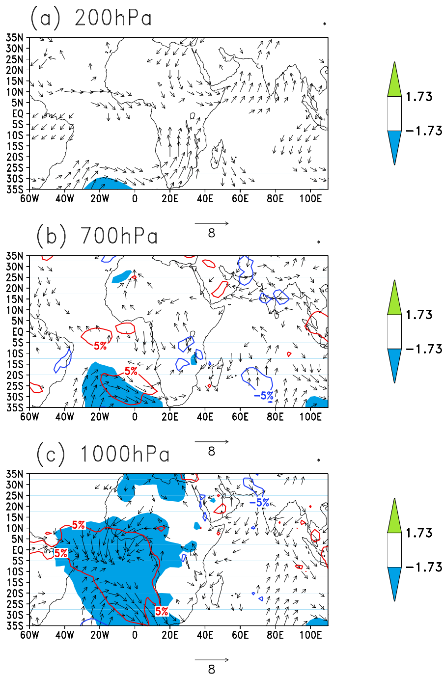
FIG. 8.6 – Composites "chaud-froid" de champs atmosphériques NCEP associés aux TSO de l'océan Atlantique tropical sud en juillet-septembre (1968-1997)
