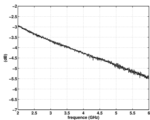
(b) S12
