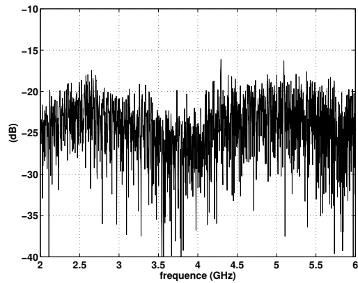
(d) S22
