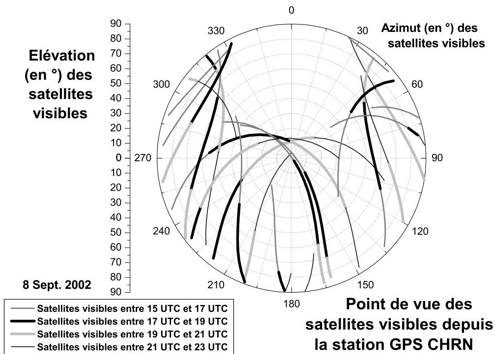
FIG. 3.2 – Répartition des trajectoires des satellites à la station de Château-Renard (CHRN de latitude Nord 43.881^\circ , de longitude Est 4.862^\circ et d'altitude 103.031 m).
