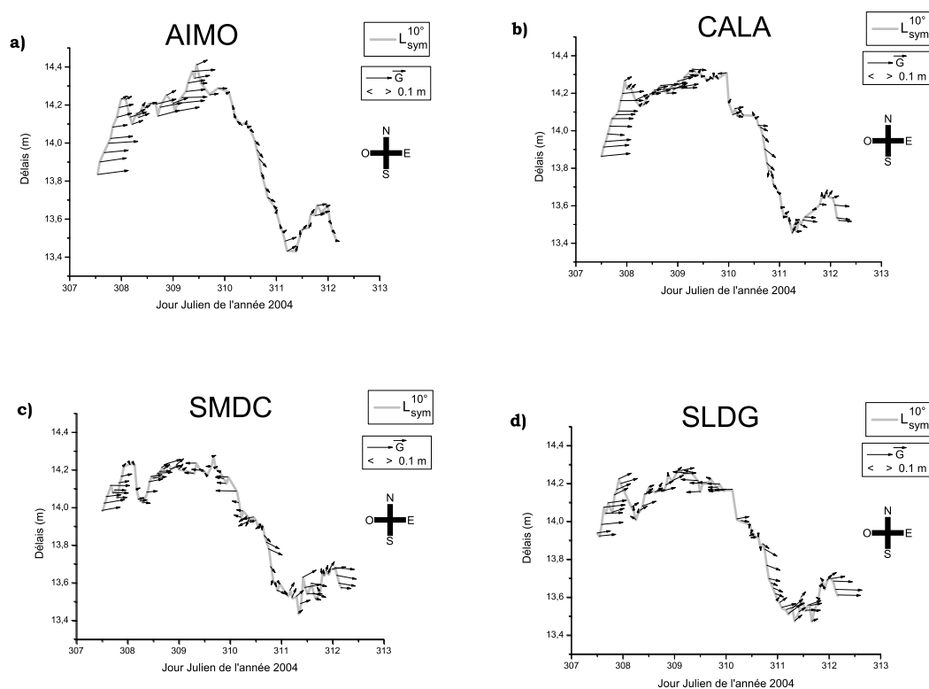
FIG. 1.25 – Séries temporelles de délais isotropes L_{sym}^{10^\circ} et des gradients associés \vec{G} estimés aux stations a) de Aigues-Mortes (AIMO), b) de Calabrun proche des Sainte-Marie-de-la-Mer (CALA), c) de Saint-Martin-de-Croc (SMDC) et d) de Salins-de-Girault (SLDG) du 3 au 9 novembre 2004 (du jour Julien 307 au jour 313). Graphiques similaires à celui de la Figure 1.16.
