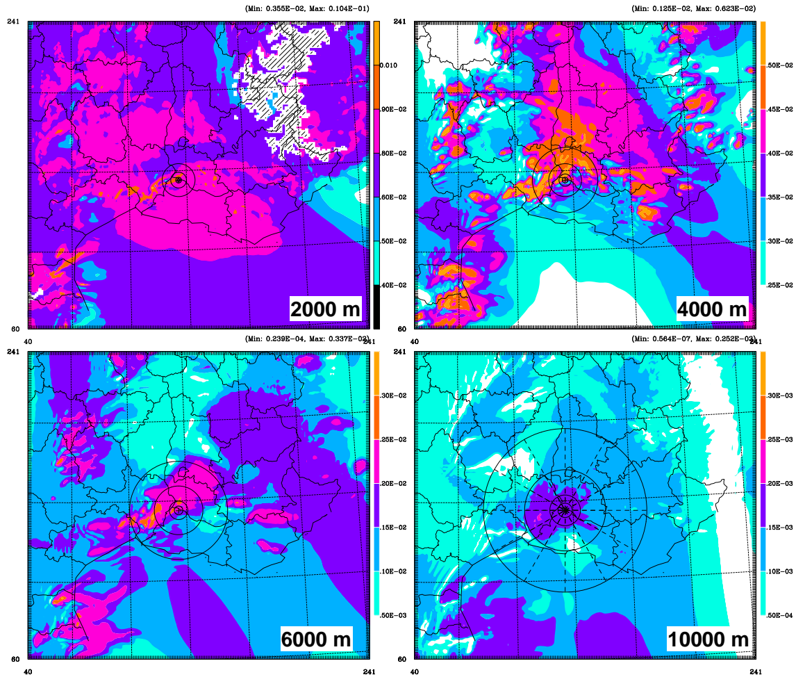
FIG. 3.7 – Rapport de mélange en vapeur d’eau (kg/kg) à différentes altitudes pour la simulation Més0-NH RAD12 à 15h UTC le 8 septembre 2002. Les cercles correspondent du plus extérieur au plus intérieur à l’intersection avec les plans des coupes horizontales des cônes à partir de la station de Château-Renard d’ouvertures respectives 5°, 10°, 25° et 45°.
