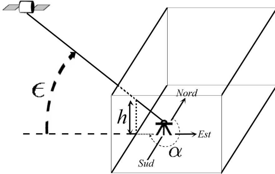
FIG. 3.1 – Simulation des STD dans le domaine fils de Més0-NH. Tir dans une direction d’élévation \epsilon par rapport à l’horizon et d’angle \alpha par rapport à la direction du Nord. La hauteur minimale ( h ) de la dernière altitude du calcul est un degré de liberté du calcul.
