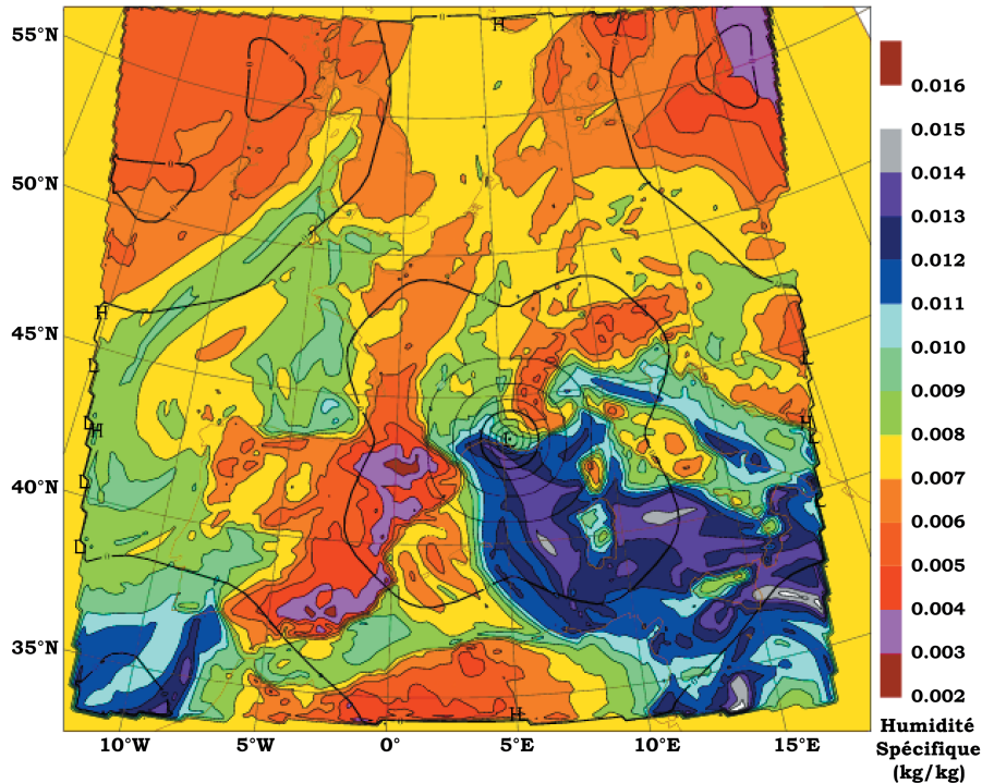
FIG. 5.2 – Analyse d’une observation de ZTD à la station d’Aix en Provence avec le 3Dvar ALADIN : humidité spécifique près du sol en plage de couleurs sur laquelle est superposé l’incrément d’analyse par pas de 0.1g/kg. L’écart à l’ébauche pour l’observation d’Aix en Provence est de 14 mm.
