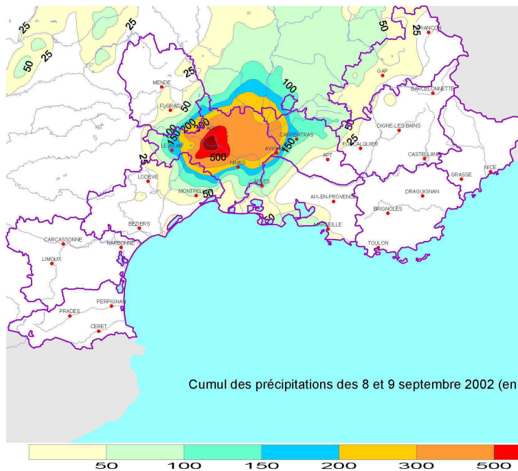
FIG. 1.4 – Cumul de précipitation enregistré lors de l'évènement des 8-9 septembre 2002. (source : Météo-France)
