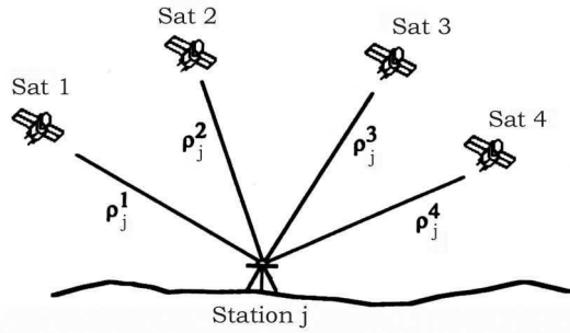
FIG. A.3 – Distances géométriques \rho_j^1 , \rho_j^2 , \rho_j^3 et \rho_j^4 entre les satellites GPS 1, 2, 3 et 4 et la station GPS j .
