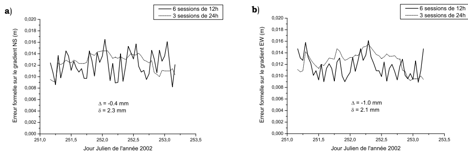
FIG. 2.9 – Comparaison des erreurs formelles GAMIT de a) G_{\text{NS}} , b) G_{\text{EW}} , les 8-9 septembre 2002 à la station CHRN pour le calcul de 6 sessions de 12h (référence statistique) et pour celui de 3 sessions de 24h.
