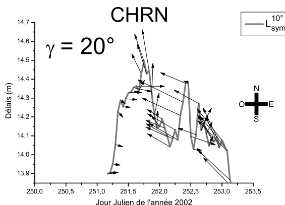
FIG. 2.5 – Série temporelle du délai isotrope L_{sym}^{10^\circ} et de ses gradients associés pour la station de CHRN les 8-9 septembre 2002. Le traitement GPS a été procédé avec un cutoff de 20^\circ .
