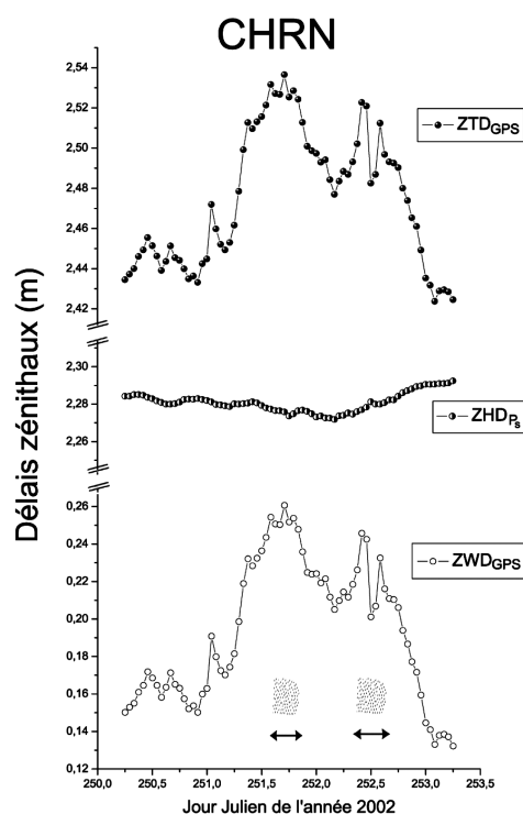
FIG. 1.14 – Séries temporelles du délai zénithal total ( ZTD_{GPS} ), du délai zénithal hydrostatique ( ZHD_{P_S} ), et du délai zénithal humide ( ZWD_{GPS} ), évalués à la station CHRN de Château-Renard (voir Figure 1.2 pour la position du site GPS). Le jour Julien 250 de l'année 2002 correspond au 7 septembre, le jour Julien 253 au 10 septembre. Les doubles flèches figurent les périodes de précipitations.
