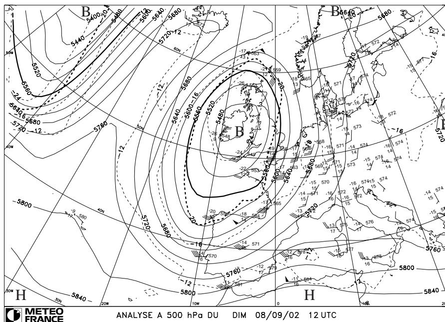
FIG. 1.5 – Analyse du 8 septembre 2002 à 12 UTC en surface (haut) et à 500 hPa (bas). Au pointage des observations sont superposés les géopotentiels (trait plein) et la température (trait tiret) à 500 hPa et la pression au niveau de la mer (trait plein) issus de l'analyse ARPEGE. (source : Météo-France)
