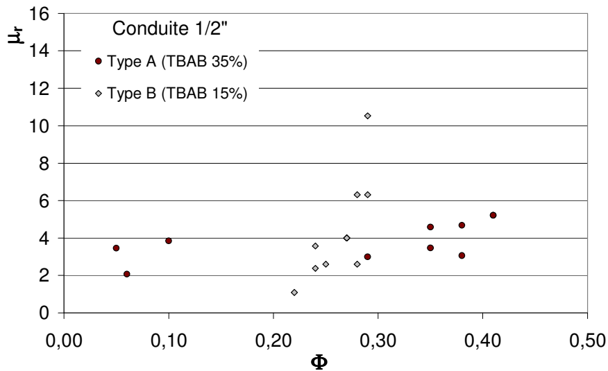
Figure 3.4-2 : Comparaison des viscosités relatives des coulis d'hydrates de TBAB de types A et B (Conduite 1/2 ")
