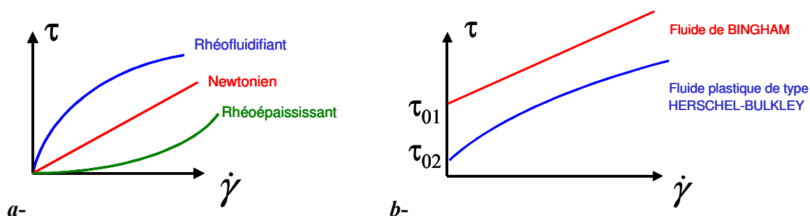
Figure 1.2-1 : Différents comportements rhéologiques des fluides a- Sans contrainte critique, b- Avec contrainte critique. (Midoux, 1993)
