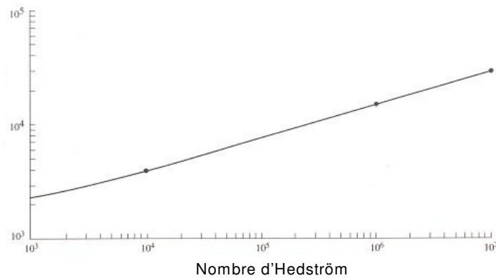
Figure 3.1-14 : Evolution du nombre de Reynolds critique en fonction du nombre d'Hedström pour une suspension modélisée comme un fluide de Bingham (Schetz et al. 1999)
