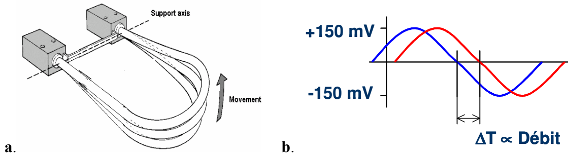
Figure 2.3-6 : Principe de fonctionnement du débitmètre Coriolis
