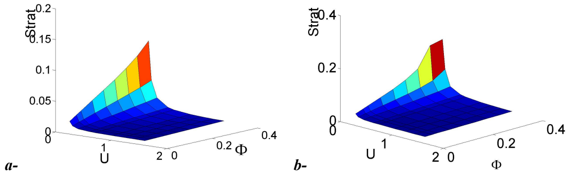
Figure 4.3-10 : Visualisation des régimes d'écoulement des coulis d'hydrates de TBAB en fonction des conditions d'écoulement ( D = 0,016 \text{ m} ). a- Hydrates de type A ( x_0 = 0,35 - D_p = 50 \text{ } \mu\text{m} ) b- Hydrates de type B ( x_0 = 0,15 - D_p = 25 \text{ } \mu\text{m} )
