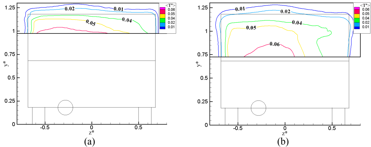
figure 4-15 : Ecart type de la température \langle T^{*2} \rangle^{1/2} : (a) x^* = -0,25 ; (b) x^* = 0 ; (c) x^* = 0,25 ; (d) x^* = 1 ; (e) x^* = 2 et (f) x^* = 5 pour \alpha = 40^\circ et U_\infty = 12,5 \text{ m.s}^{-1}
