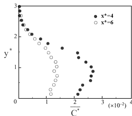
figure 1-22: Profils de concentration en aval de l'obstacle (Vinçont et al. [69])
