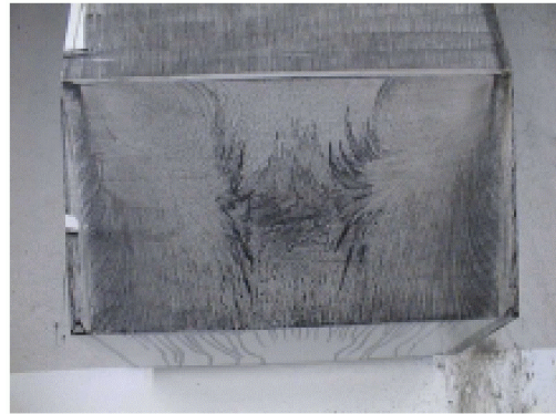
figure 1-12: Photographie des lignes de frottement sur la lunette arrière (Lienhart et Becker [48][49][50])
