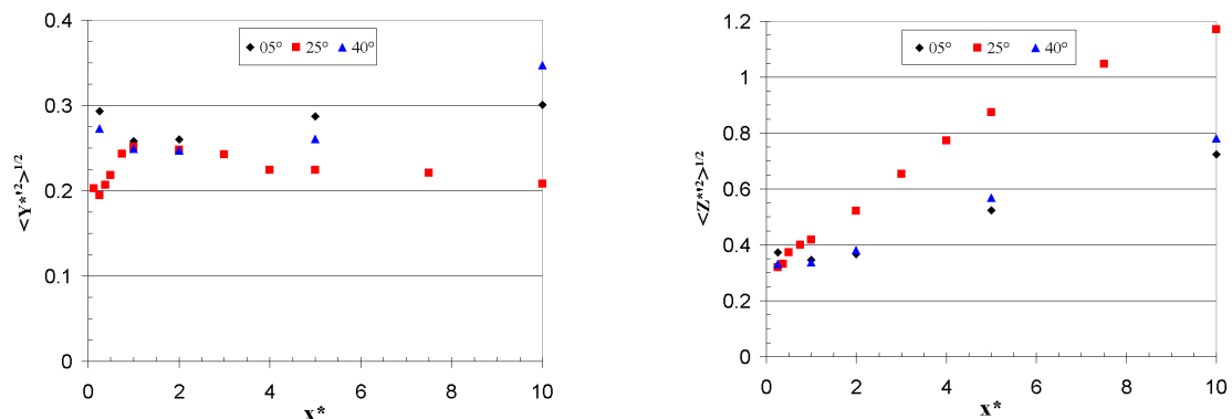
figure 5-28: Variations de \langle Y^{*2} \rangle^{1/2} et de \langle Z^{*2} \rangle^{1/2} en fonction de x^* et de \alpha
