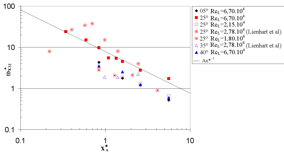
figure 3-36 : vorticité longitudinale moyenne \omega_{xM}^* en fonction du nombre de Reynolds Re_L , de l'angle \alpha et de x_+^*
