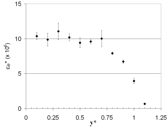
figure 5-39: Taux de dissipation total des fluctuations de température \varepsilon_{\theta}^* en fonction de y^* à x^*=2 et z^*=-0,40
