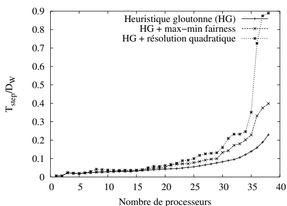
FIG. 3.11 – Première plate-forme.
