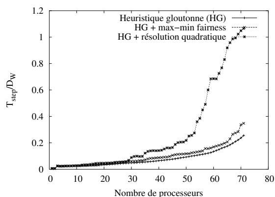
FIG. 3.12 – Deuxième plate-forme.
