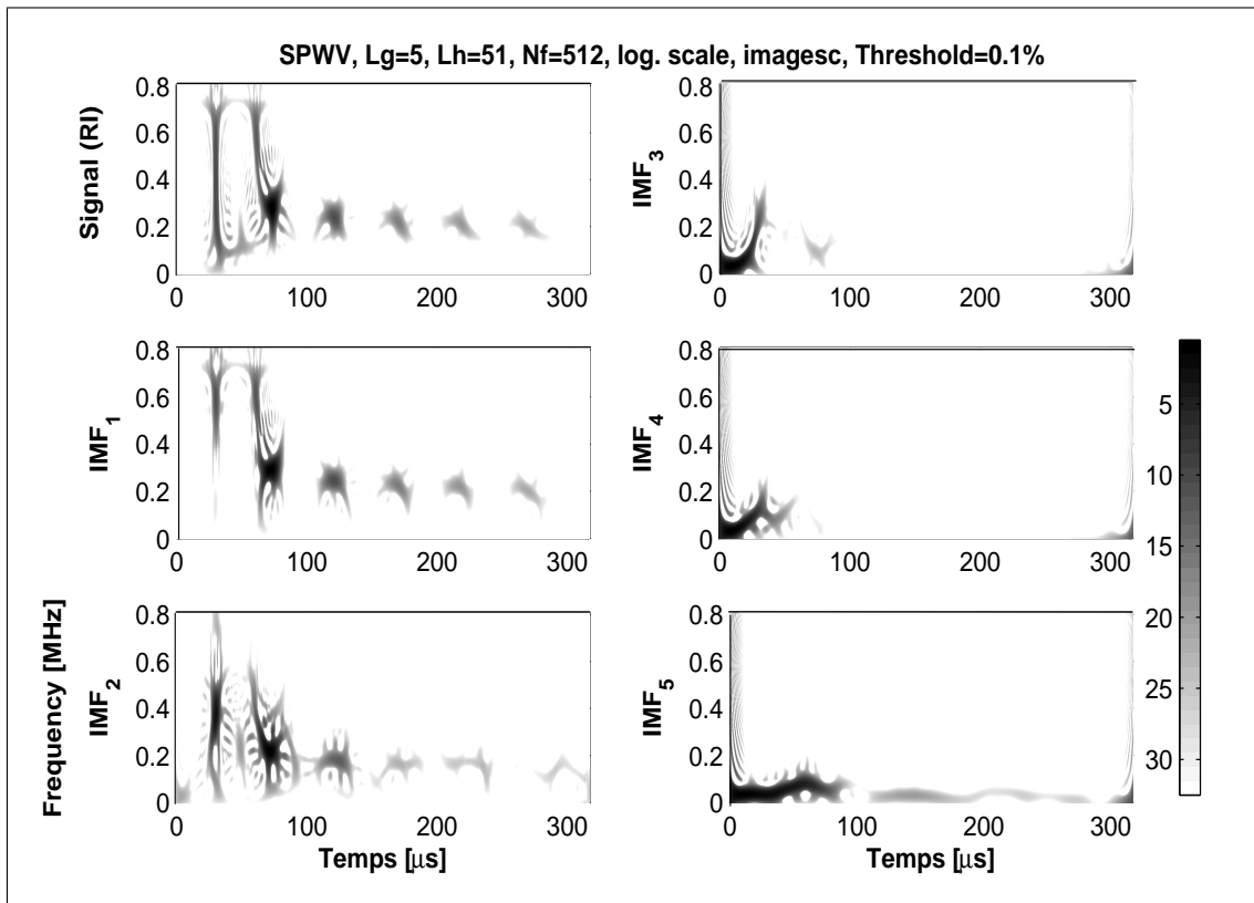
Figure VI.4 — Décomposition par EMD et densité spectrale d'énergie de chaque IMF de la RI d'une coque sphérique en Nickel-Molybdène ( a = 15\text{mm} , b/a = 0.94 , c_l = 5554\text{m/s} , c_t = 3021\text{m/s} , \rho = 9217\text{kg/m}^3 ).
