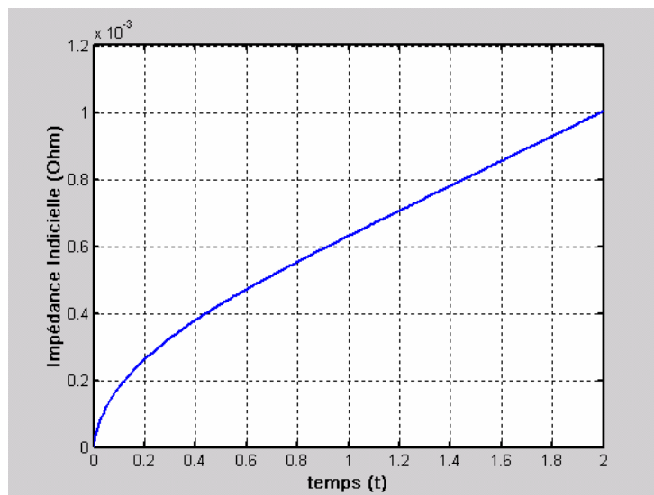
Fig. 2.27.: Impédance inductive d'une ligne de transmission( C=2700F, R=0.85m\Omega )
