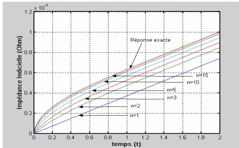
Fig. 2.34.: Simulation du modèle circuit d'une ligne de transmission ( C=2700F, R=0.85m\Omega )
