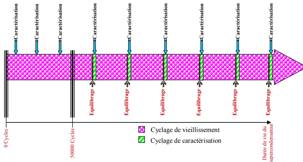
Fig. 3.54 : Utilisation de deux types différents de cycle pour l'étude de vieillissement
