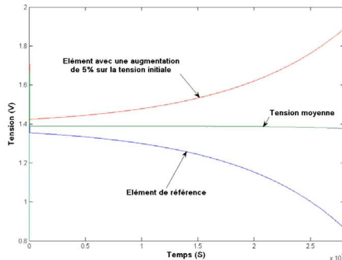
Fig. 4.18. : Variation de la tension de fin de cycle pour deux éléments supercondensateurs avec une différence de 5% de la tension initiale
