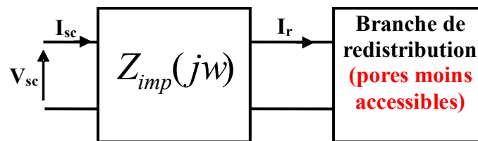
Fig. 2.16.: Utilisation des branches supplémentaires pour représenter la redistribution des charges
