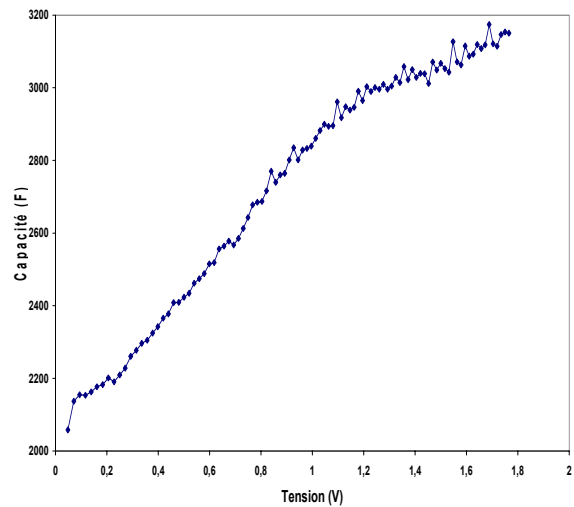
Fig. 2.37: Variation de la capacité en fonction de la tension
