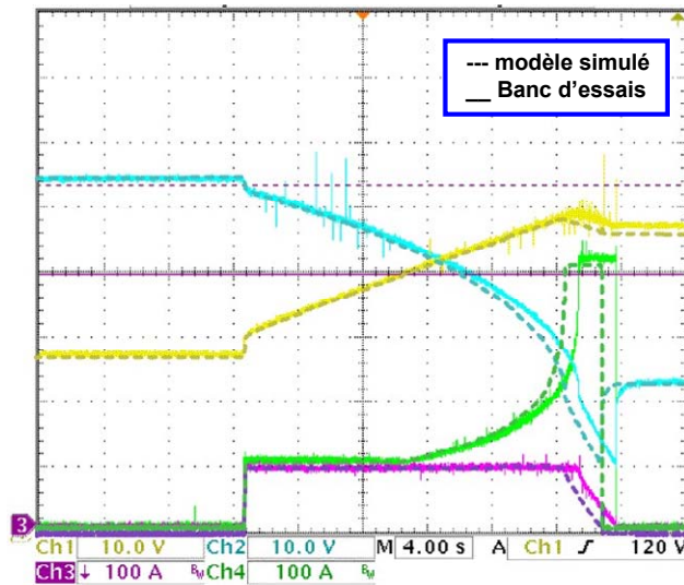
Fig. 3.23. : Validité du modèle simulé
