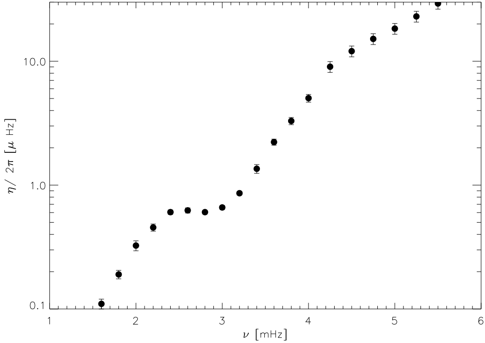
FIG. 2.5 – Taux d’amortissement ( \eta/2\pi ) des oscillations solaires mesuré par Libbrecht par ajustement du profil Lorentzien sur le spectre de puissance observé. Les points de mesures sont accompagnés de leur barre d’erreur respective.
