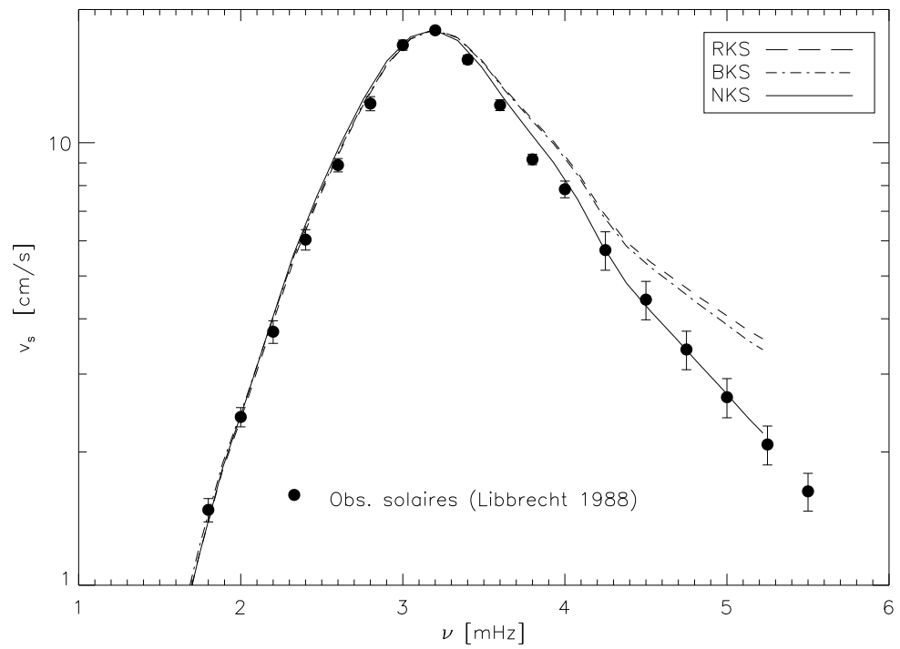
FIG. 5.3 – Estimations des vitesses des oscillations solaires calculées sur le modèle d'équilibre basé sur la MLT introduite par Gough. Les valeurs des paramètres \beta et \lambda ont été ajustées de manière à ajuster l'allure et l'amplitude maximale des vitesses aux vitesses spectroscopiques des données solaires. Les notations et considérations de la figure 5.2 ont été adoptées.
