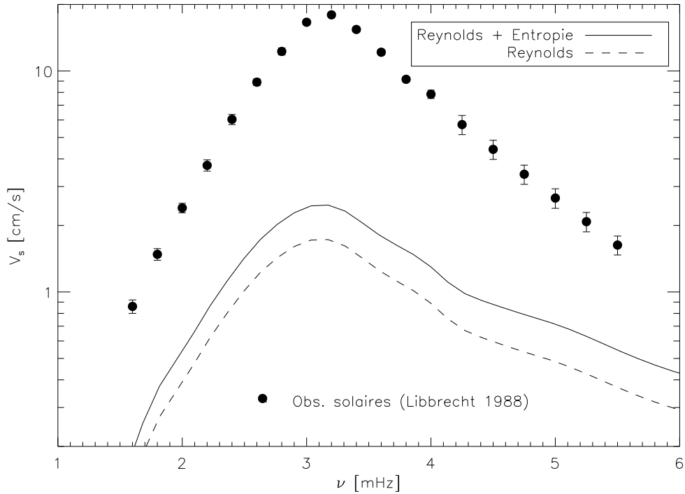
FIG. 5.1 – présente le calcul de v_s(\omega_0) effectué en considérant les sources termes de l'entropie et de Reynolds (courbe continue) et la seule contribution du terme de Reynolds (courbe discontinue). Le spectre de turbulence utilisé ici est le spectre de Kolmogorov (KS) et le modèle solaire considéré est basé sur la MLT classique. Les amortissements utilisés dans le calcul de v_s sont les amortissements mesurés. Les cercles pleins accompagnés des barres d'erreur respectives représentent les données solaires de Libbrecht [1988].
