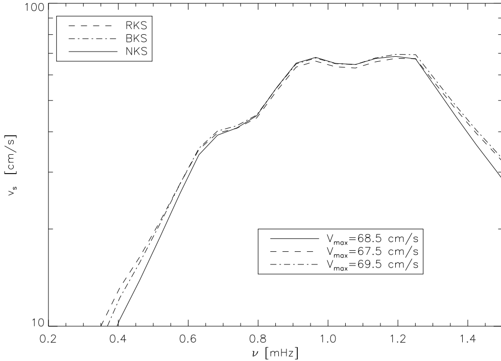
FIG. 6.9 – Vitesses des oscillations prédites pour le modèle d'équilibre de Procyon basé sur le traitement non-local et dépendant du temps de la MLT de Gough. Différents spectres turbulents sont envisagés.
