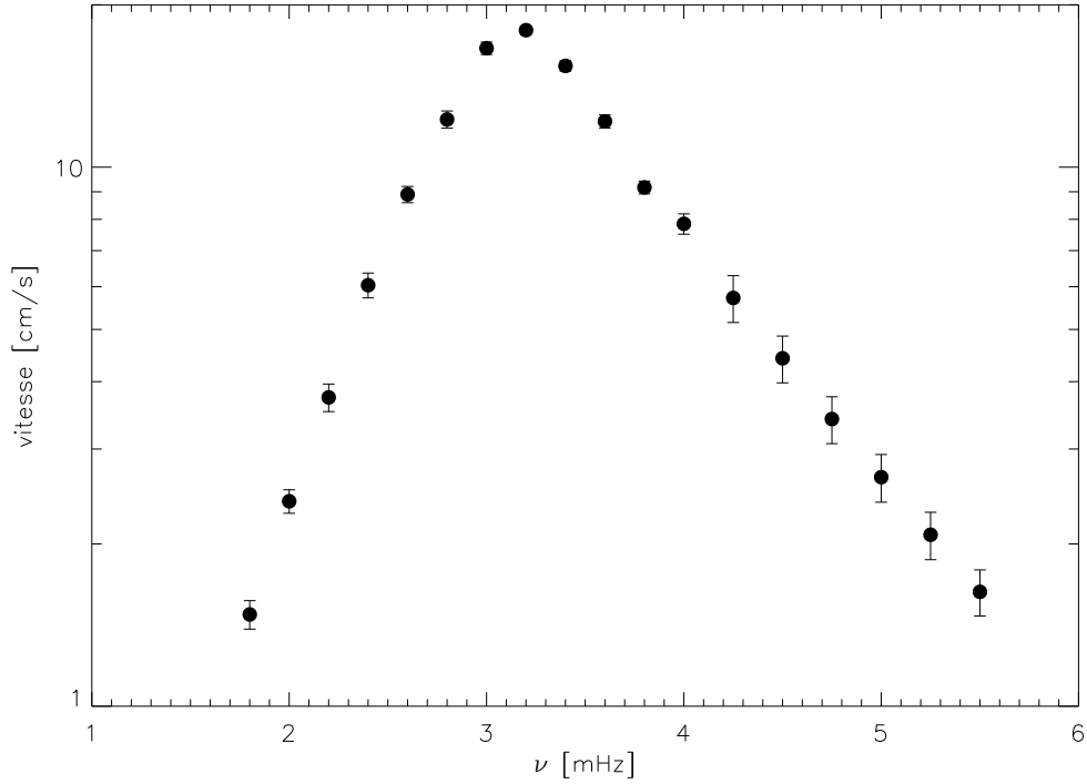
FIG. 2.4 – Racine carré de la vitesse quadratique moyenne des oscillations solaires mesurée par Libbrecht par ajustement du profil Lorentzien sur le spectre de puissance observé. Les points de mesures sont accompagnés de leur barre d'erreur respective.
