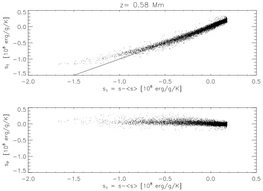
FIG. 5.11 – Tracés effectués à la profondeur z = 0.58 Mm avec les mêmes considérations que celles de la figure 5.10.
