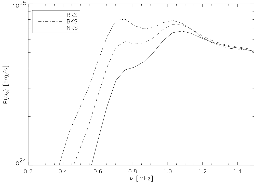
FIG. 6.1 – Spectre de puissance P(\omega_0) calculé pour le modèle de Procyon en considérant différents spectres de turbulence. Le modèle de Procyon a été obtenu à l'aide du code CESAM tandis que les modes propres ont été obtenus à l'aide au code adiabatique FILOU.
