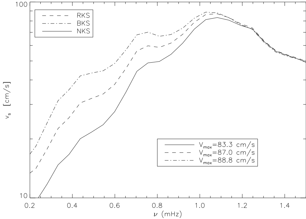
FIG. 6.10 – Idem figure 6.9, les estimations concernent ici le modèle d'équilibre de Procyon basé sur la MLT standard.
