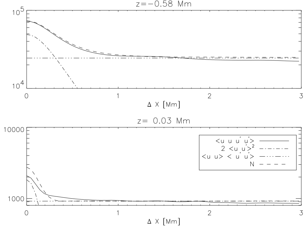
FIG. 5.5 – Tracés des quantités \langle uu'u'u' \rangle , 2 \langle u'u' \rangle^2 , \langle u'u' \rangle \langle u'u' \rangle et N(\Delta x) en fonction de \Delta x (voir texte pour la signification de ces quantités). Le panneau supérieur concerne la couche supérieure de la simulation (de profondeur z = -0.58 Mm) tandis que le panneau inférieur concerne la profondeur z = 0.03 Mm correspondant à la couche où l'écart-type de la vitesse radiale est maximale. Le terme cumulant C(\Delta x) correspond à l'écart entre les courbes \langle uu'u'u' \rangle (ligne continue) et N (ligne discontinue).
