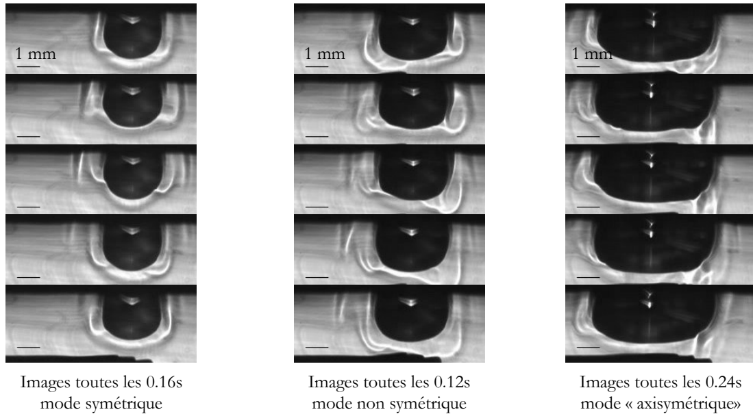
Figure V-10: Différents modes oscillatoires lors de la croissance de la bulle de vapeur, T_1=39,3^\circ\text{C} , P_c=1450\text{ mW} . [BARTHES-2005-a]
