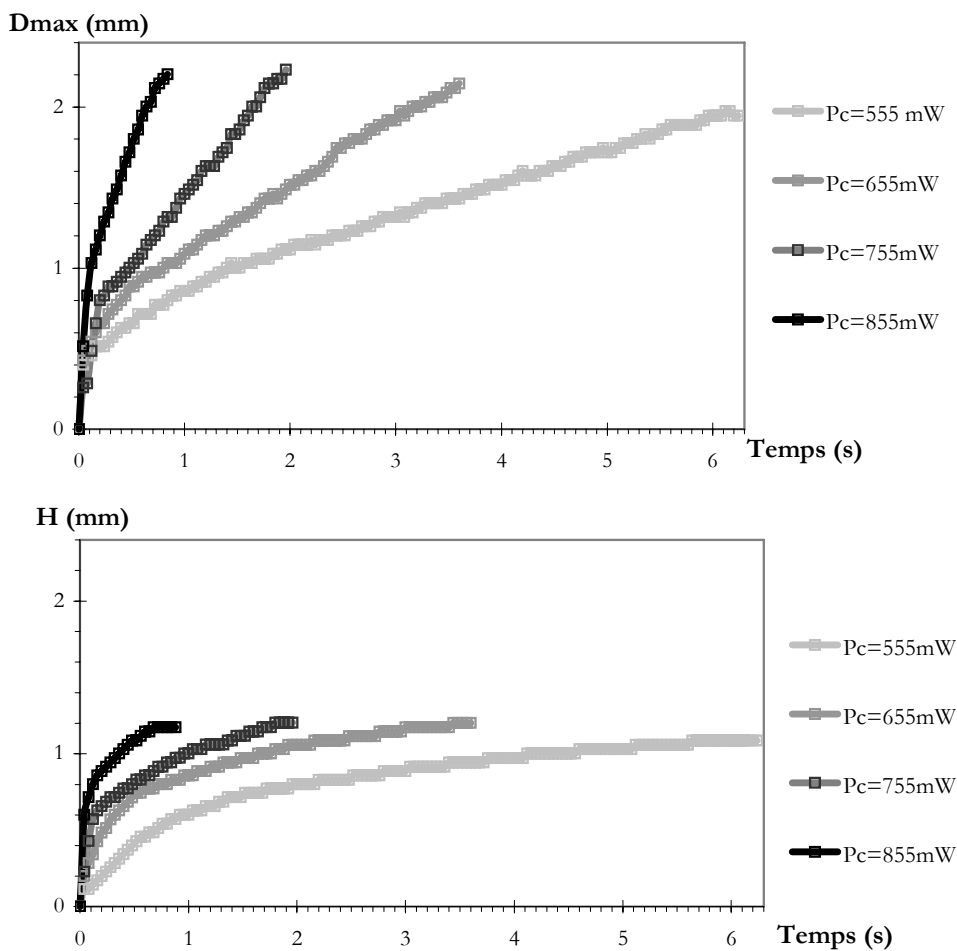
Figure IV-7 : Influence de la puissance de chauffe sur l'évolution temporelle du diamètre maximal et de la hauteur, \Delta T_{sub} = 8,4 \pm 0,3^\circ\text{C} , \alpha=1,4^\circ .
