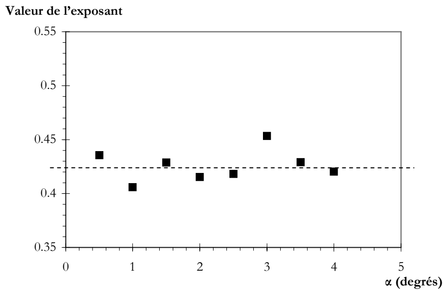
Figure IV-29 : Exposant en fonction de l'angle d'inclinaison. : Variation de l'exposant en fonction de l'inclinaison, \Delta T_{\text{sub}}=8,3\pm 0,2^{\circ}\text{C} , P_c= 700 \text{ mW} .
