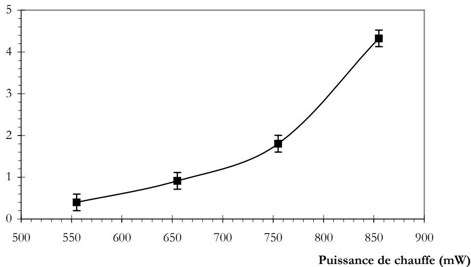
Figure IV-36 : Flux d'évaporation moyen en fonction de la puissance de chauffe, \Delta T_{\text{sub}}=8,3\pm 0,3^{\circ}\text{C} , \alpha=1,4^{\circ} .
