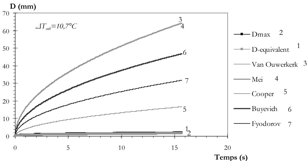
Figure IV-24 : Comparaison de modèles de la littérature et des résultats expérimentaux, (diamètre maximal et diamètre équivalent), \Delta T_{sub} = 10,7^\circ C , P_c = 555 \text{ mW} , \alpha = 1,8^\circ .
