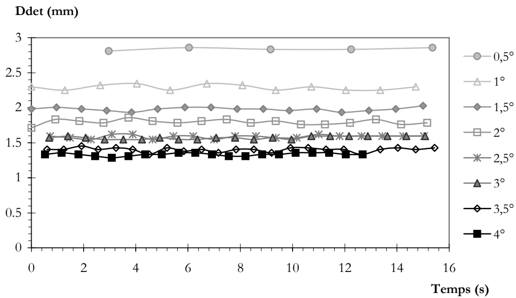
Figure IV-11 : Diamètre de détachement en fonction du temps pour \Delta T_{sub} = 10 \pm 0,3^\circ C , P_c = 900 mW.
