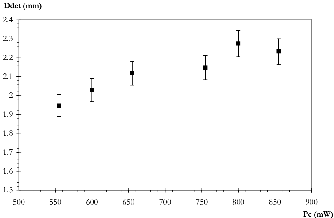
Figure IV-17 : Influence de la puissance de chauffe sur le diamètre de détachement, \alpha=1^\circ , \Delta T_{\text{sub}}=8,6\pm 0,3^\circ\text{C} .
