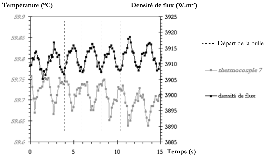
Figure IV-50 : Influence de la bulle sur la température du thermocouple situé en périphérie de l'élément et sur la densité de flux, \Delta T_{\text{sub}}=8,8\pm 0,1^{\circ}\text{C} , P_c=734\text{ mW} .
