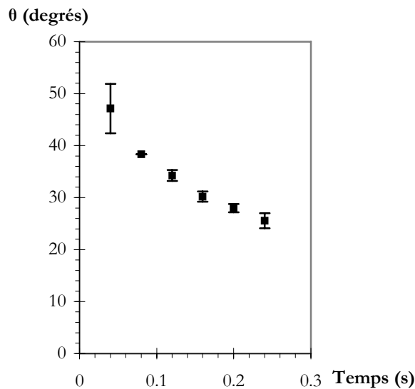
Figure IV-44 : Évolution temporelle de la valeur de l'angle de contact calculé pour la bulle accrochée en totalité sur le site, jusqu'à son « décrochement ». \Delta T_{\text{sub}}=9,9\pm 0,1^{\circ}\text{C} , P_c=700\text{ mW} , \alpha=0,5^{\circ} .
