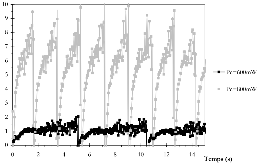
Figure IV-33 : Flux d'évaporation, \Delta T_{\text{sub}}=8,3 \pm 0,2^\circ\text{C} , \alpha=0,5^\circ .
