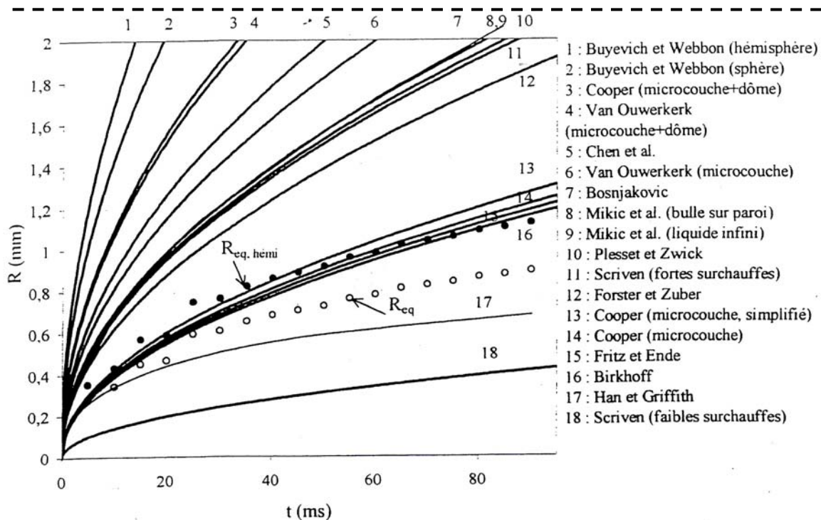
Modèles de croissance R(t) et croissance expérimentale ( P = 1 \text{ bar} , Q_p = 1,12 \text{ W} , \Delta T_{\text{sat}} = 8,1 \text{ K} )
