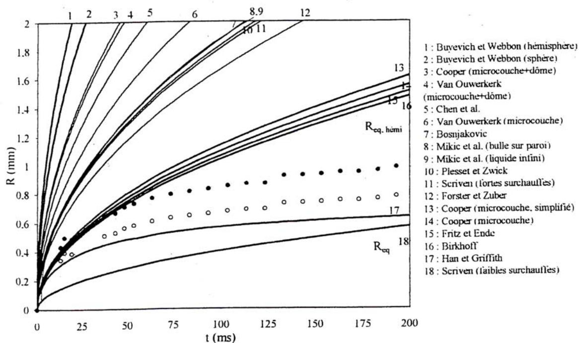
Modèles de croissance R(t) et croissance expérimentale ( P = 1 \text{ bar} , Q_p = 1,12 \text{ W} , \Delta T_{\text{sat}} = 8,1 \text{ K} )
