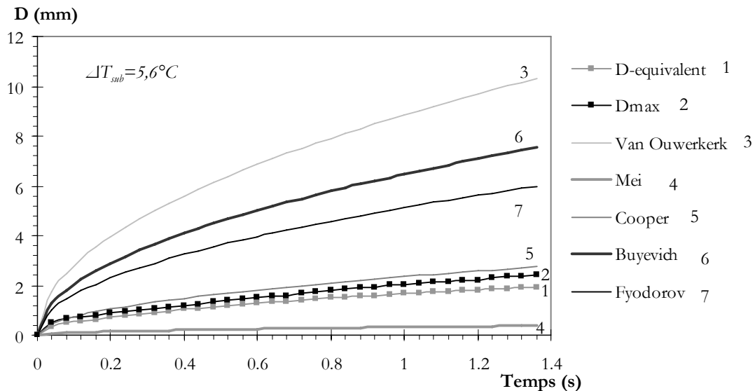
Figure IV-23 : Comparaison de modèles de la littérature et des résultats expérimentaux (diamètre maximal et diamètre équivalent), \Delta T_{sub} = 5,6^\circ C , P_c = 555 \text{ mW} , \alpha = 1,8^\circ .
