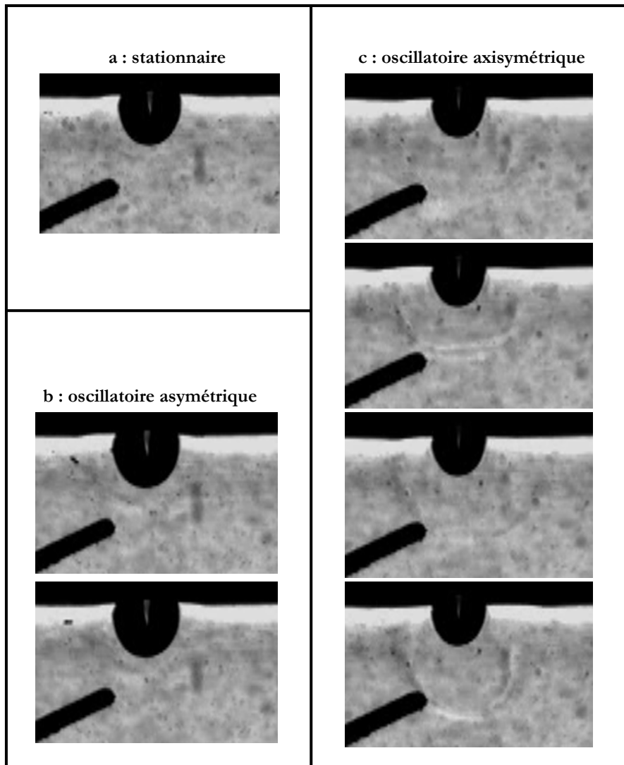
Figure V-13: Visualisation des régimes d'écoulement autour de la bulle de vapeur (FC-72) en croissance, puis en recondensation. T_1=33,5\pm 0,5^\circ\text{C} , P_c=1061\text{ mW} .
