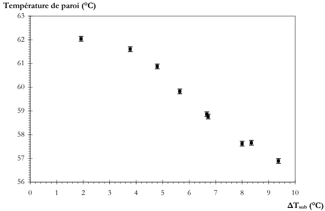
Figure IV-51: Évolution de la température moyenne de paroi en fonction du niveau de sous-refroidissement, P_c=555 mW, \alpha=1,8^\circ .
