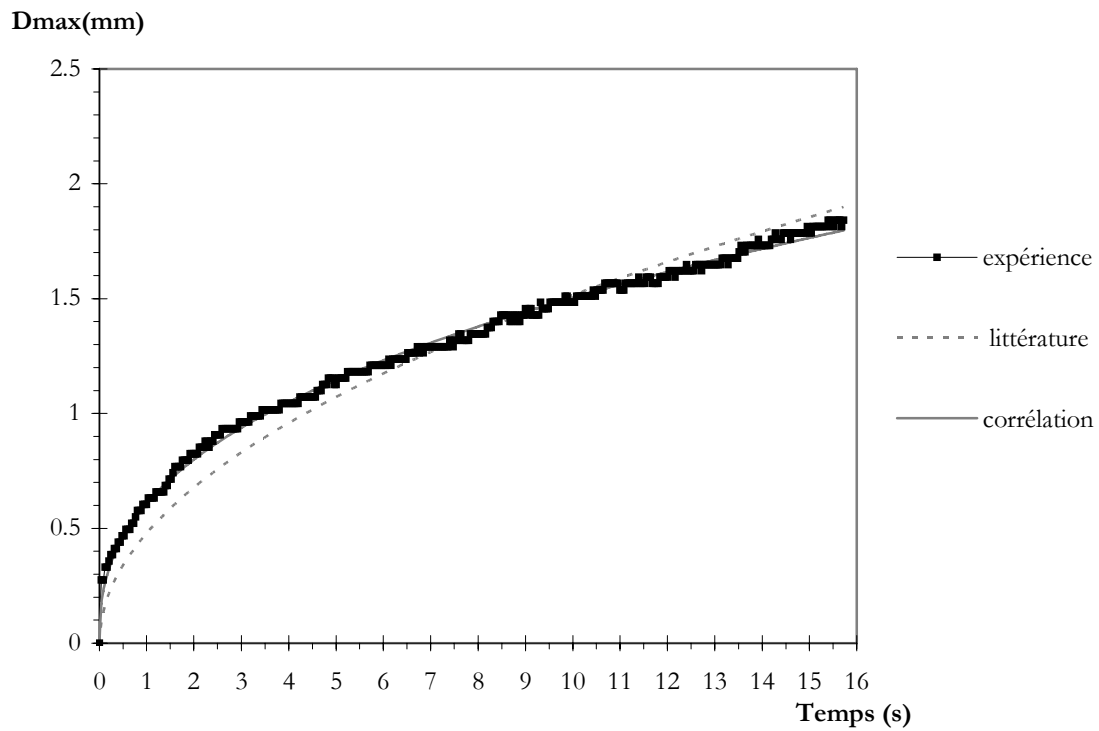
Figure IV-26 : Comparaison expérience et littérature, \Delta T_{\text{sub}}=10,7\pm 0,1^{\circ}\text{C} , \alpha=1,8^{\circ} , P_c=555\text{ mW} .
