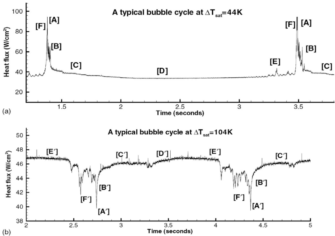
Figure II-7 : Cycle d'ébullition d'une bulle isolée pour deux surchauffes : 44 et 104°C, FC-72 sous-refroidi, \Delta T_{sub} = 31,5^\circ C , [CHEN-2004].
