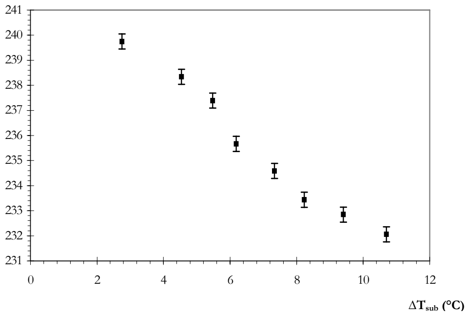
Figure IV-55 : Évolution du flux total moyen (mesuré par le fluxmètre thermique) en fonction du niveau de sous-refroidissement, P_c = 555 mW, \alpha = 1,8^\circ .
