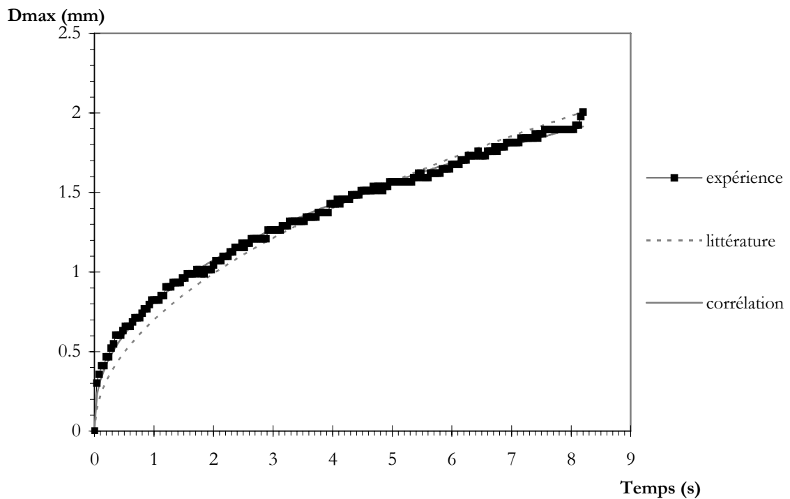
Figure IV-27 : Comparaison expérience et littérature, \Delta T_{\text{sub}}=8,2\pm 0,1^{\circ}\text{C} , \alpha=1,8^{\circ} , P_c=555\text{ mW} .
