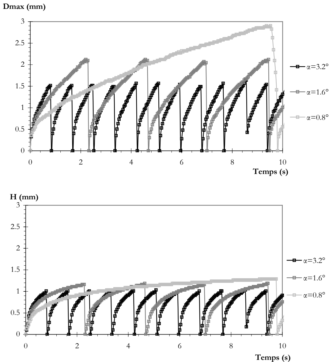
Figure IV-9 : Diamètre maximal et hauteur de la bulle en fonction du temps : influence de l'inclinaison de la surface de nucléation sur l'évolution temporelle du diamètre maximal, \Delta T_{sub} = 7,2 \pm 0,2^\circ C , P_c = 585 mW.
