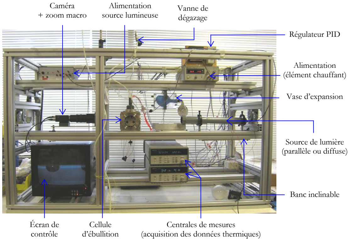
Figure III-4: Photo du montage expérimental
