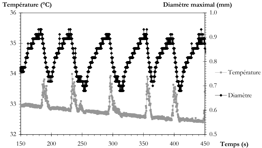
Figure V-14: Diamètre maximal et température mesurée sous la bulle de vapeur en fonction du temps : mise en évidence de l'influence des « bouffées » de convection sur les mesures de température. T_1=33,5 \pm 0,5^\circ\text{C} , P_c=1061 \text{ mW} .
