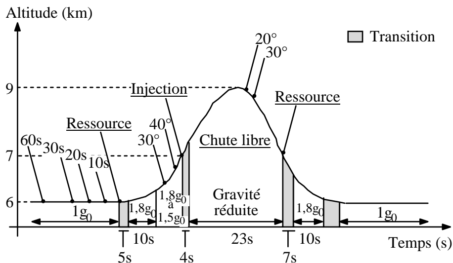
Figure III-2 : Description de la manœuvre parabolique [REYNARD-2001-a].
