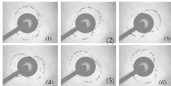
Figure V-5 : Images du mode oscillatoire symétrique à deux extrema dans un plan horizontal par ensencement. Rayon de la bulle d'air : 3,1 mm, gradient de température : 2,1 \text{ }^\circ\text{C}/\text{mm} . [REYNARD-2005].
