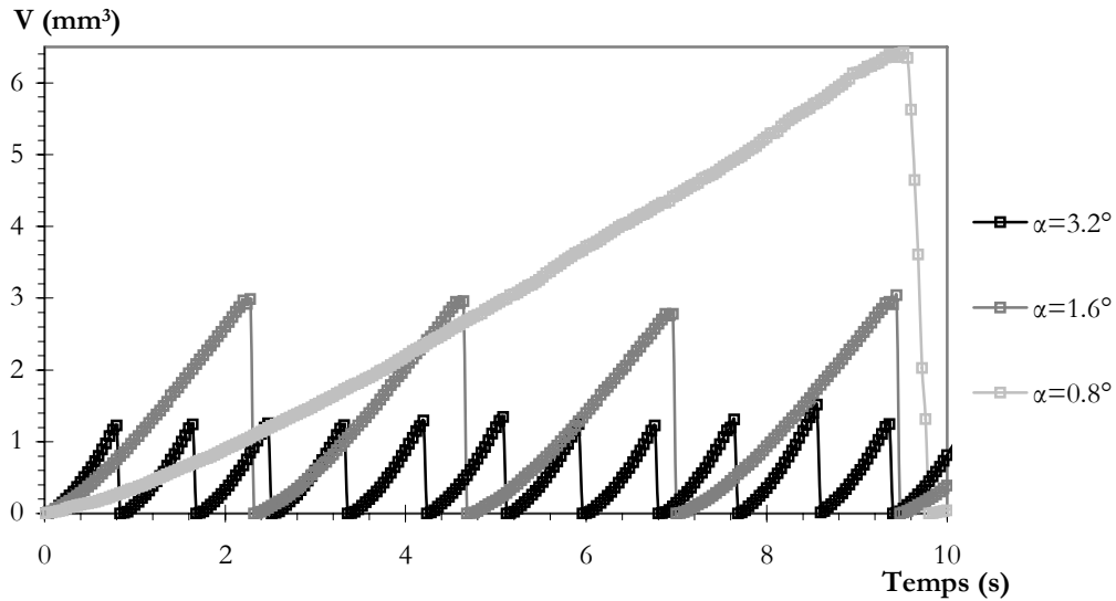
Figure IV-10 : Influence de l'angle d'inclinaison de la surface de nucléation sur l'évolution temporelle du volume, \Delta T_{sub} = 7,2 \pm 0,2^\circ C , P_c = 585 mW.
