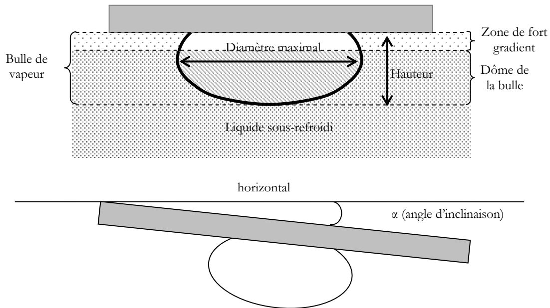
Figure IV-1 : Dénomination des parties de la bulle
