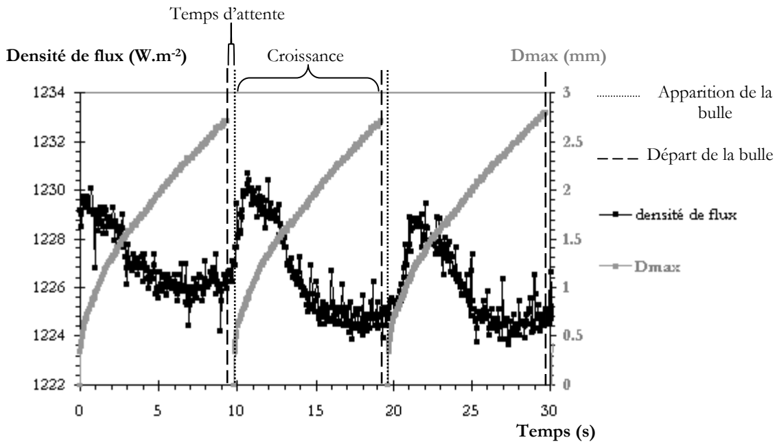
Figure IV-47 : Synchronisation des signaux optiques et thermiques : phases de croissance de la bulle de vapeur. \Delta T_{sub}=10,0 \pm 0,1^{\circ}C , P_c=700 mW, \alpha=0,5^{\circ} .
