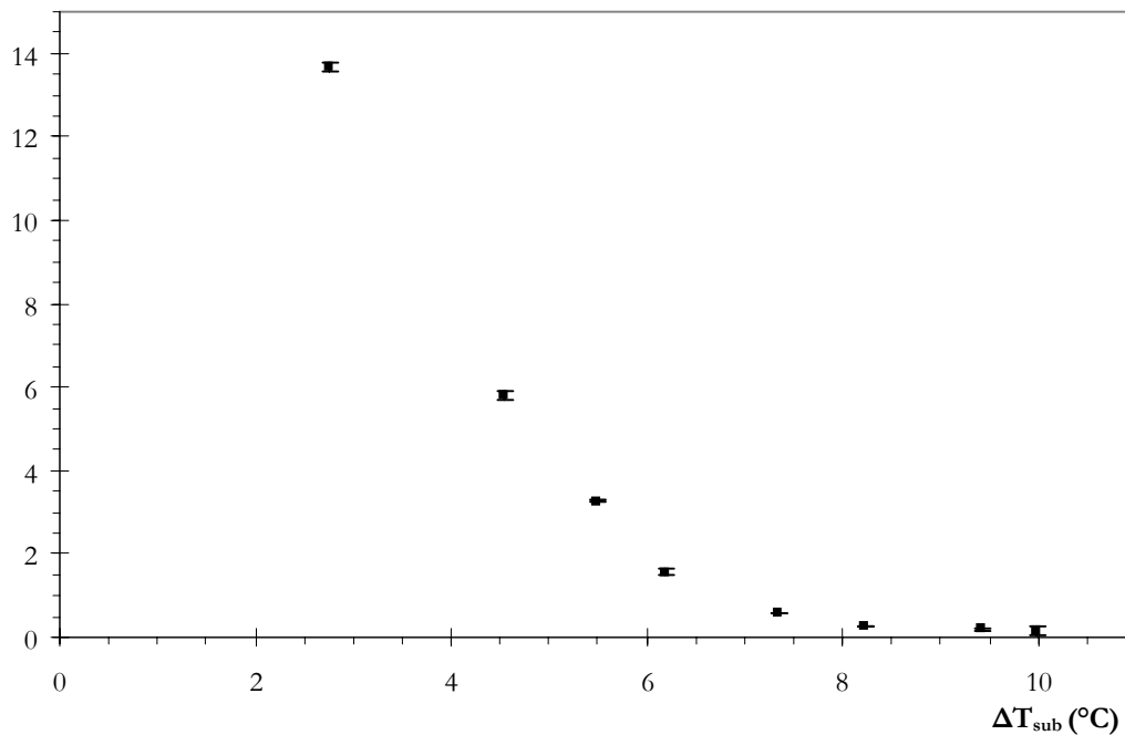
Figure IV-35 : Flux d'évaporation moyen en fonction du sous-refroidissement, Pc=555 mW, α=1,8°. [BARTHES-2005-b].
