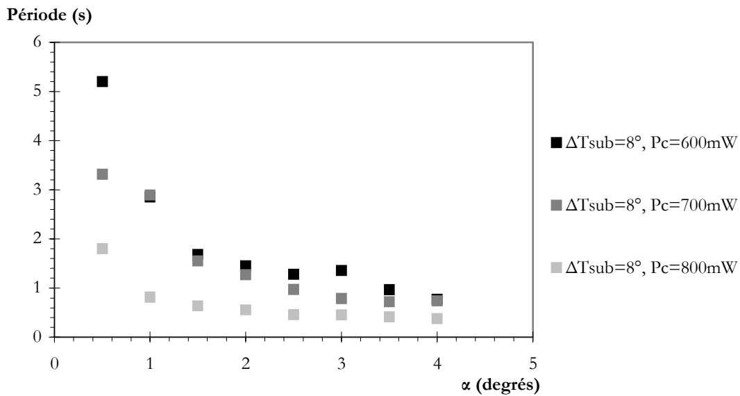
Figure IV-22 : Influence de la puissance de chauffe et de l'inclinaison sur la période d'émission de bulles, \Delta T_{sub}=8,6\pm 0,3^{\circ}C .
