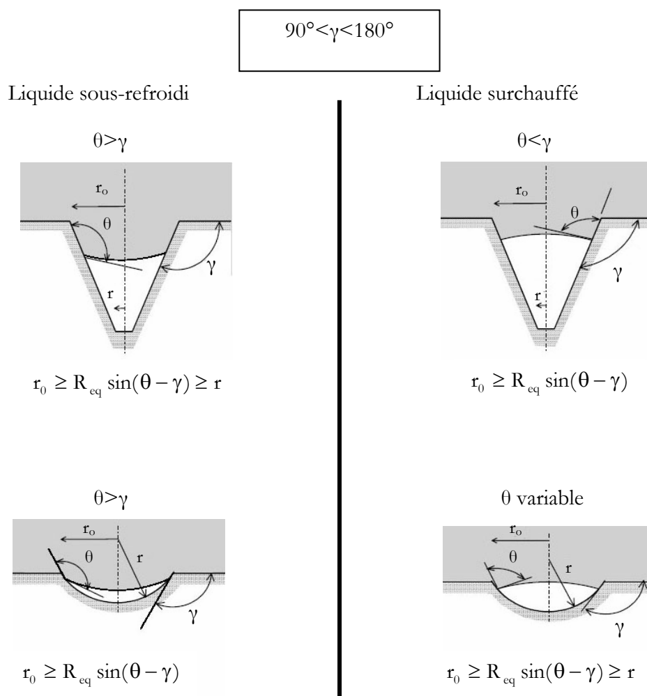
Figure I-11 : Conditions d'existence de l'embryon de vapeur à l'équilibre avec la phase liquide sous-refroidi ou surchauffé- Cavités coniques et sphériques ouvertes, [STUTZ-2003].
