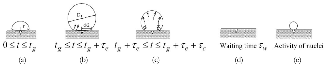
Figure I-14 : Cycle d'ébullition [ZHAO-2002].
