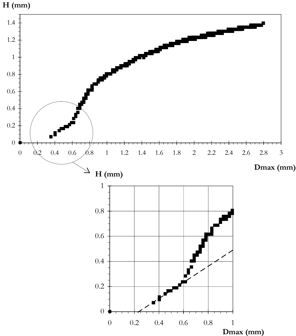
Figure IV-39 : Hauteur en fonction du diamètre maximal, \Delta T_{sub}=9,9\pm 0,1^\circ\text{C} , P_c=700 mW, \alpha=0,5^\circ .
