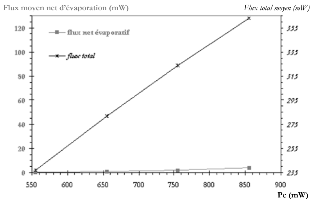
Figure IV-66 : Influence de la puissance de chauffe sur les flux moyens (d'évaporation et total), \Delta V=8,3\pm 0,3^{\circ}C , \alpha=1,4^{\circ} .
