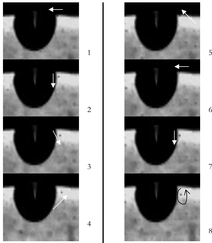
Figure V-9 : Mise en évidence du régime stationnaire par ensemencement. Pas de temps : 0,04s. T_1=33,5\pm 0,5^\circ\text{C} , P_c=1061\text{ mW} , diamètre de la bulle : environ 0,8 mm.
