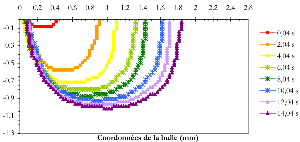
Figure IV-3 : Contour de la bulle, \Delta T_{\text{sub}}=10,7\pm 0,1^\circ\text{C} , P_c=555 mW, \alpha=1,8^\circ .
