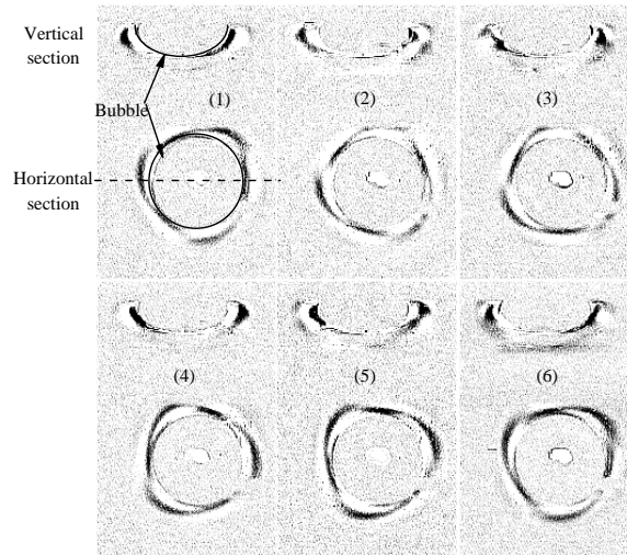
Figure V-6 : Image du mode oscillatoire tridimensionnel asymétrique à trois extrema dans les plans horizontal et vertical, par ombroscopie. Rayon de la bulle d'air : 4,1 mm, gradient de température : 3,3 °C/mm). [REYNARD-2005].
