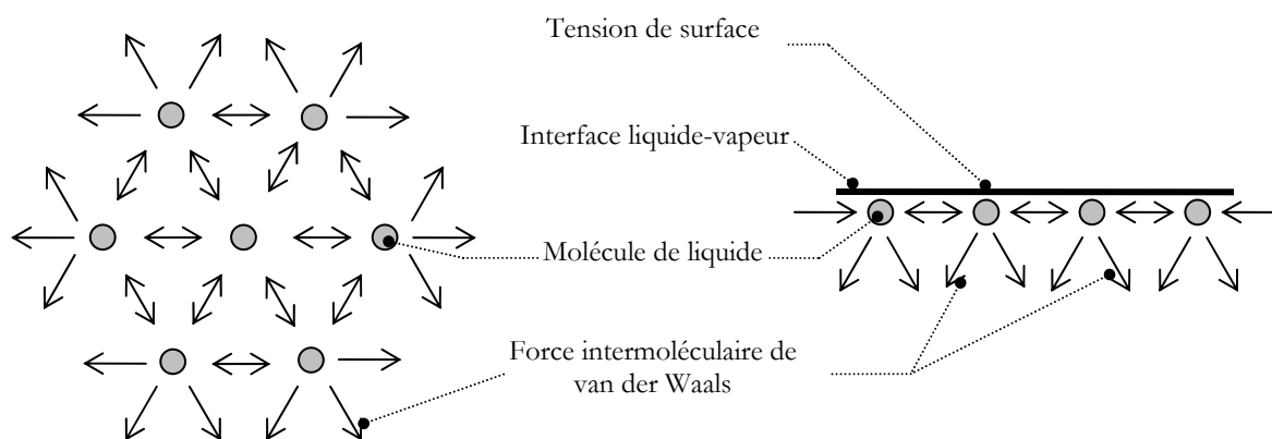
Figure I-3 : Molécules au sein et à la surface d'un liquide. Notion de tension de surface.
