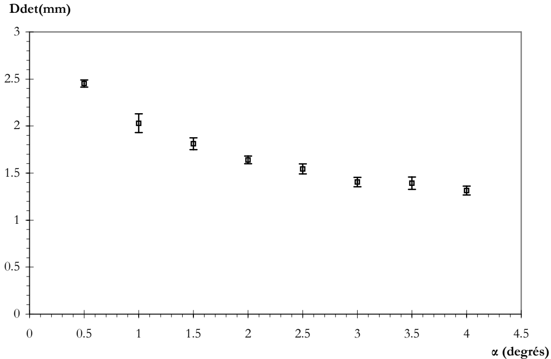
Figure IV-18 : Influence de l'inclinaison sur le diamètre de détachement. \Delta T_{sub}=8,3\pm 0,2^{\circ}C , P_c= 600 mW.
