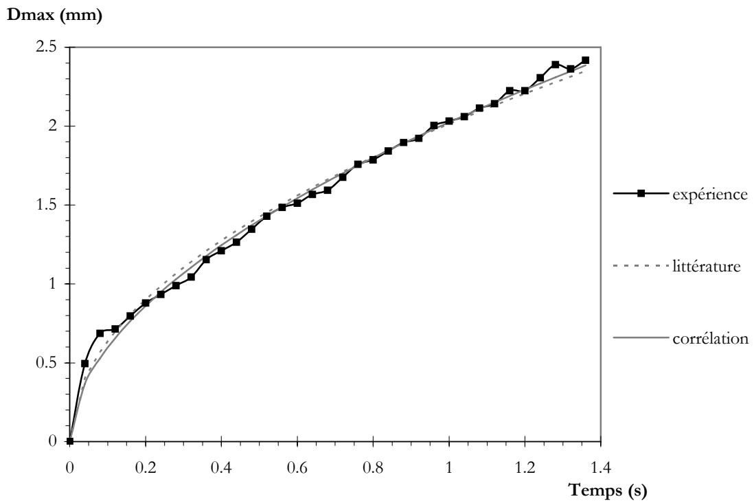
Figure IV-28 : Comparaison expérience et littérature, \Delta T_{sub}=5,6\pm 0,1^{\circ}C , \alpha=1,8^{\circ} , P_c=555 mW.
