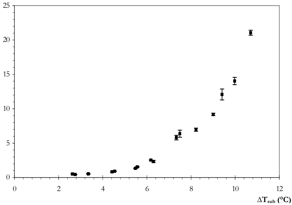
Figure IV-54 : Période d'émission de bulle en fonction du niveau de sous-refroidissement, déterminée par traitement du signal délivré par le fluxmètre (transformée de Fourier), P_c = 555 mW, \alpha = 1,8^\circ . [BARTHES-2005-b]
