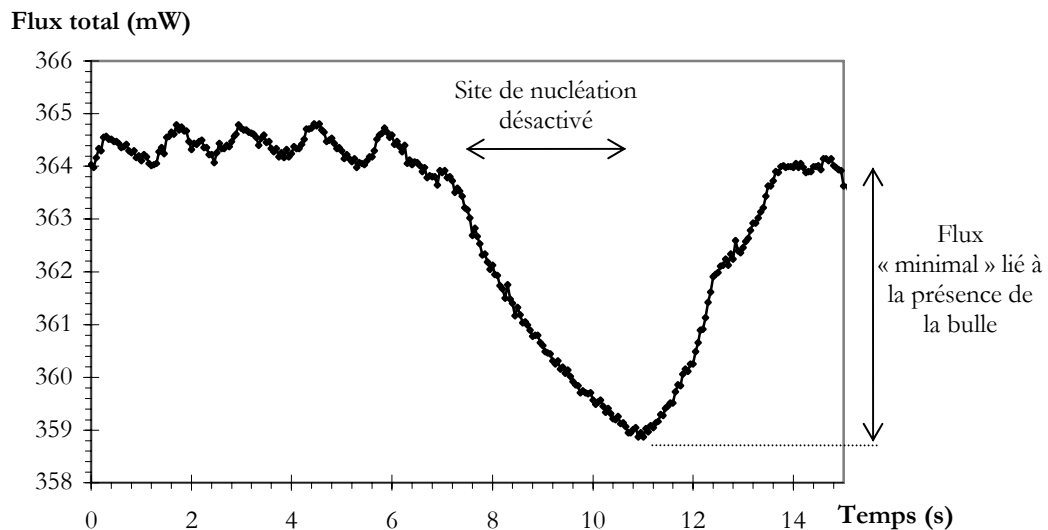
Figure IV-63 : Influence de la bulle sur le signal délivré par le fluxmètre thermique. \Delta T_{\text{sub}}= 8,6\pm 0,1^{\circ}\text{C} , P_c=855 mW ( T_p=61,7^{\circ}\text{C} ), \alpha=1,4^{\circ} .
