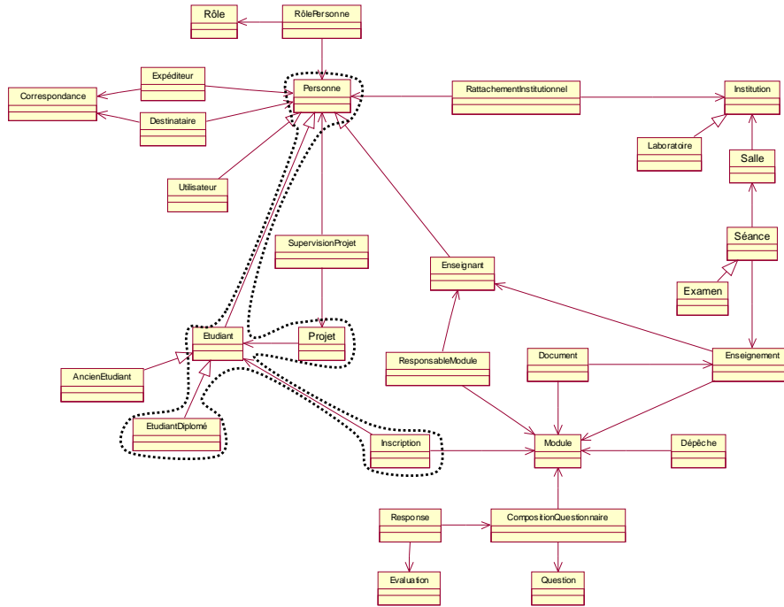
Figure 14 : D_{M@TIS} , le diagramme de classes de M@TIS
