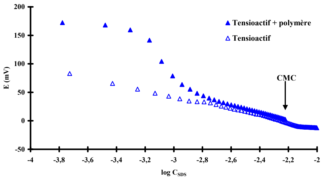
Figure I-4 : E_{em} en fonction du logarithme de la concentration en tensioactif : courbe typique de calibration d'un tensioactif pur (triangles ouverts). Courbe typique pour un mélange tensioactif – polymère.
