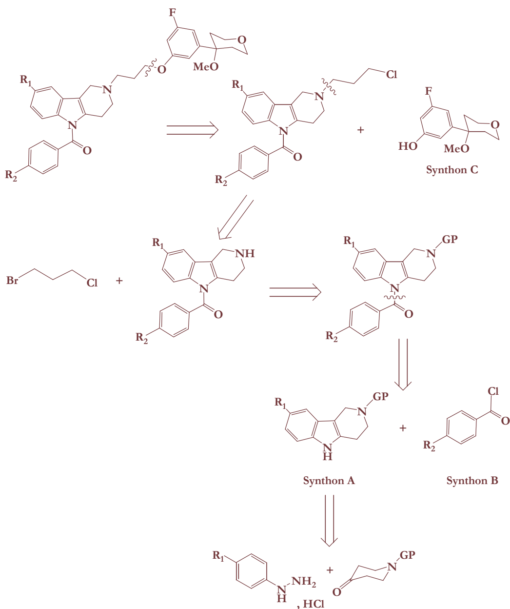
Schéma 7: Schéma de rétrosynthèse.
