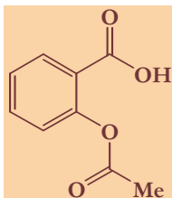
Figure 18 : Structure de l'aspirine.
