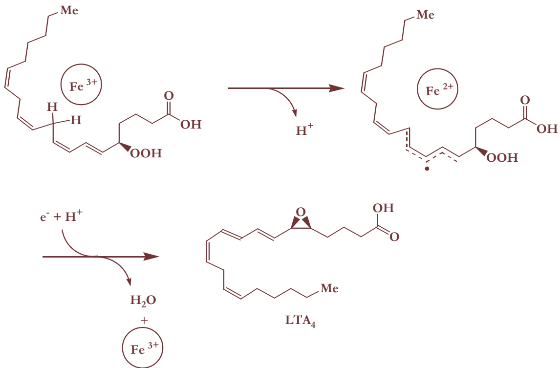
Figure 6 : Mécanisme de la 5-lipoxygénase. Formation du LTA 4 .
