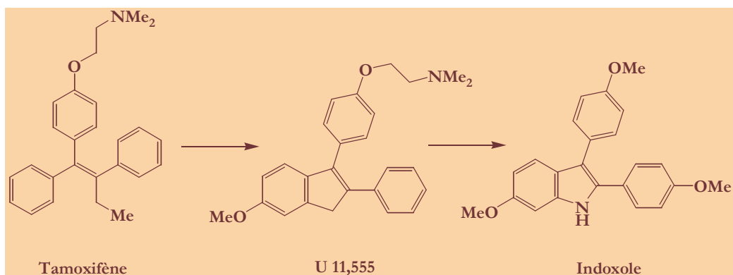
Figure 17: Evolution vers les premiers anti-inflammatoires.
