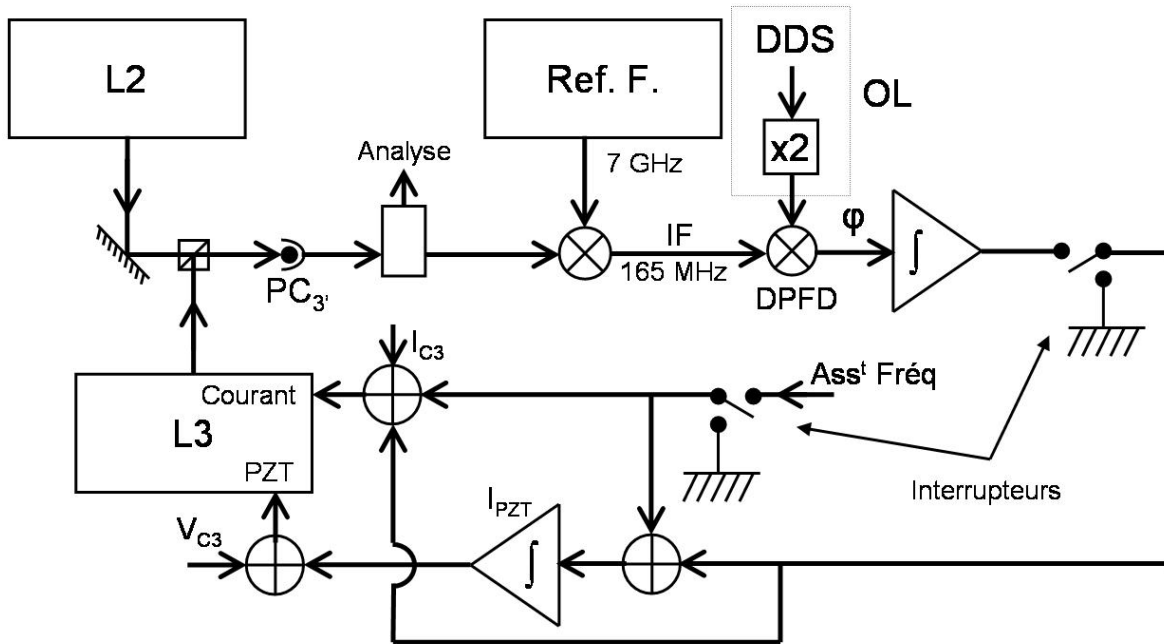
FIG. 4.13 – Boucle d’asservissement de phase de L3. Le battement entre L2 et L3 est mesuré sur un dernier photoconducteur rapide PC_{3'} et comparé à la même référence de fréquence à 7 GHz. La fréquence intermédiaire est comparée à un oscillateur local (OL) constitué d’un synthétiseur digital de fréquence (DDS) doublé en fréquence. La comparaison est effectuée dans un détecteur phase/fréquence digital (DPFD). Le signal d’erreur de phase est intégré puis sommé au courant d’alimentation du laser L3. Il est également sommé au signal de contrôle de la cale piézo-électrique de l’asservissement de fréquence avant la dernière intégration.
