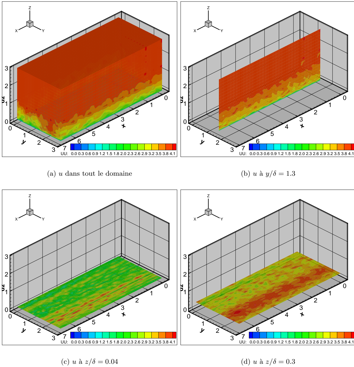
FIG. 6.1 – Visualisation de la composante longitudinale de la vitesse instantanée, u , sur trois plans correspondant à y/\delta = 1.3 , z/\delta = 0.04 et z/\delta = 0.3 .
