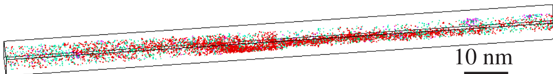
FIG. 5.8 – Analyse d'un objet riche en cuivre, probablement un joint de grain, dans un alliage prérevenu. Cet objet n'est pas enrichi en magnésium.
