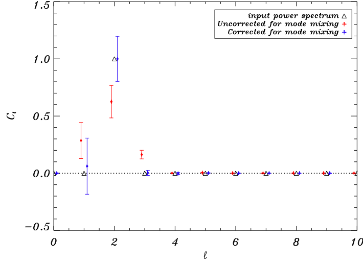
FIG. 3.1 : Démonstration de principe de la méthode d'estimation du spectre de puissance (Monte-Carlo). On injecte des événements dont la distribution sur le ciel est un pur quadripôle d'axes principaux aléatoires. En rouge sont représentés les pseudo- C_\ell reconstruits, et en bleu les C_\ell estimés après déconvolution par les M_{\ell\ell'} , avec leurs barres d'erreur analytiques.
