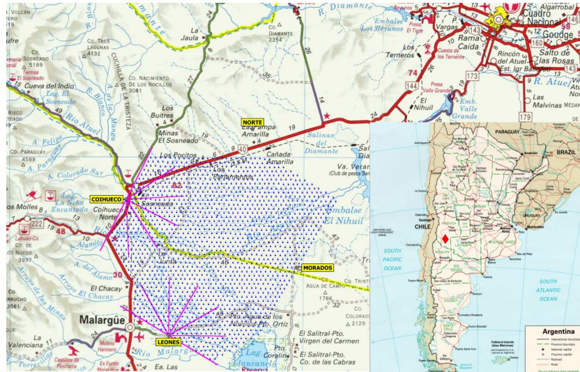
FIG. 1.1 : Site Sud de l'Observatoire, au pied des Andes. La ville au Nord-est est San Raphaël. Le centre d'acquisition des données se trouve à Malargüe. Chaque point symbolise une des 1600 cuvas prévues, et les quatre sites de fluorescence sont aussi représentés.
