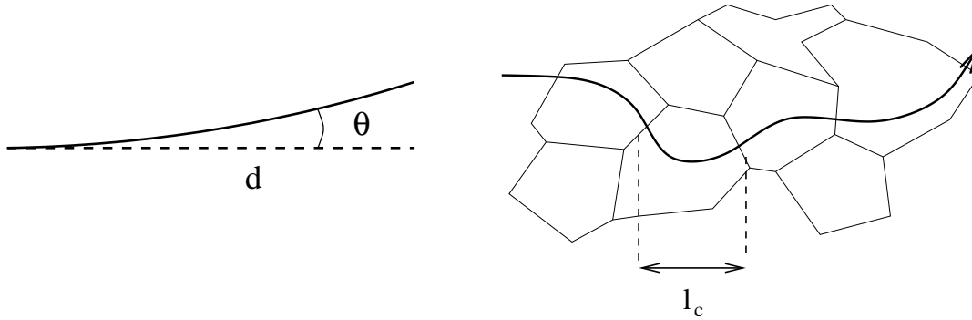
FIG. 5.6 : Gauche : géométrie d'une déflexion faible dans un champ magnétique uniforme. Droite : géométrie d'une déflexion faible dans un champ magnétique de longueur de cohérence l_c . Les « cellules » représentent des domaines de cohérence du champ magnétique.
