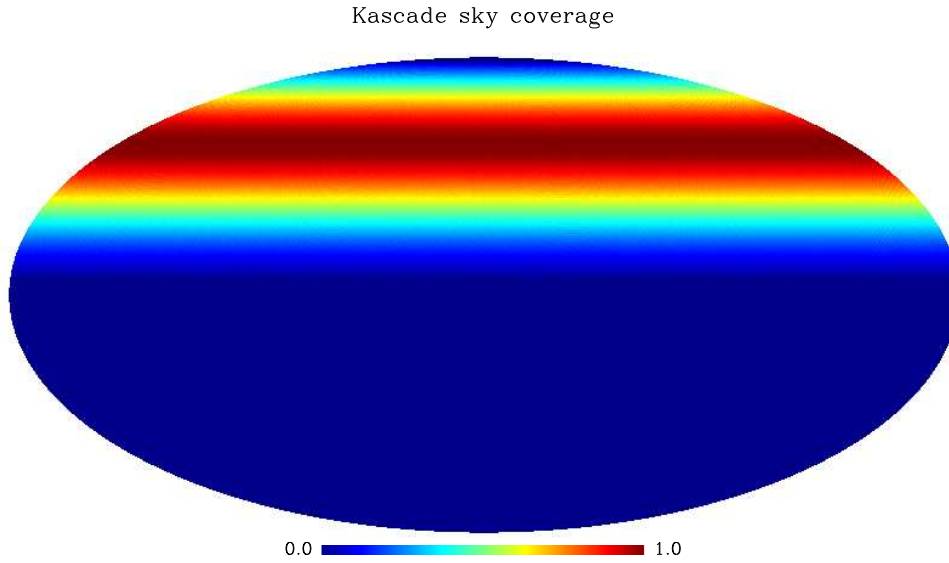
FIG. 3.3 : Couverture du ciel de l'expérience Cascade. À cause de la trop faible longueur d'atténuation des gerbes aux énergies du genou, la couverture est limitée à une portion du ciel bien plus faible qu'Auger.
