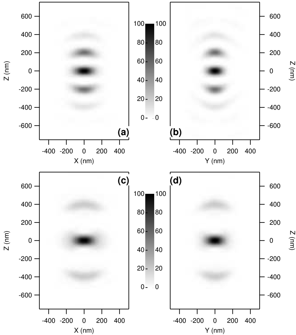
FIG. 5.34 – Cartes d'efficacité de détection dans le plan (XOZ) pour (a) et (c) et dans le plan (YOZ) pour (b) et (d) , d'un microscope d'ouverture numérique NA=1.3 dans l'huile et de grossissement m=40 . L'excitation est à 1 photon ( \lambda=488nm ) pour (a) et (b) et à 2 photons ( \lambda = 2 \times 488nm ) pour (c) et (d) . Le Laser est gaussien ( \beta=0.1 ) polarisé rectilignement selon X . La fluorescence est considérée comme monochromatique ( \lambda=525nm ). Le trou confocal a un diamètre de 20 microns.
