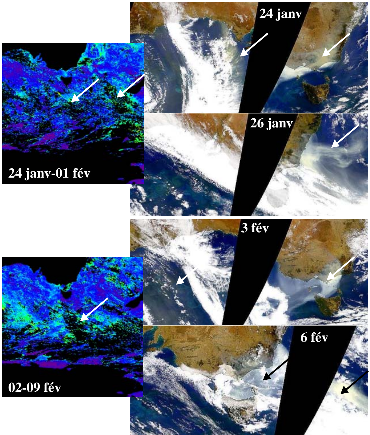
Figure C.1 Cartes hebdomadaires de la distribution d'épaisseur optique d'aérosols (AOT) et de couleur vraie issues de SeaWiFS pour les semaines du 24 janvier au 1 février et du 2 au 9 février 2003.
