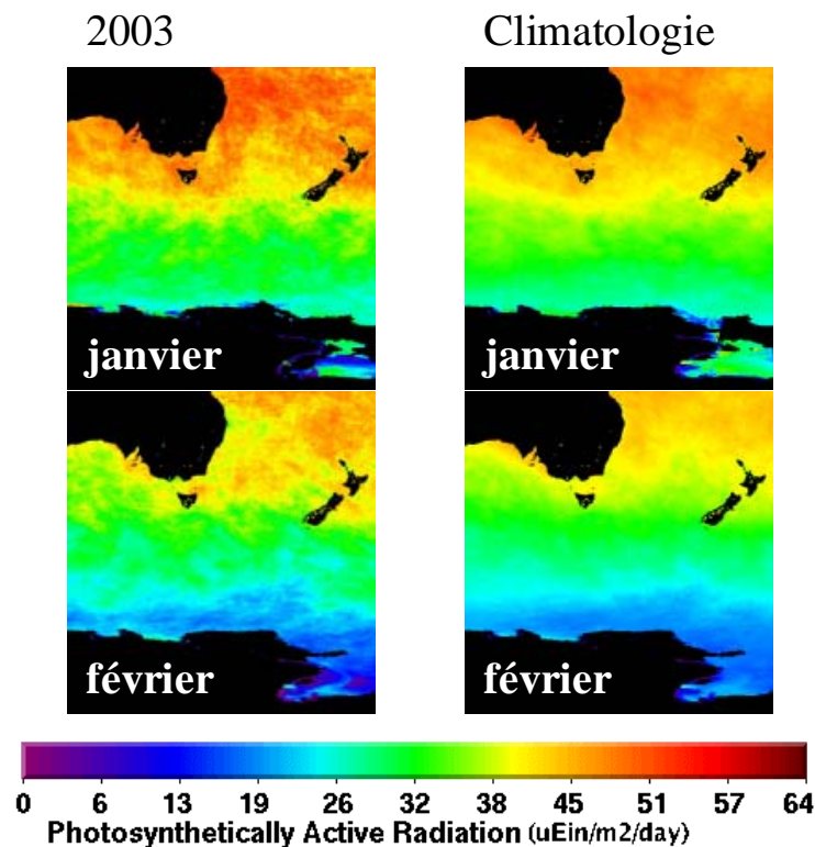
Figure B.3 Distribution de PAR moyennes mensuelles issues de SeaWiFS de janvier et février 2003 à gauche et climatologique à droite.
