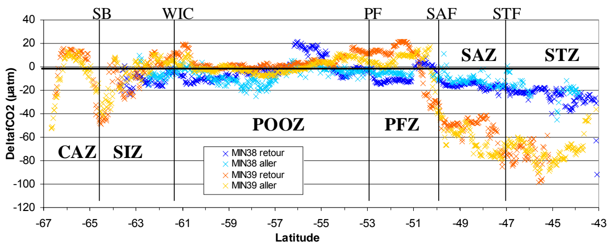
Figure A.6 Distribution de \Delta fCO_2 en fonction de la latitude pour les campagnes MIN38 et MIN39.
