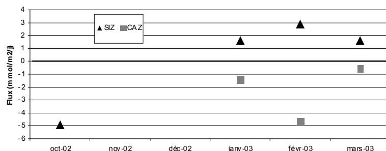
Figure C.1 Variations saisonnières du flux de CO 2 à l'interface air-mer dans la SIZ et la CAZ. Les flux sont calculés à partir des données des campagnes MINERVE R0, R2 et R4 et OISO10.
