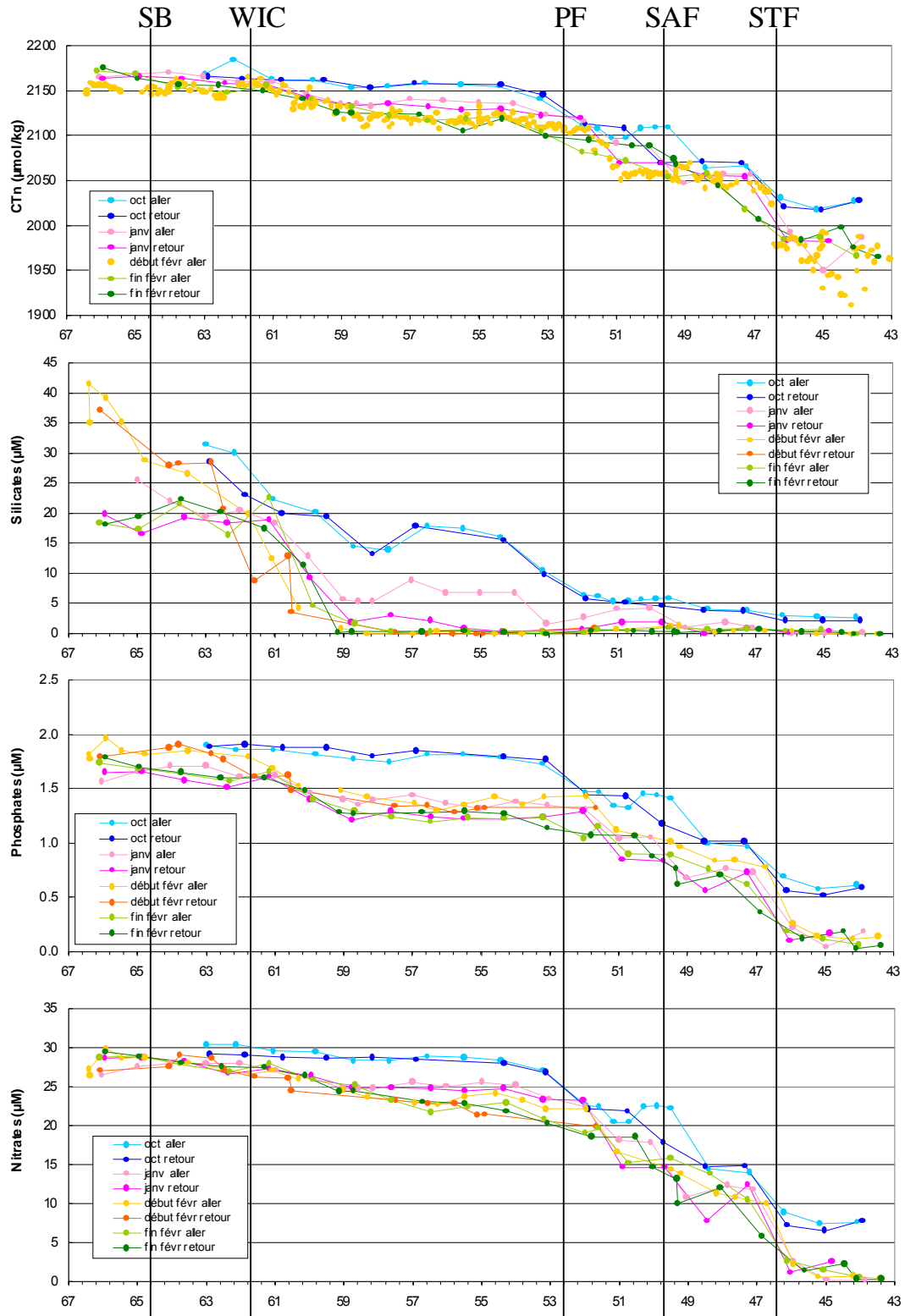
Figure B.3 Distribution des paramètres biogéochimiques (sels nutritifs et CTn) des campagnes MINERVE R0, R2 et R4 et OISO10 en fonction de la latitude.
