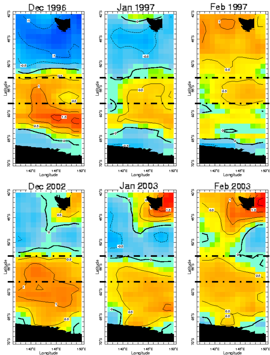
Figure A.1 Cartes représentant les anomalies de SST dans l'océan Austral au sud de la Tasmanie pour les mois de décembre, janvier et février de 1996/97 et 2002/03.
