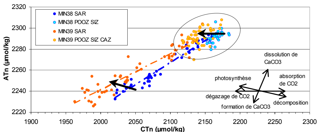
Figure A.5 ATn en fonction de CTn pour les campagnes MIN38 et MIN39.
