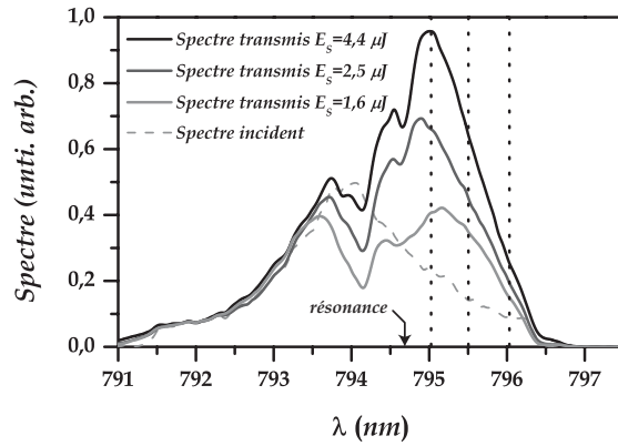
FIG. IV.20 – Spectre de l'impulsion faible transmise pour E_S=1,6 \mu\text{J} , 2,5 \mu\text{J} et 4,4 \mu\text{J} ( \lambda_S = 799,3 \text{ nm} , \Delta\lambda_S = 1,1 \text{ nm} FWHM). Les pointillés matérialisent les longueurs d'onde \lambda = 795,02 \text{ nm} , 795,5 \text{ nm} et 796,03 \text{ nm} .
