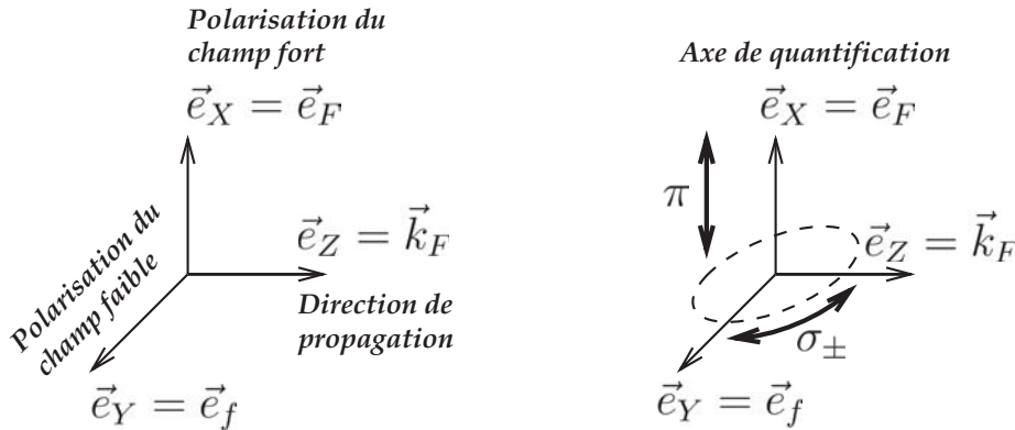
FIG. V.1 – Définition des axes de polarisation et de quantification : Les ondes gauche et droites sont définies par rapport à l'axe de quantification \pi selon \vec{e}_X . Elles ne sont pas identiques aux ondes gauche et droite définies par rapport au vecteur d'onde \vec{k}_F = \vec{e}_Z qui définit la direction de propagation.
