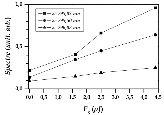
FIG. IV.21 – Spectre de l'impulsion faible transmise en fonction de l'énergie E_S du champ fort pour \lambda = 795,02 \text{ nm} , 795,5 \text{ nm} et 796,03 \text{ nm} avec E_S=0, 1,6 \mu\text{J} , 2,5 \mu\text{J} et 4,4 \mu\text{J} ( \lambda_S = 799,3 \text{ nm} , \Delta\lambda_S = 1,1 \text{ nm} FWHM).
