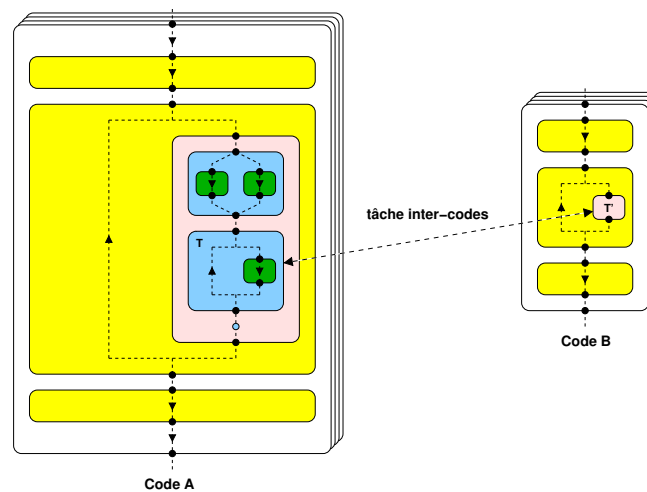
FIG. 8.1 – Définition d’une tâche inter-codes entre deux MHTs couplés.
