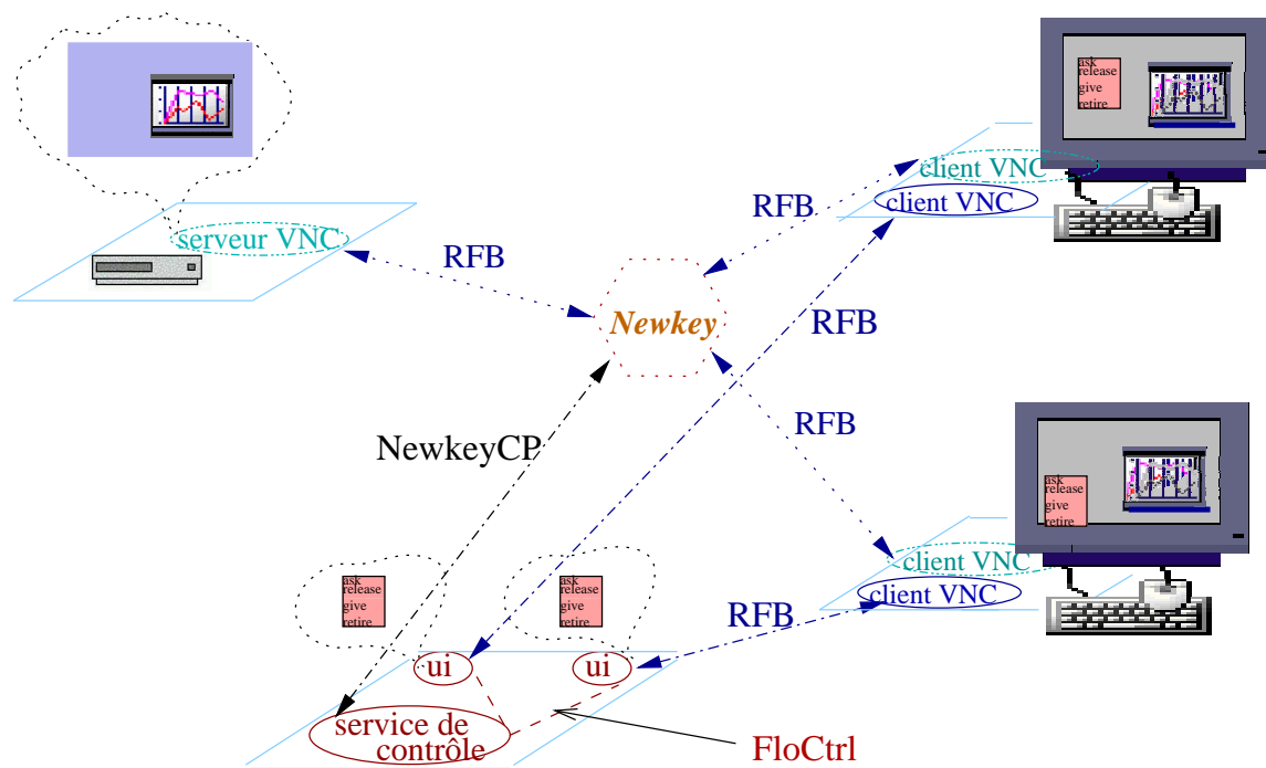
FIG. 5.5 – L'architecture du système NC enrichi avec le contrôle de droit d'entrée floor .
