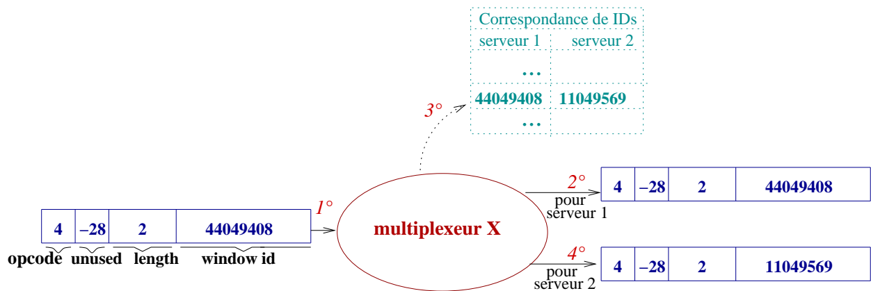
FIG. 3.5 – Translation des identificateurs pour les Requetes. La figure illustre le cas concret d’un message simple qui demande la destruction d’une fenetre. Le premier serveur est principal.
