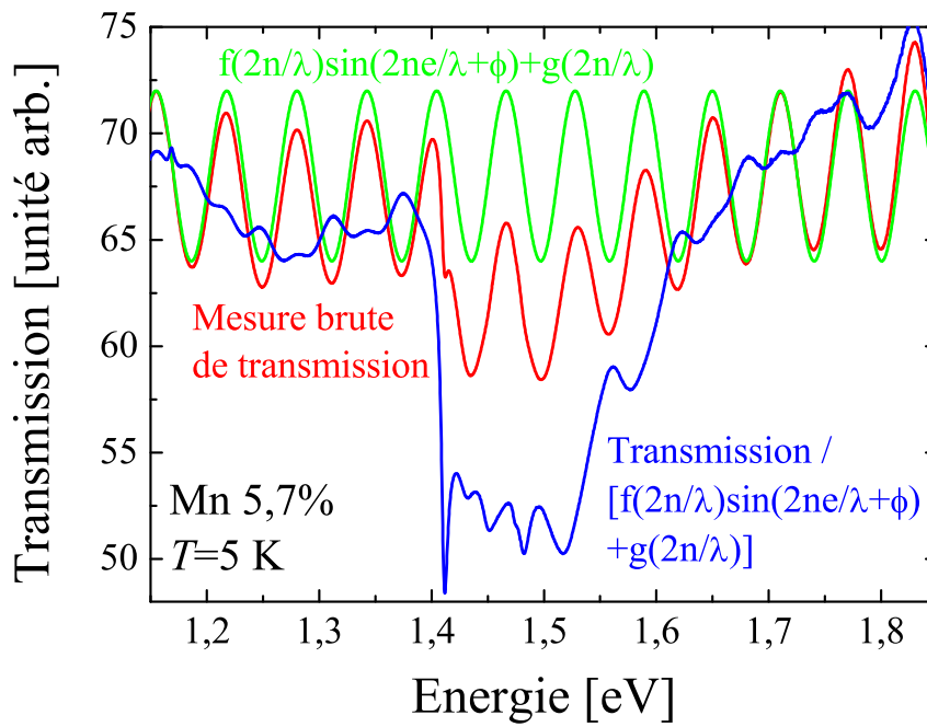
FIG. 3.2: Mesure brute de transmission à 5 K d'une couche dopée à 5,7% (en rouge), fonction sinusoïdale reproduisant les oscillations (en vert) et rapport des deux courbes (en bleu).
