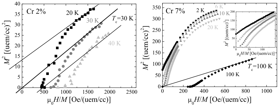
FIG. 1.9: Tracés d'Arrott pour une couche dopée à 2% et 7% (mesures de N. Ozaki).
