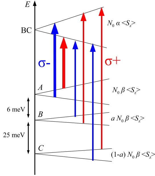
FIG. 2: Levée de dégénérescence des niveaux d'énergie et transitions optiques autorisées pour la structure wurtzite. Les énergies de séparation des bandes sont celles de GaN.
