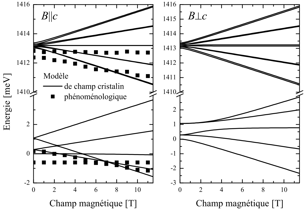
FIG. 2.31: Niveaux d'énergie déterminés phénoménologiquement (carrés) et calculés d'après le modèle de champ cristallin (lignes) du quintuplet fondamental et du niveau {}^5E jusqu'à 11 T avec le champ magnétique parallèle et perpendiculaire à l'axe c .
