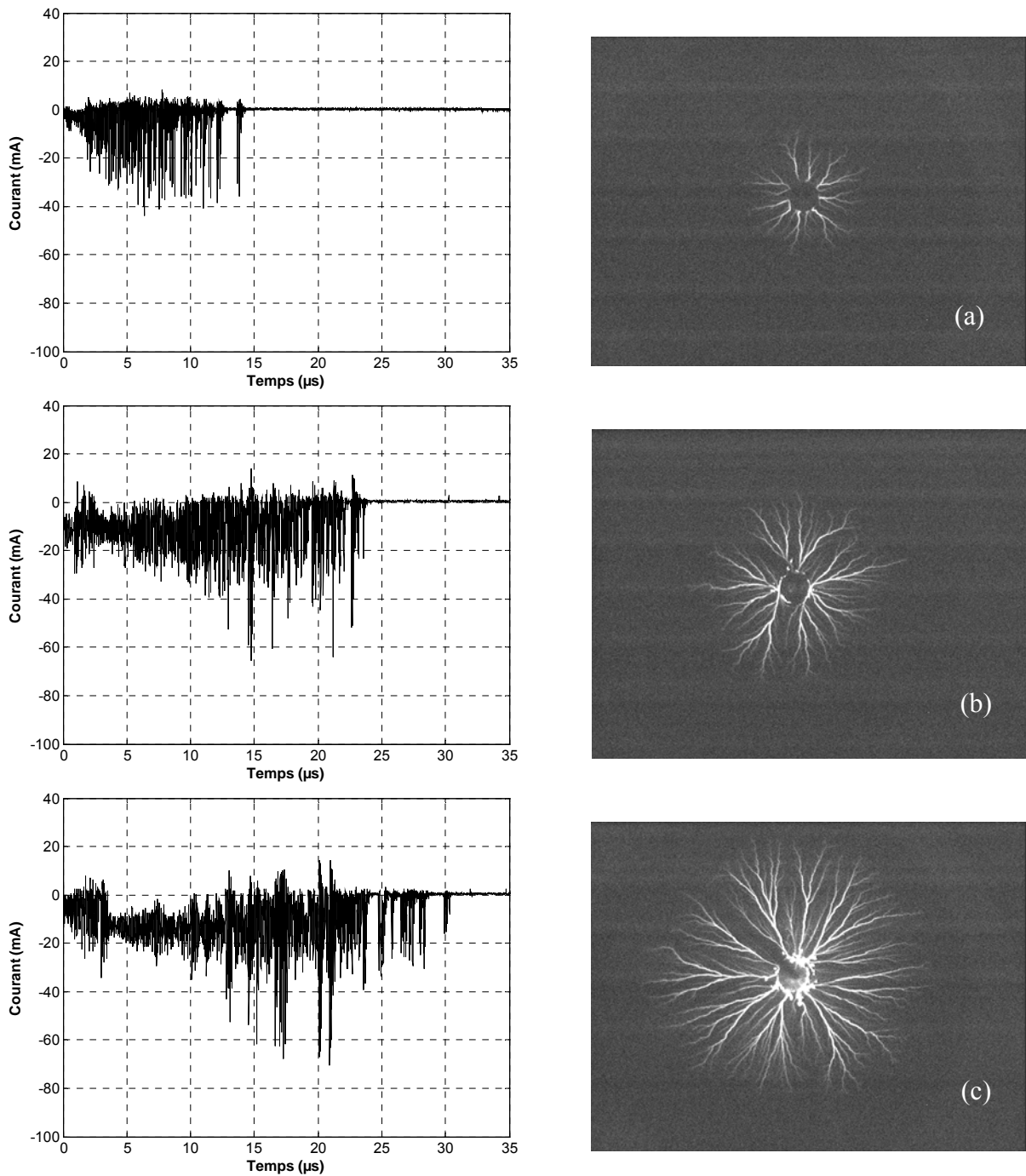
Figure II. 18. Décharges négatives obtenues avec des échantillons en bakélite de 2 mm d'épaisseur et les courants associés pour différentes valeurs de tension : (a) U_{crête} = 16 kV, (b) U_{crête} = 22 kV et (c) U_{crête} = 28 kV.
