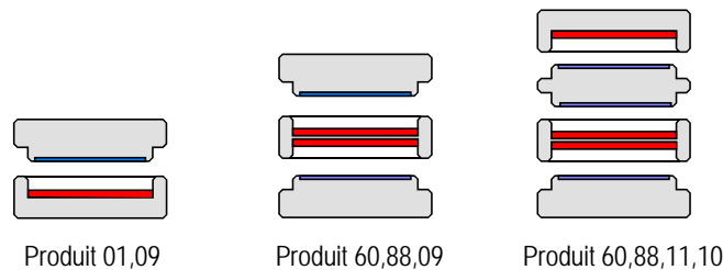
Figure 104 : Exemples de produits assemblés sur le SFP
