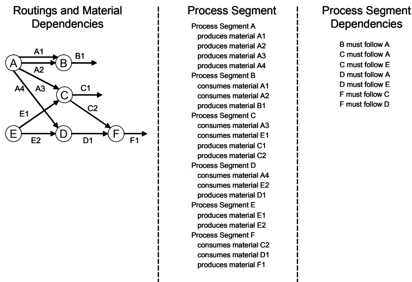
Figure 51 : Routes des produits et dépendances matérielles
