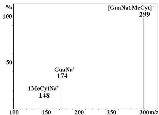
Figure 89 : Spectre CID du dimère [GuaNa1MeCyt] + .
