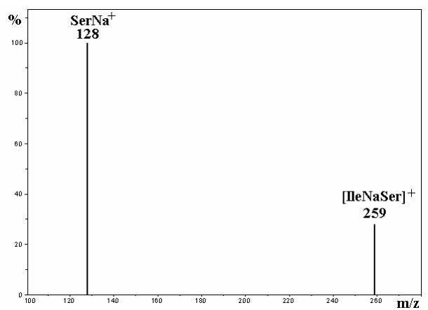
Figure 16 : Spectre CID obtenu après sélection puis fragmentation du dimère [IleNaSer]^+ .
