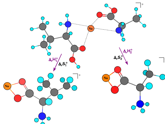
Figure 101 : Fragmentation du dimère [AlacsNaValcs]^+ en AlazwNa^+ et Valzwna^+ .
