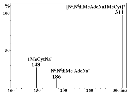
Figure 88 : Spectre CID du dimère [N 6 ,N 6 diMeAdeNa1MeCyt] + .
