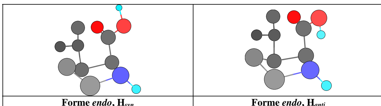
Figure 48 : Forme endo, H syn et forme endo, H anti de la 5-isopropyl proline.
