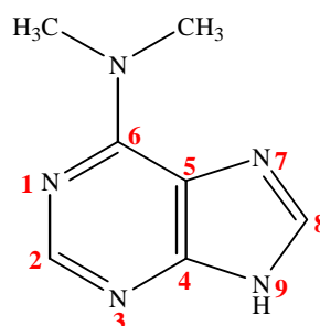
N 6 ,N 6 -diméthyl adénine
