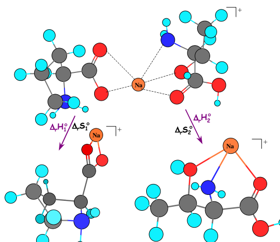
Figure 103 : Fragmentation du dimère [ThrcsNaProzwna]^+ en ThrcsNa^+ et Prozwna^+ .
