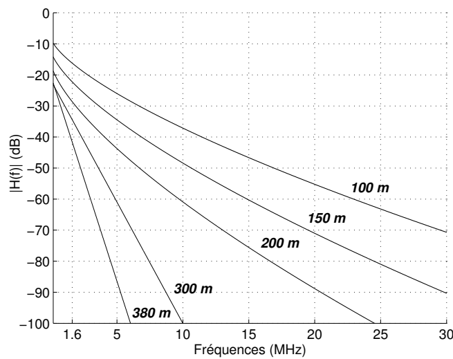
FIG. 1.8 – Profils d'atténuation pour différentes longueurs de ligne
