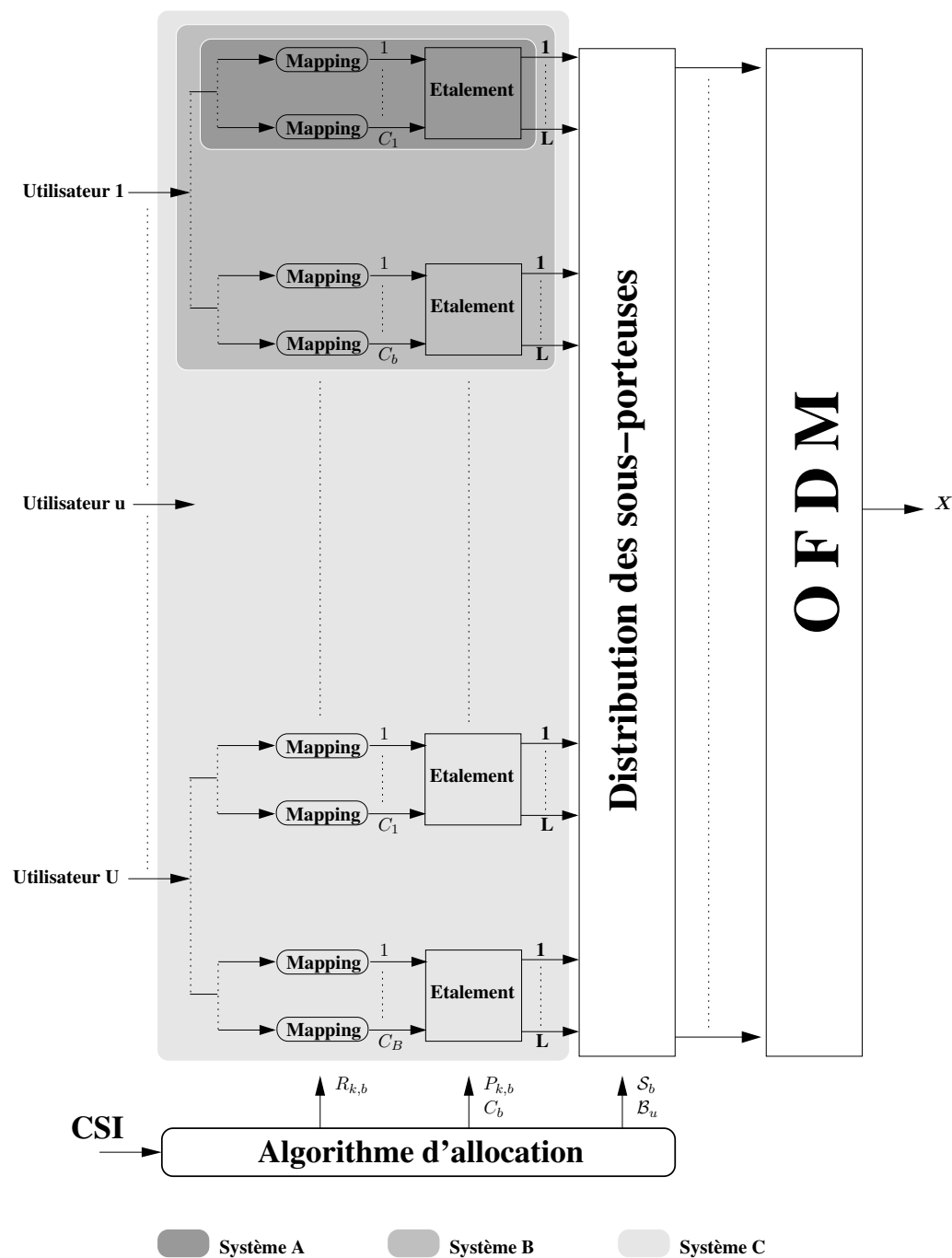
FIG. 7.1 – Schéma représentatif du paramétrage du signal SS-MC-MA par les algorithmes d'allocation dynamique des ressources
