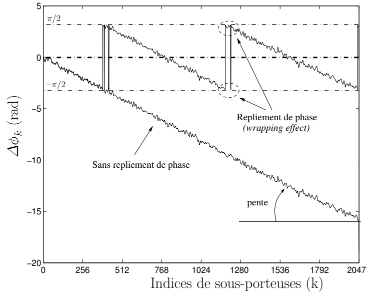
FIG. 4.7 – Effet du repliement de phase ( wrapping effect ) dû à l’ambiguïté de \pm\pi dans le cas d’un décalage de fenêtre de 5 échantillons sur canal gaussien pour un SNR de 0 dB.
