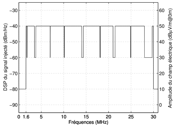
FIG. 1.5 – Exemple de masque de puissance avec prise en compte des fréquences radioamateur. Correspondance entre la puissance du signal CPL injecté sur une ligne et l’amplitude du champ électrique induit à 3 mètres.
