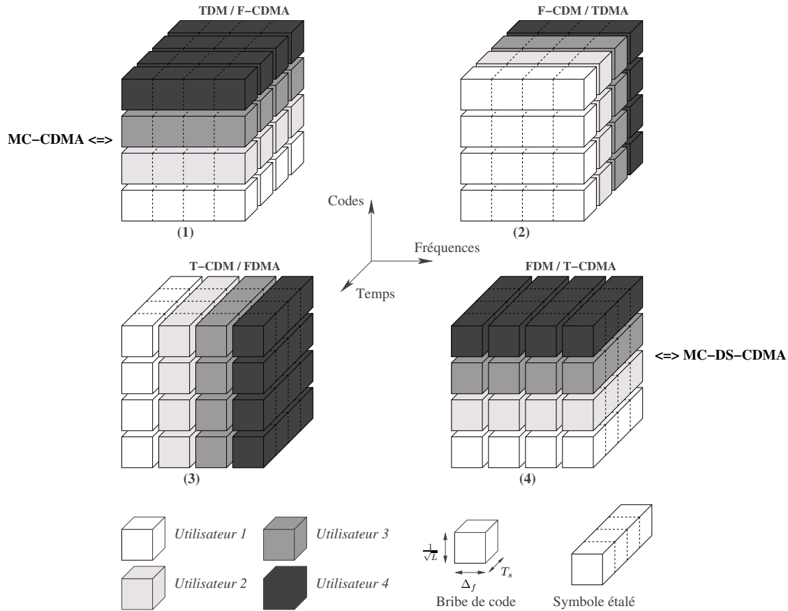
FIG. 2.3 – Représentation schématique du chip mapping des différents systèmes hybrides monoblocs
