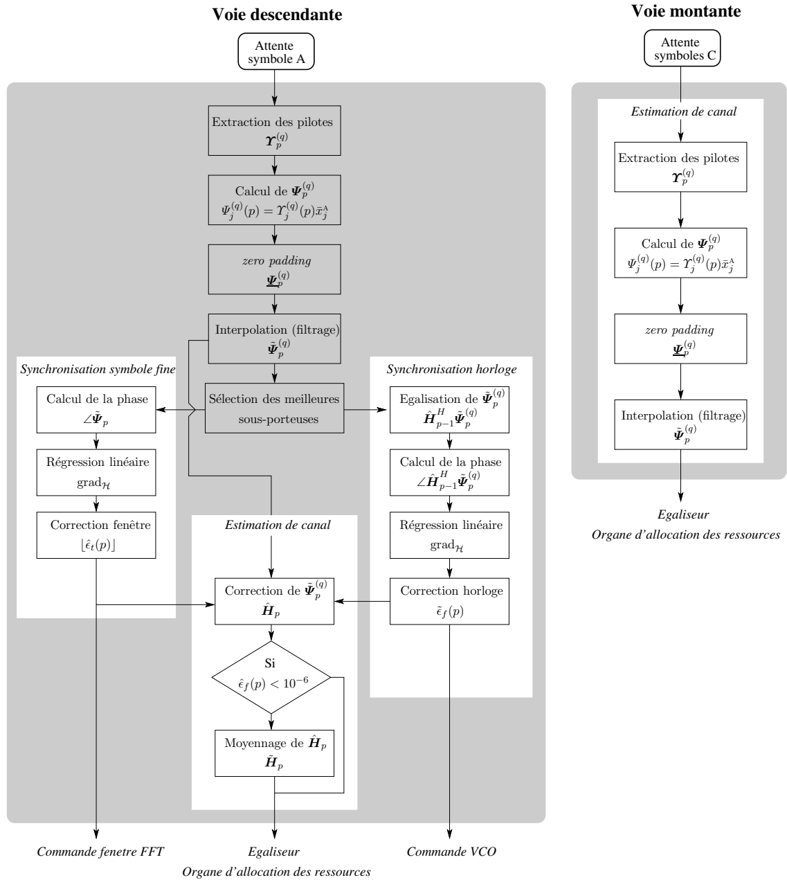
FIG. 4.11 – Synoptiques des fonctions d'estimation mises en œuvre au sein des récepteurs de la voie descendante (à gauche) et de la voie montante (à droite)
