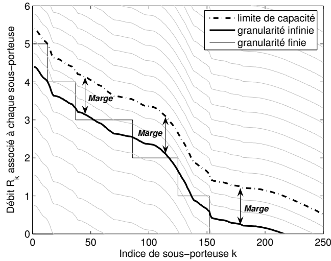
FIG. 6.4 – Comparaison des résultats d'allocation des bits en granularité infinie et finie dans le cadre de la maximisation de la marge de bruit en DMT pour une limitation en DSP et un débit cible donnés.
