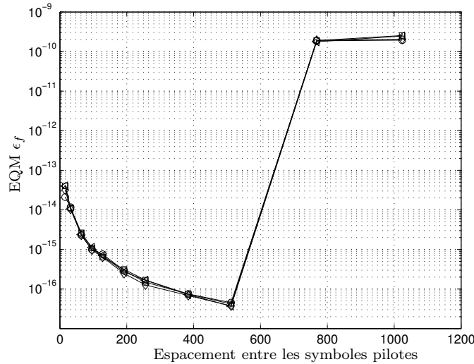
FIG. 5.11 – Évolution de la variance de l'erreur résiduelle \epsilon_f sur la fréquence d'échantillonnage en fonction de l'écart entre les symboles pilotes pour les 4 canaux de référence.
