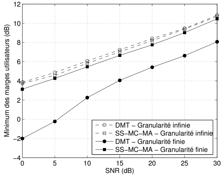
FIG. 7.14 – Comparaison des marges minimales obtenues avec la DMT et le SS-MC-MA en fonction du SNR pour 4 utilisateurs et un facteur d'étalement de L = 64 .
