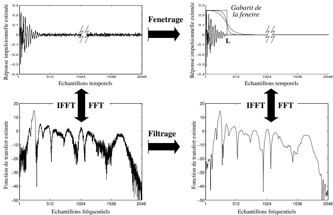
FIG. 4.10 – Principe du filtrage de la réponse fréquentielle estimée
