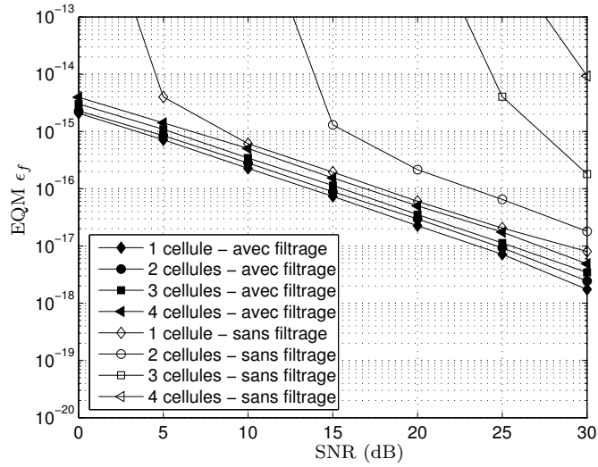
FIG. 5.9 – Variance de l'erreur résiduelle \epsilon_f sur la fréquence d'échantillonnage en fonction du SNR pour différents nombres de cellules adjacentes. Comparaison des résultats avec et sans filtrage de la sortie du filtre adapté.
