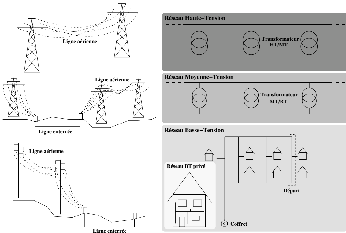
FIG. 1.2 – Structure du réseau de distribution de l'énergie électrique
