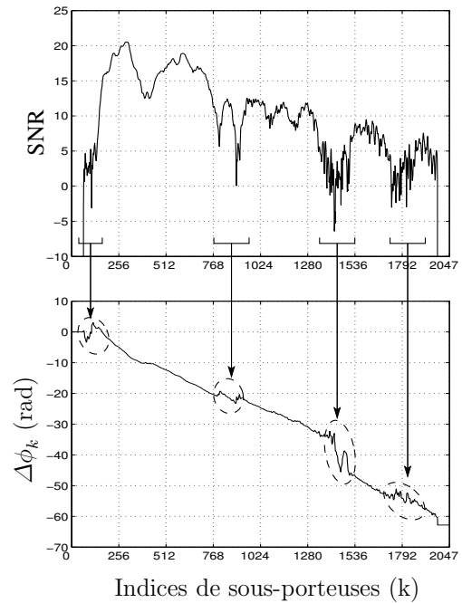
FIG. 4.9 – Influence des évanouissements profonds sur l'allure des différences de phase observées
