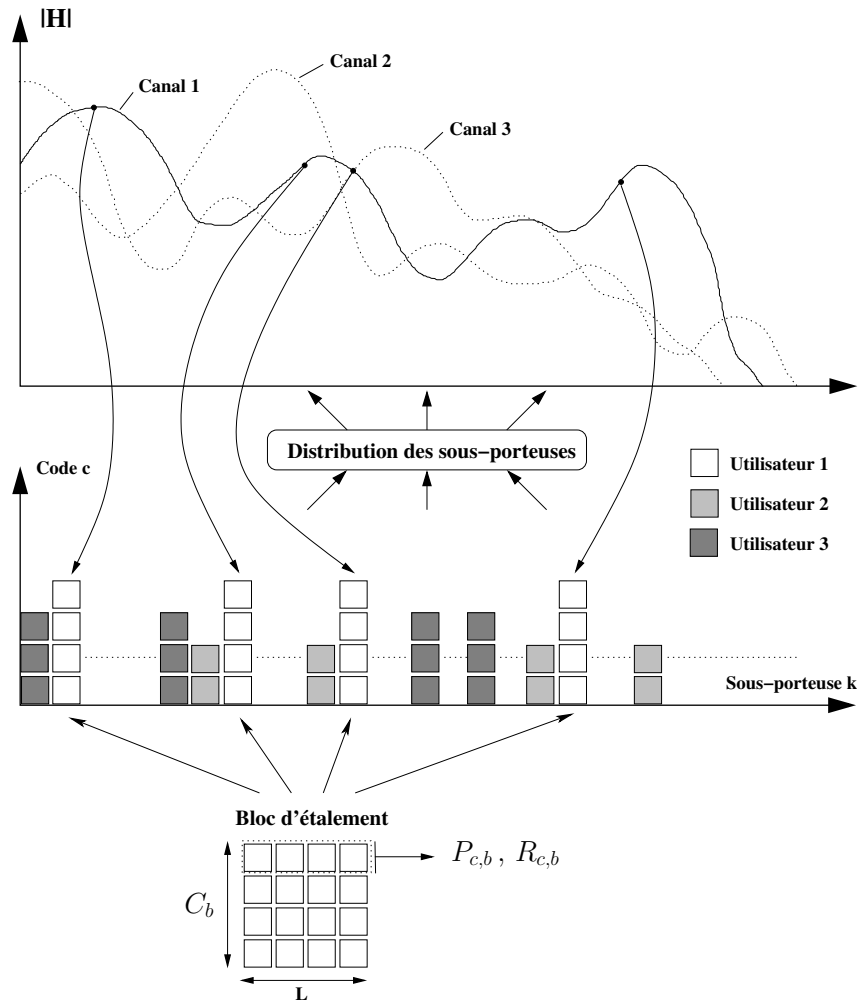
FIG. 7.2 – Principe d'allocation adaptative des ressources dans un système SS-MC-MA multiutilisateur.
