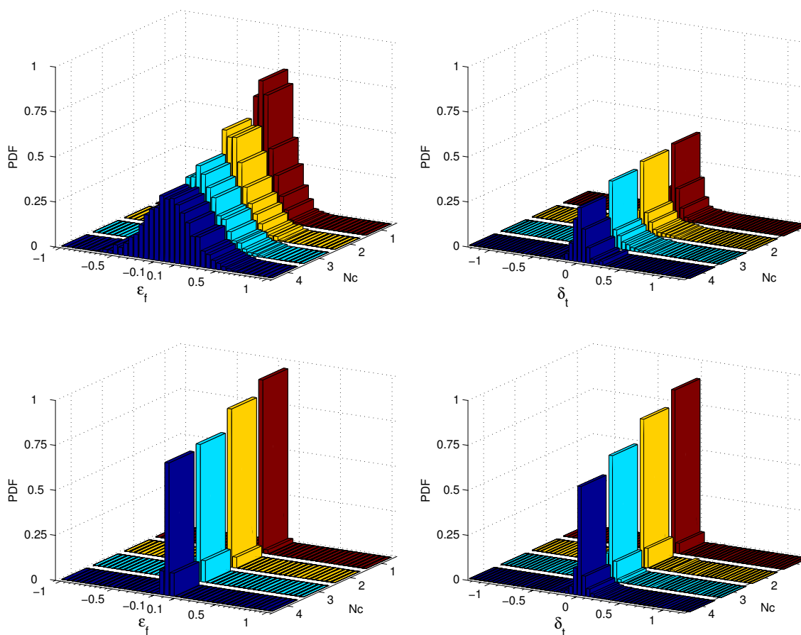
FIG. 5.8 – Densité de probabilité des erreurs résiduelles d'estimation de décalage de la fréquence d'échantillonnage (à gauche) et de décalage de la fenêtre FFT (à droite) après asservissement de l'oscillateur local dans un contexte multicellulaire pour des SNR de 10 dB (en haut) et 30 dB (en bas).
