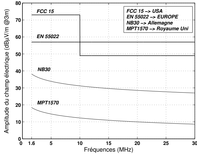
FIG. 1.4 – Différentes propositions de réglementation des seuils d'émission CPL
