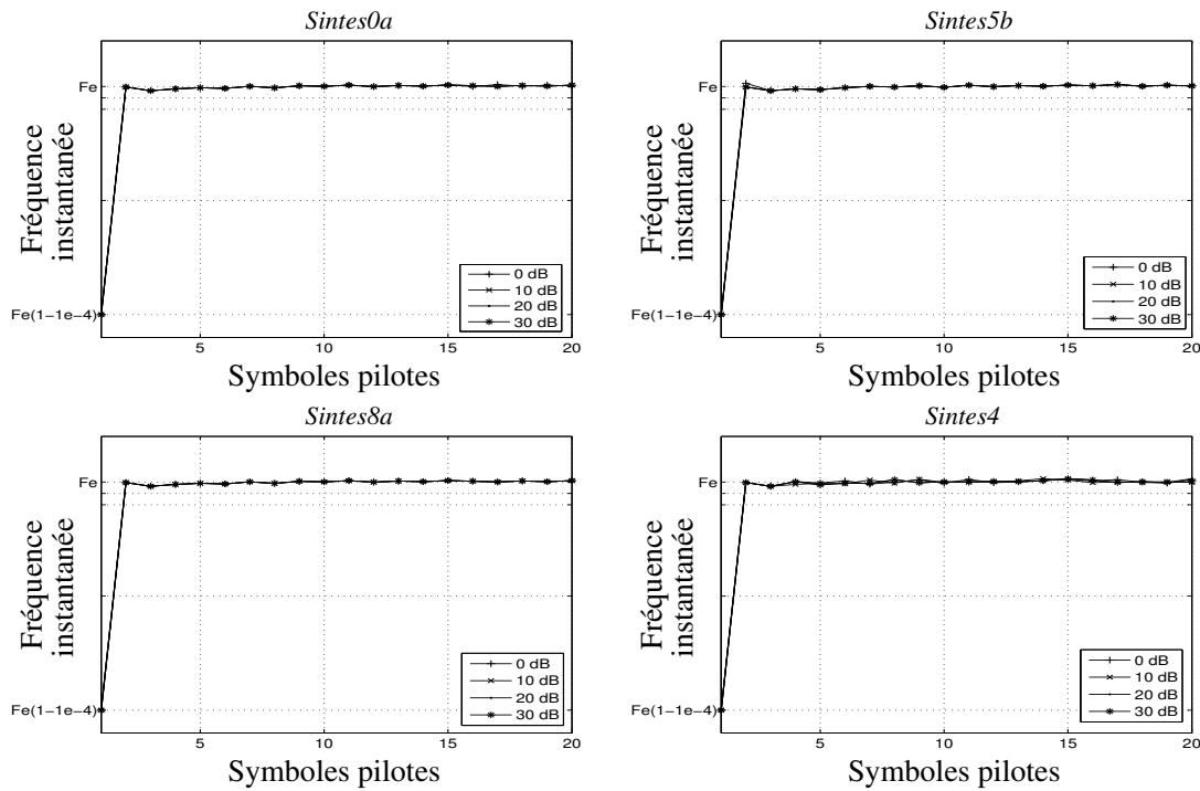
FIG. 5.13 – Résultats de l'estimation du décalage de fréquence d'horloge en phase d'accrochage pour les 4 canaux de référence.
