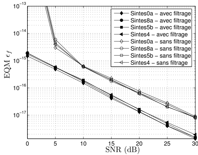
FIG. 5.6 – Variance de l'erreur résiduelle \epsilon_f sur la fréquence d'échantillonnage en fonction du SNR pour les 4 canaux de référence. Comparaison des résultats avec et sans filtrage de la sortie du filtre adapté.
