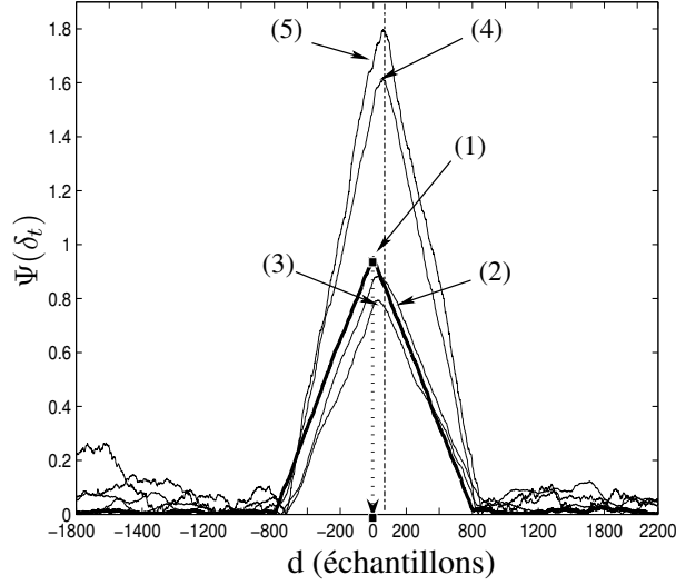
FIG. 4.4 – Résultat du moyennage de la fonction de corrélation pour différents scénarios : (1) canal AWGN, \epsilon_f = 0 , SNR=10 dB, 1 cellule — (2) canal Sintesa , \epsilon_f = 0 , SNR=10 dB, 1 cellule — (3) canal Sintesa , \epsilon_f = 10^{-4} , SNR=10 dB, 1 cellule — (4) canal Sintesa , \epsilon_f = 10^{-4} , SNR=10 dB, 4 cellules — (5) canal Sintesa , \epsilon_f = 10^{-4} , SNR=0 dB, 4 cellules.
