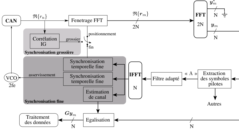
FIG. 4.12 – Principe général du fonctionnement d'un récepteur à porteuses multiples de la voie descendante, incluant les organes de synchronisation et d'estimation de canal mis en œuvre dans le domaine temporel.
