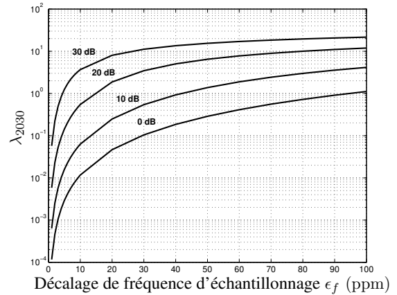
FIG. 3.4 – Dégradation du SNR en fonction de l'erreur d'échantillonnage \epsilon_f pour la sous-porteuse la plus défavorisée et pour différents SNR de réception
