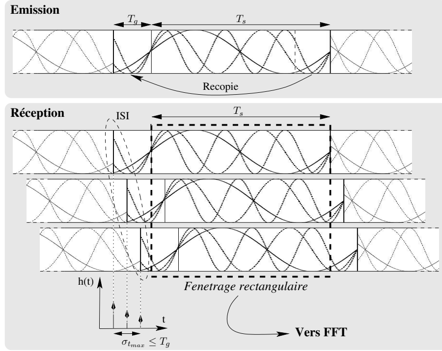
FIG. 2.2 – Fonctionnement de l'intervalle de garde ou préfixe cyclique
