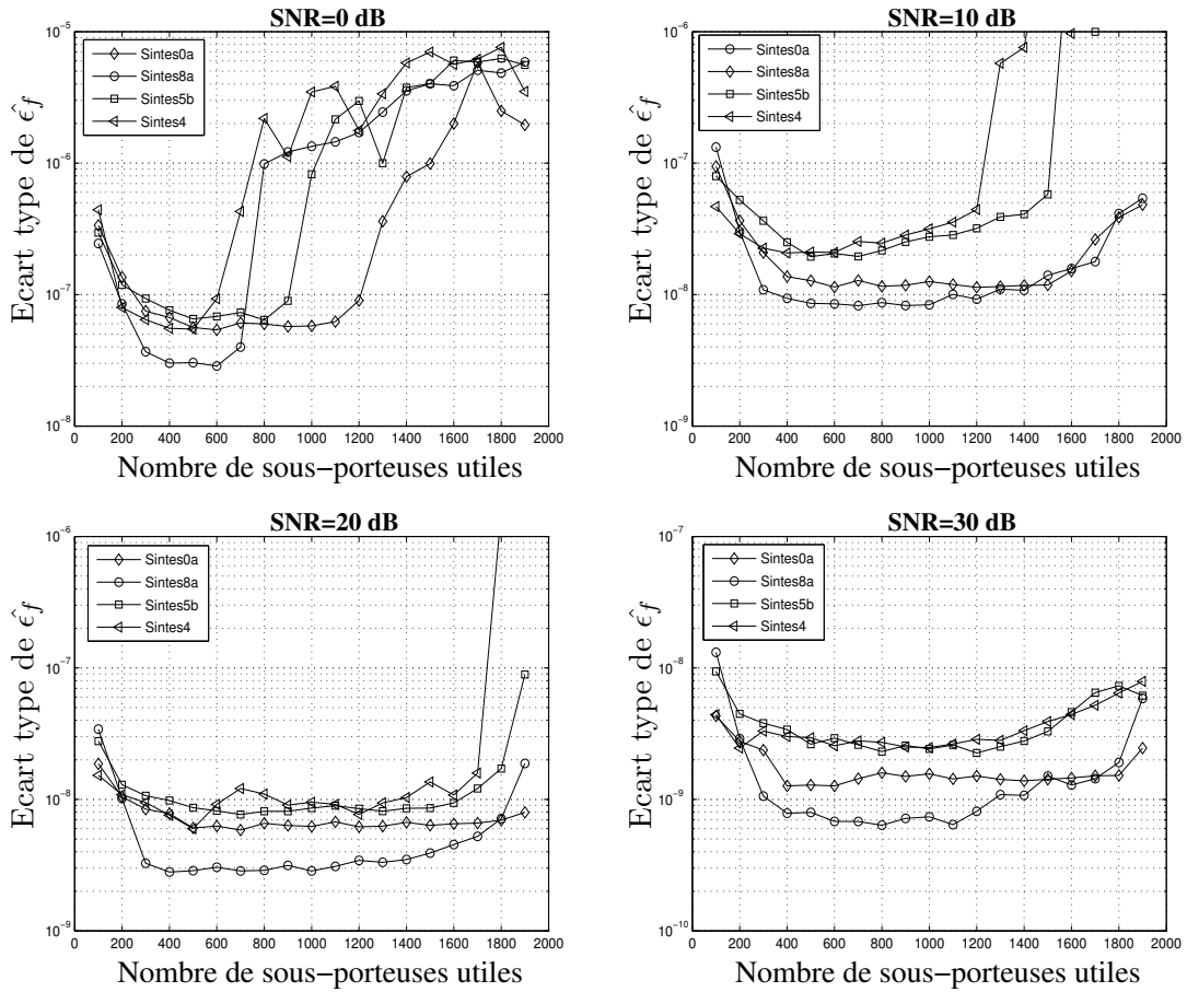
FIG. 5.1 – Evolution de l'erreur d'estimation du décalage de fréquence d'échantillonnage en fonction du nombre de sous-porteuses utilisées et pour différents SNR.
