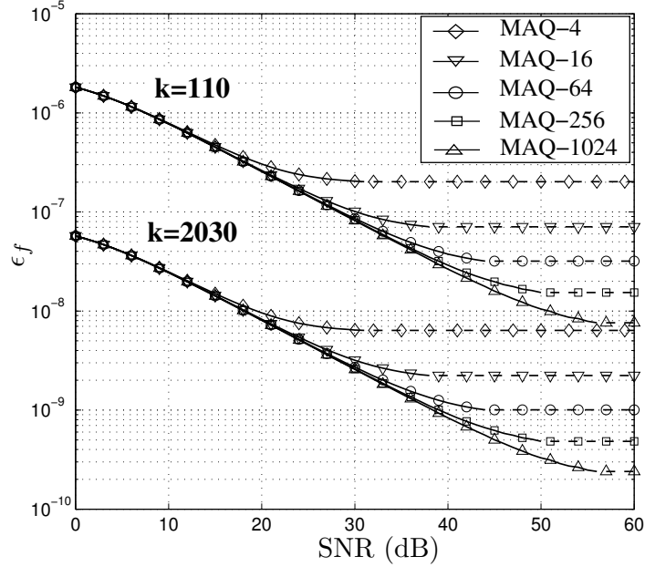
FIG. 3.6 – Précision minimale requise par l'oscillateur local en fonction du SNR de réception pour garantir une dégradation du SNR de moins de 0,1 dB subies par différentes sous-porteuses du spectre. La longueur des trames est de M = 128 .
