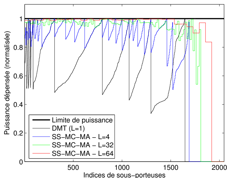
FIG. 7.9 – Évolution de la répartition des puissances en fonction du facteur d'étalement (SNR=20 dB).
