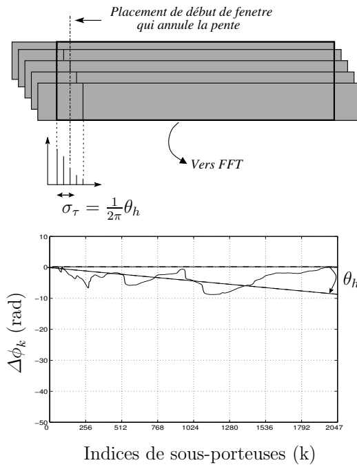
FIG. 4.8 – Influence de la phase du canal sur l'allure des différences de phase observées
