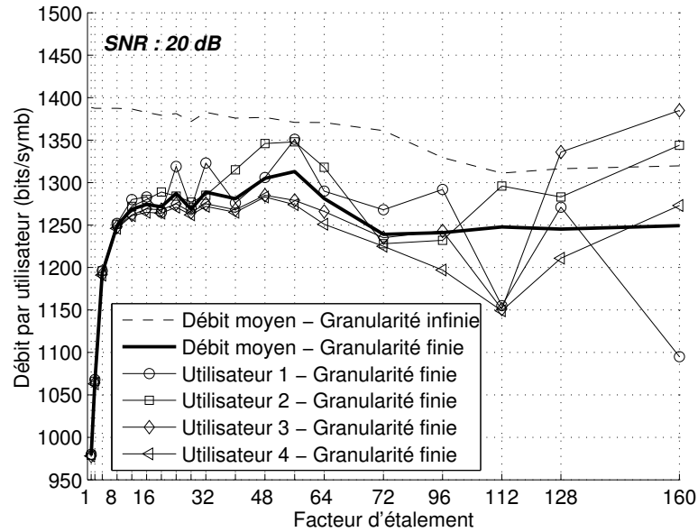
FIG. 7.10 – Comparaison des débits obtenus par utilisateur avec la DMT et le SS-MC-MA en fonction du facteur d'étalement pour 4 utilisateurs et un SNR de 20 dB.
