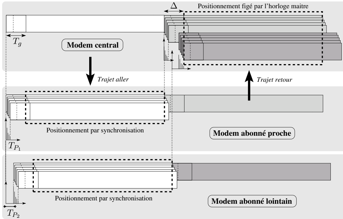
FIG. 2.6 – Synchronisation du réseau par surdimensionnement de l'intervalle de garde
