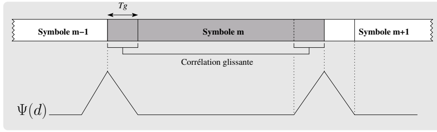
FIG. 4.2 – Principe de synchronisation symbole par corrélation de l'intervalle de garde
