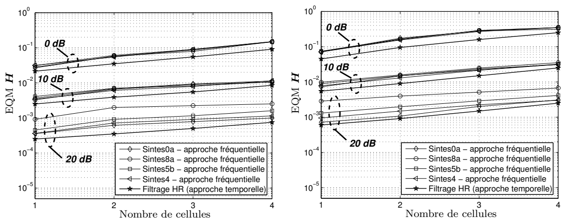
FIG. 5.22 – Comparaison de la variance de l’erreur d’estimation du canal entre les approches fréquentielle et temporelle en voies descendante (gauche) et montantes (droite) en contexte multicellulaire.
