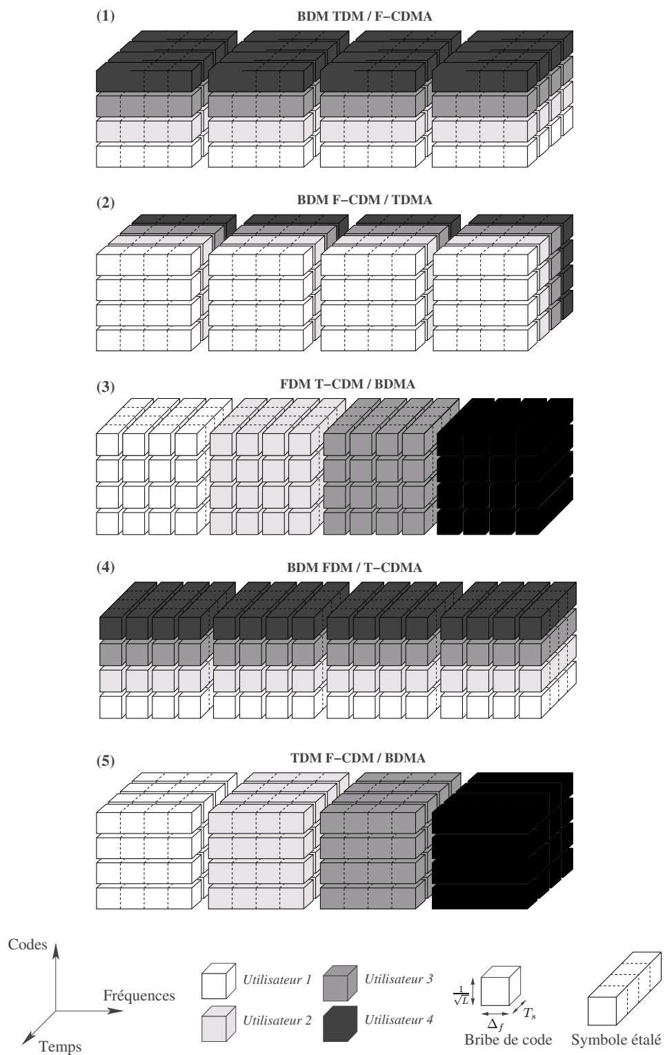
FIG. 2.4 – Représentation schématique du chip mapping des différents systèmes hybrides multiblocs
