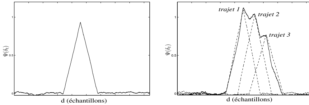
FIG. 4.3 – Effet des trajets multiples sur la fonction de corrélation moyennée sur 10 symboles successifs. À gauche, canal AWGN, à droite canal à trois trajets.
