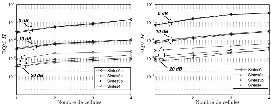
FIG. 5.10 – Variance de l'erreur d'estimation du canal en voies descendante (gauche) et montante (droite) en fonction du nombre de cellules actives.
