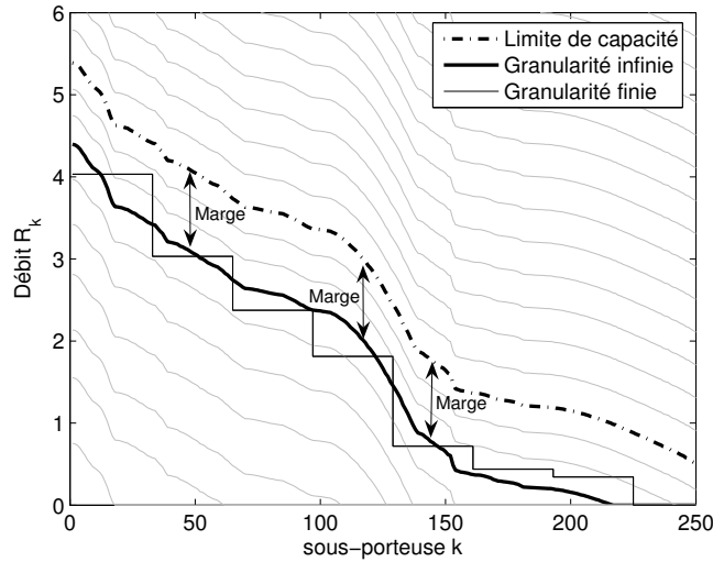
FIG. 7.7 – Comparaison des résultats de l'allocation des puissances en granularité infinie et finie dans le cadre de la maximisation de la marge de bruit du système B pour un débit cible donné.
