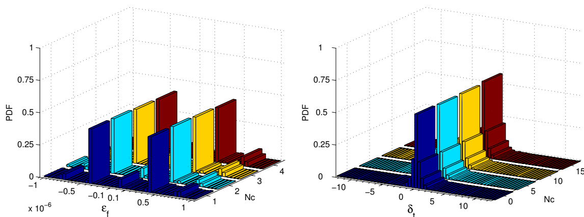
FIG. 5.18 – Densité de probabilité des erreurs résiduelles d'estimation de décalage de la fréquence d'échantillonnage (à gauche) et de décalage de la fenêtre FFT (à droite) après asservissement de l'oscillateur local dans un contexte multicellulaire pour un SNR de 10 dB.
