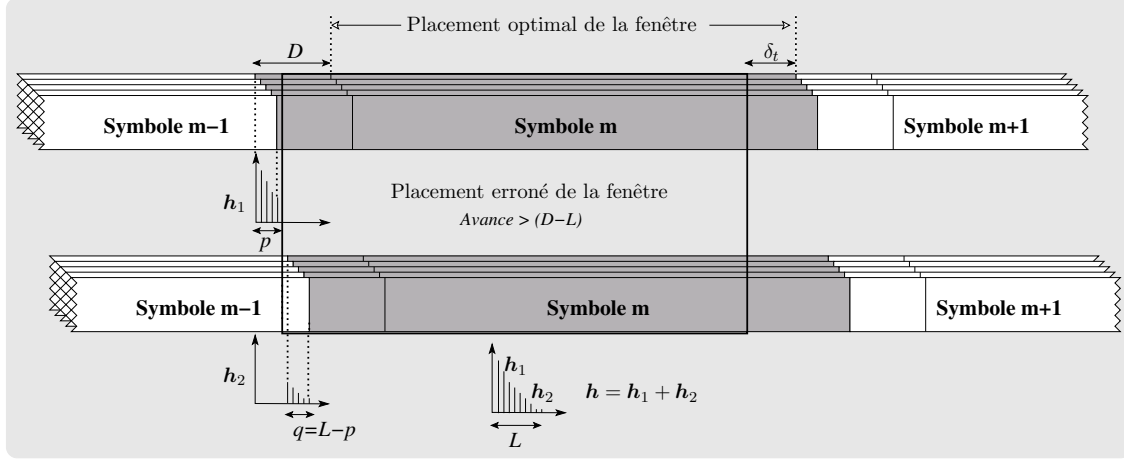
FIG. B.1 – Représentation du placement erroné de la fenêtre FFT en avance sur sa position optimale. Illustration du principe de découpage de la réponse impulsionnelle en deux réponses successives \mathbf{h}_1 et \mathbf{h}_2 .
