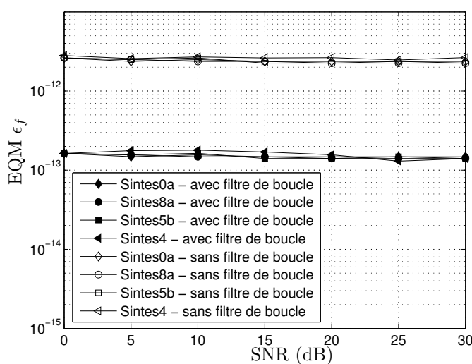
FIG. 5.16 – Variance de l'erreur résiduelle \epsilon_f sur la fréquence d'échantillonnage en fonction du SNR pour les 4 canaux de référence. Comparaison des résultats avec et sans mise en œuvre du filtre de boucle.
