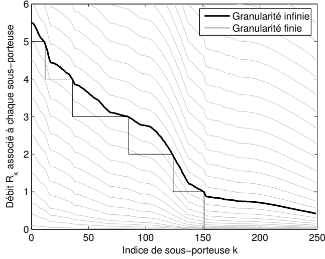
FIG. 6.2 – Comparaison des résultats d'allocation des bits en granularité infinie et finie, dans le cadre de la maximisation du débit en DMT pour une limitation en DSP donnée.
