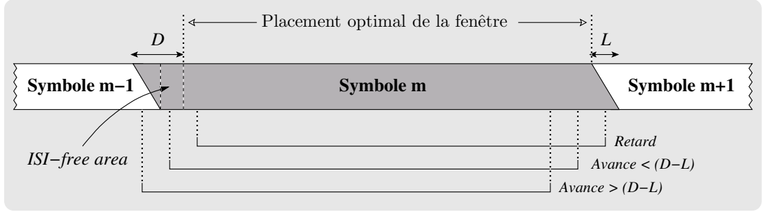
FIG. 3.1 – Représentation schématique des trois scénarios de défaut de placement de la fenêtre FFT en réception du signal à porteuses multiples
