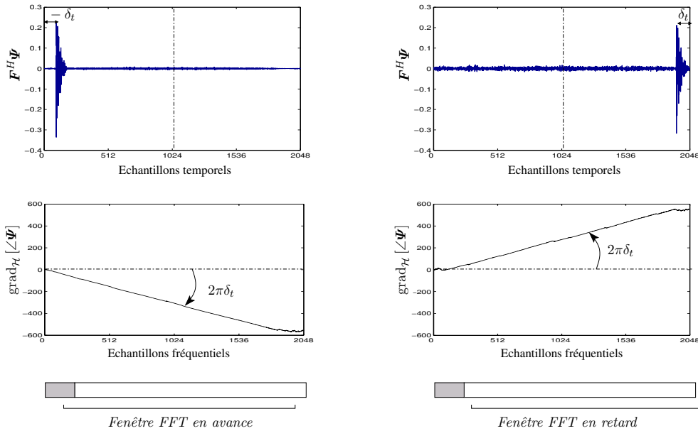
FIG. 4.13 – Représentation des conséquences d’un décalage de fenêtre FFT sur la visualisation de la réponse impulsionnelle du canal et sur la pente de la droite de régression calculée sur la phase du signal obtenu en sortie du filtre adapté.
