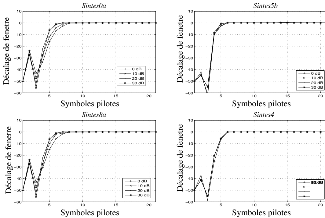
FIG. 5.3 – Résultats de l'estimation du décalage de fenêtre FFT en phase d'accrochage pour les 4 canaux de référence.
