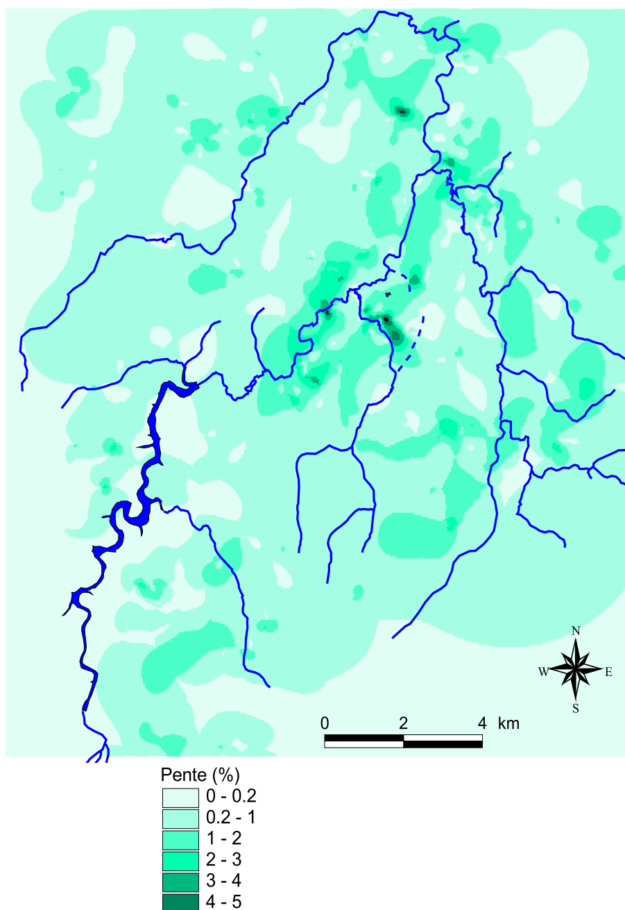
Figure 1-28. Carte des pentes du niveau de transition calculé
