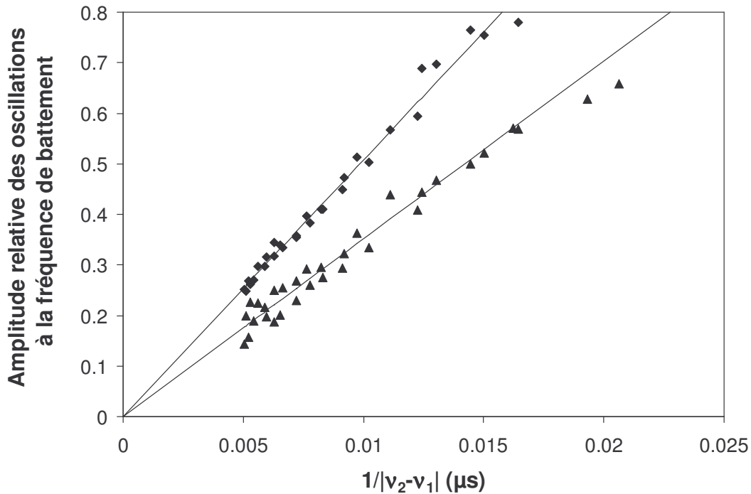
Figure II-11 : Evolution des amplitudes relatives des oscillations à la fréquence de battement de chaque laser en fonction de l'inverse du désaccord entre les lasers.
