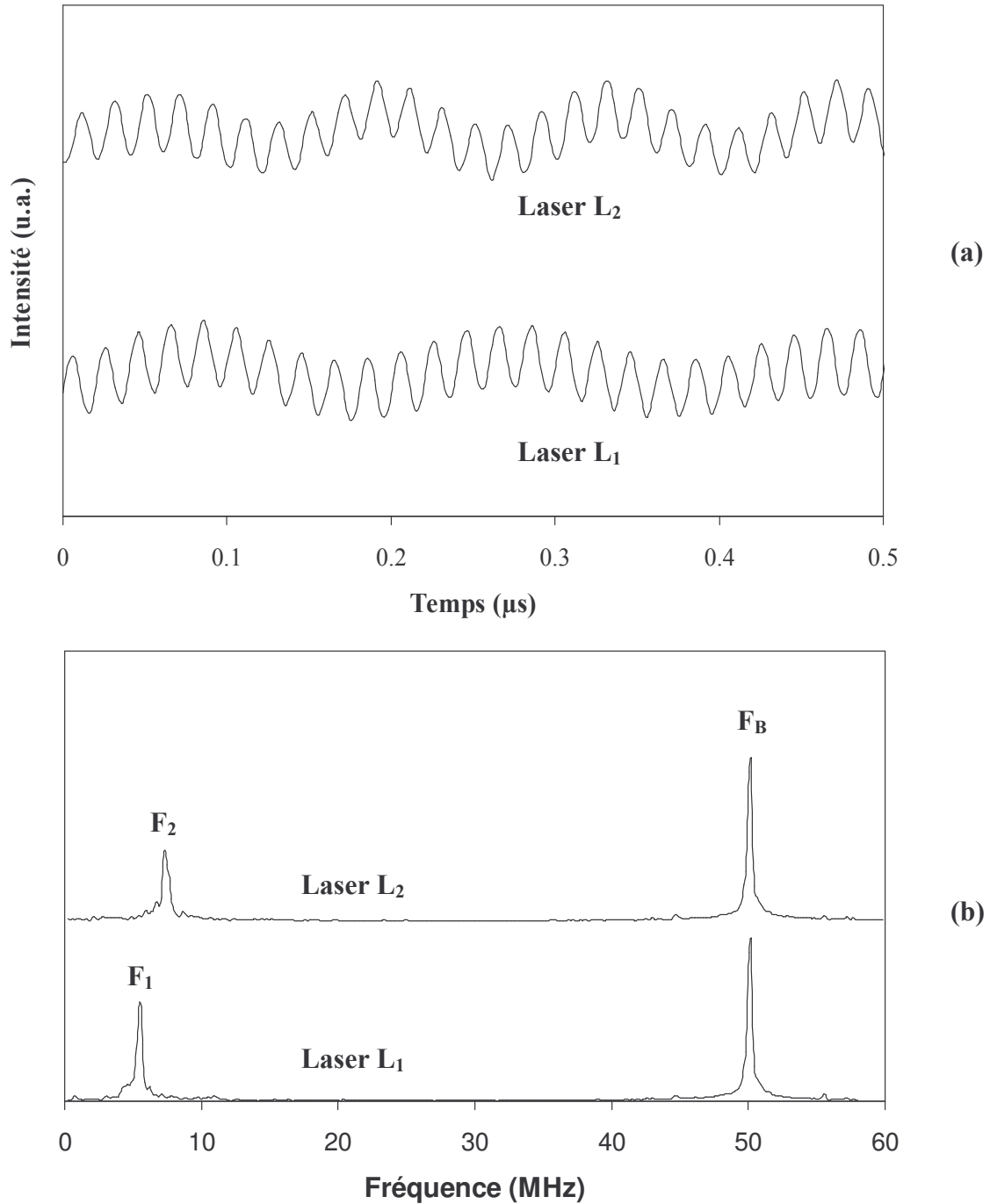
Figure II-4 : Exemple de régimes observés pour les grands désaccords : (a) Evolution temporelle de l'intensité émise par chaque laser et (b) spectres basse fréquence associés. Mêmes conditions expérimentales que la Figure II-3.
