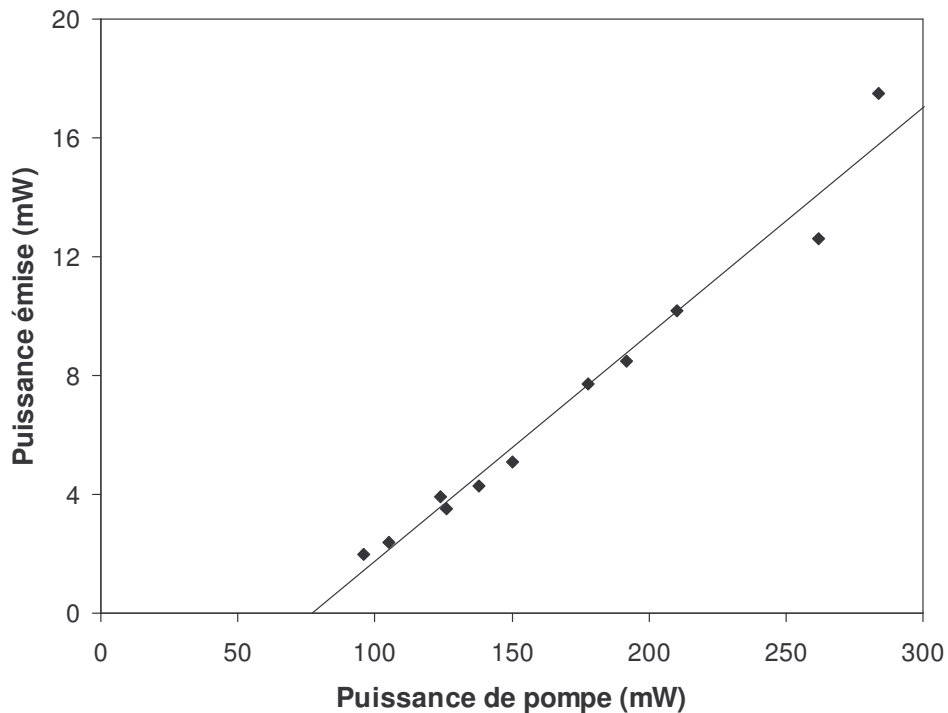
Figure I-12 : Puissance émise par le microlaser en fonction de la puissance de pompe.
