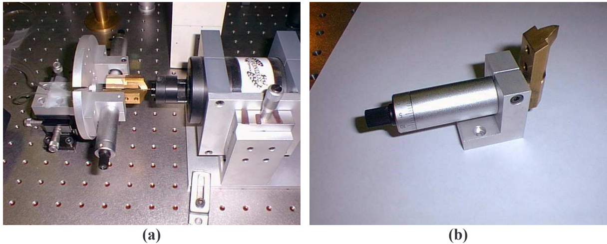
Figure II-1: Dispositif de positionnement des fibres, (a) vue globale, (b) la mâchoire du mandrin solidaire de son système de translation micrométrique
