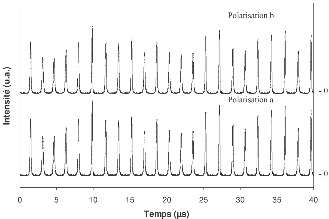
Figure III–7 : Exemple d'évolution temporelle des intensités des polarisations a et b dans le cas d'une faible anisotropie de cavité (désaccord \approx 15 MHz ; P_p/P_{ps} = 3,8 , \theta_p \approx 40^\circ ).
