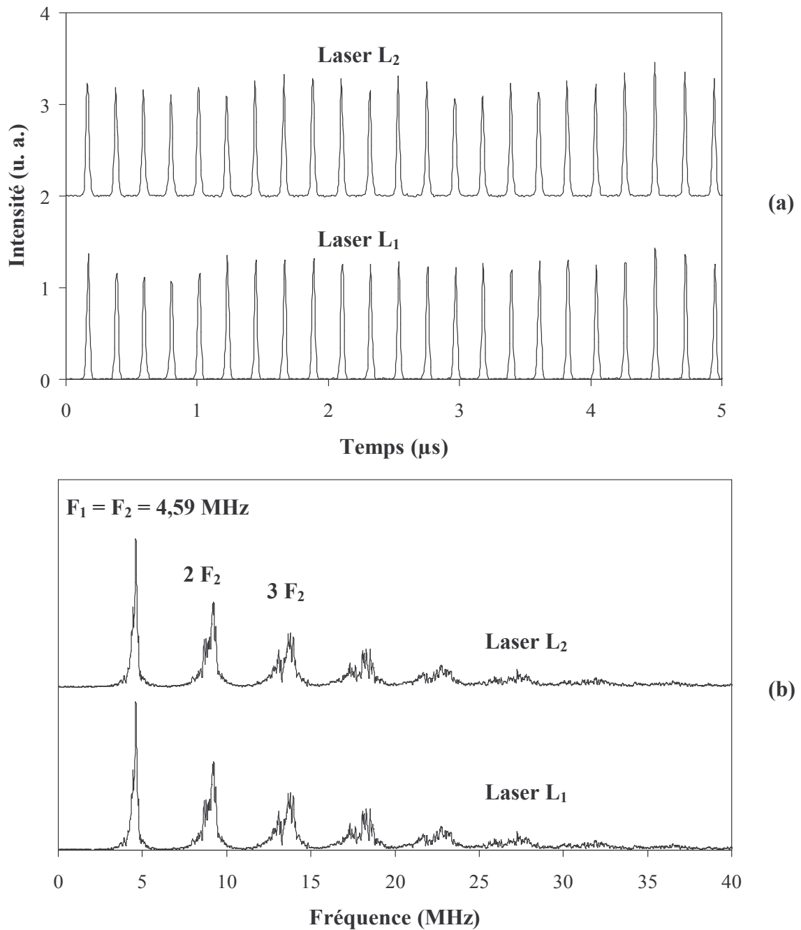
Figure II-6 a) Evolution temporelle de l'intensité émise par chaque laser et b) spectres basse fréquence associés. Mêmes conditions expérimentales que la Figure II-3. Désaccord de fréquence -8 \text{ MHz} . Les signaux temporels associés au laser L 2 ont subi un décalage d'origine des intensités de deux unités.
