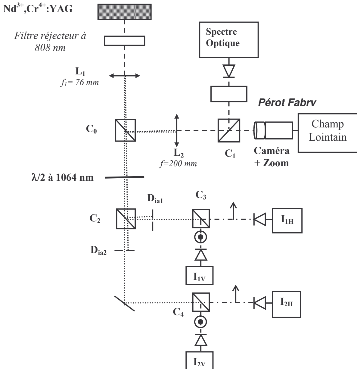
Figure III–13 : Dispositif d'analyse de la dynamique de deux microlasers \text{Nd}^{3+}, \text{Cr}^{4+}:\text{YAG} couplés ( C_0, C_1 et C_2 = cubes séparateurs de faisceaux ; C_3 et C_4 = cubes séparateurs de polarisations ; D_{ia} = diaphragme)
