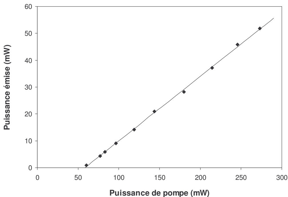
Figure I-6 : Puissance émise (à 1064 nm) en fonction de la puissance de pompe (à 808 nm)
