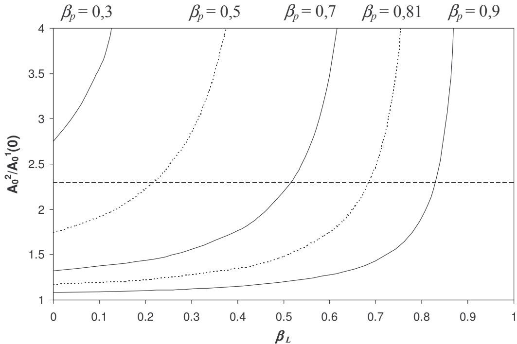
Figure III-8 : Evolution du rapport théorique entre le seuil du second mode et le seuil du premier mode en fonction de \beta_L pour différentes valeurs de \beta_p ( \Psi_p=0 ).
