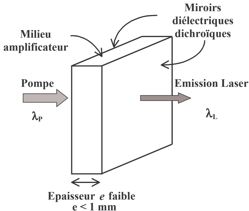
Figure I-1: Pompage longitudinal d'un microlaser plan-plan.
