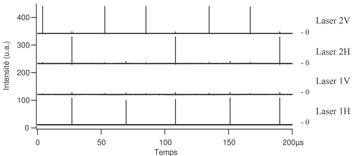
Figure III-16 : Intensité émise par chaque laser dans les deux directions de polarisation H et V dans la cas d'une synchronisation harmonique
