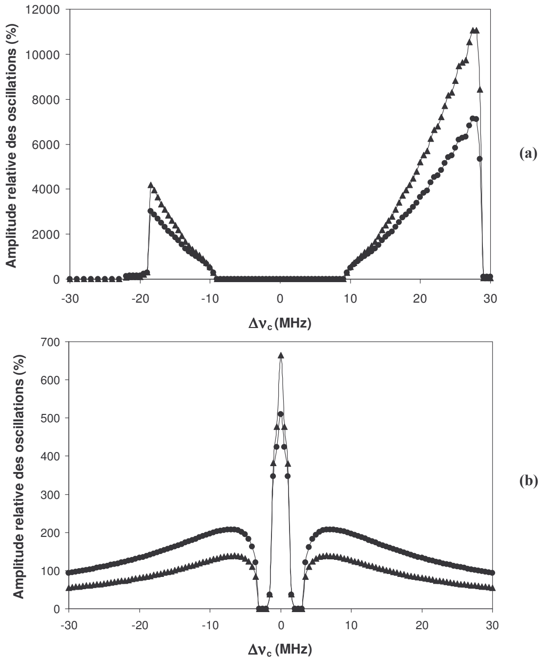
Figure II-19 : Evolution des amplitudes relatives des oscillations en fonction du désaccord pour un couplage purement réel (a) et purement imaginaire (b).
