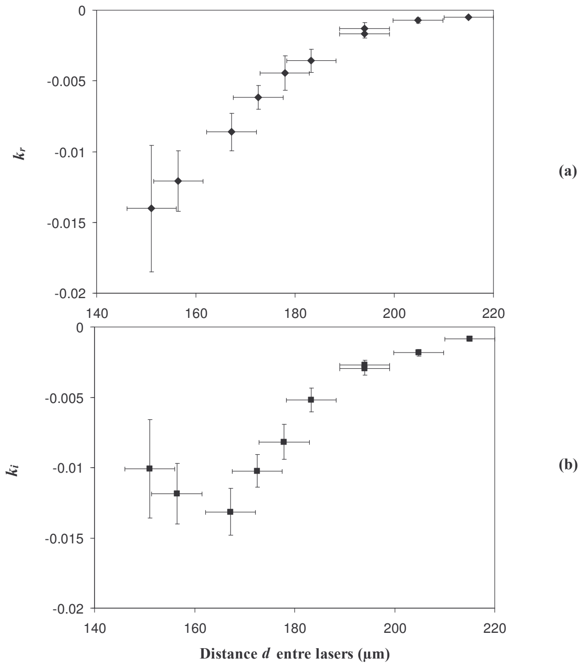
Figure II-14 : Evolution de la partie réelle k_r (a) et imaginaire k_i (b) en fonction de la distance entre les lasers.
