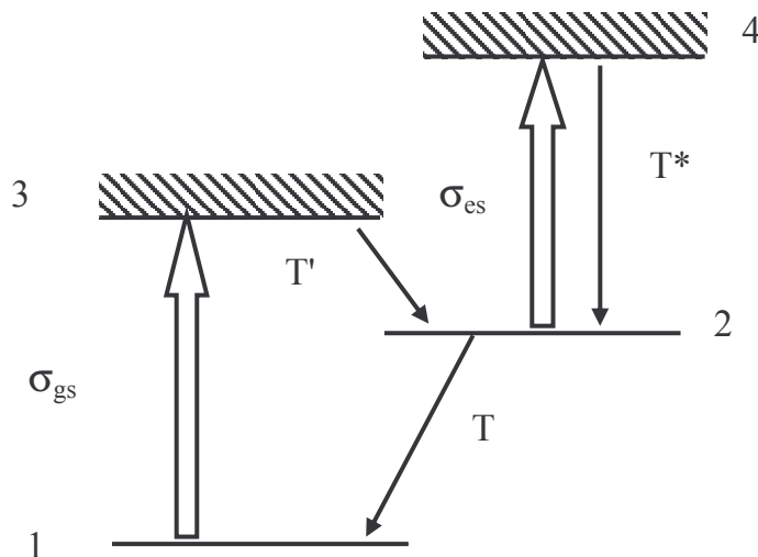
Figure I-14 : Diagramme des niveaux d'énergie impliqués dans le processus d'absorption saturée du Cr 4+ :YAG.
