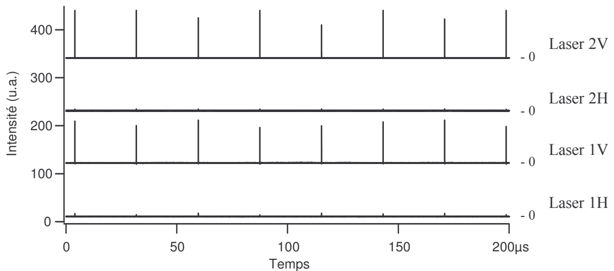
Figure III-15 : Exemple de l'intensité émise par les deux lasers dans les deux directions H et V lorsque les lasers sont synchronisés
