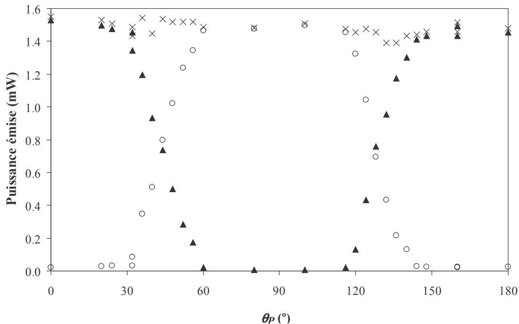
Figure III-3 : Evolution de la puissance émise dans les modes a (▲) et b (○) en fonction de la direction de la polarisation du faisceau de pompe pour un microlaser pompé légèrement au dessus du seuil ( P_p/P_{ps} = 1,4 , désaccord entre modes \approx 86 MHz). (×) puissance totale .
