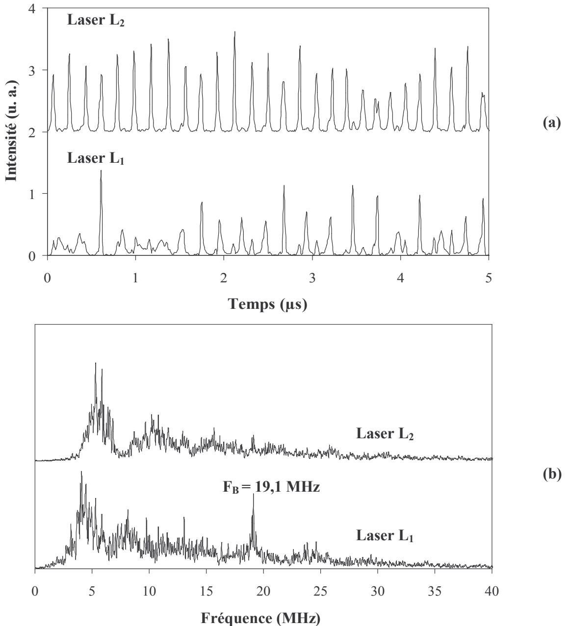
Figure II-8 : Exemple de régimes instables pour les désaccords négatifs. a) Evolution temporelle de l'intensité émise par chaque laser et b) spectres associés.
