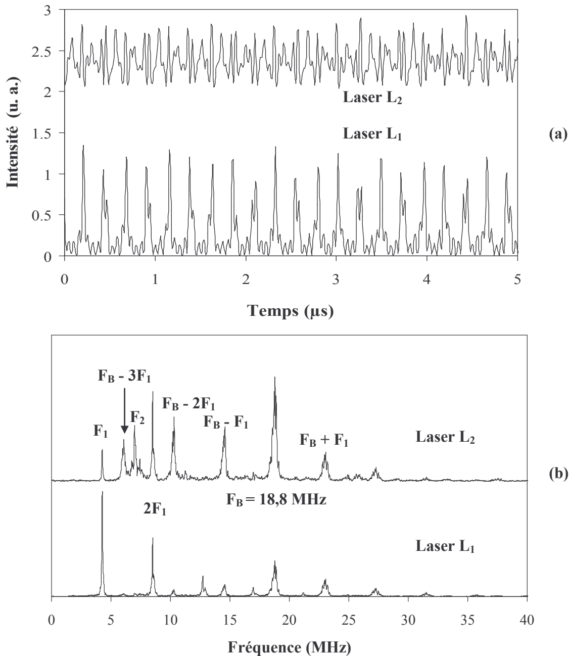
Figure II–7 : Exemple de régimes instables pour un désaccord positif. a) Evolution temporelle de l'intensité émise par chaque laser et b) spectres basse fréquence associés.
