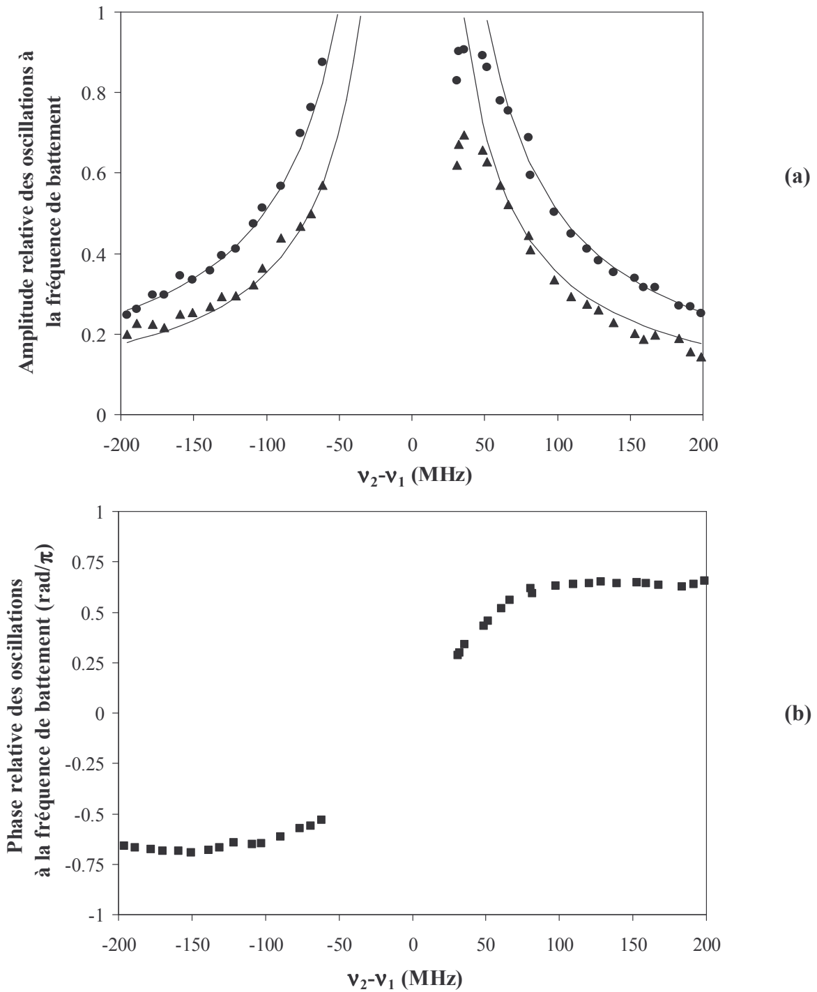
Figure II–10 : a) Amplitude relative des oscillations d'intensité à la fréquence de battement pour les deux lasers ( \bullet L_1 , \blacktriangle L_2 ), en trait plein, les hyperboles ajustées sur les données expérimentales. b) Différence de phase entre les oscillations du laser L_2 par rapport au laser L_1 .
