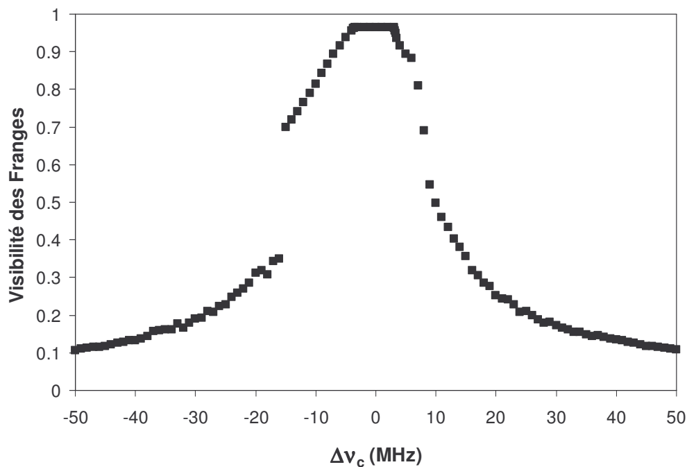
Figure II-17 : Évolution de la visibilité du système de franges en fonction du désaccord des cavités (conditions de la Figure II-15).
