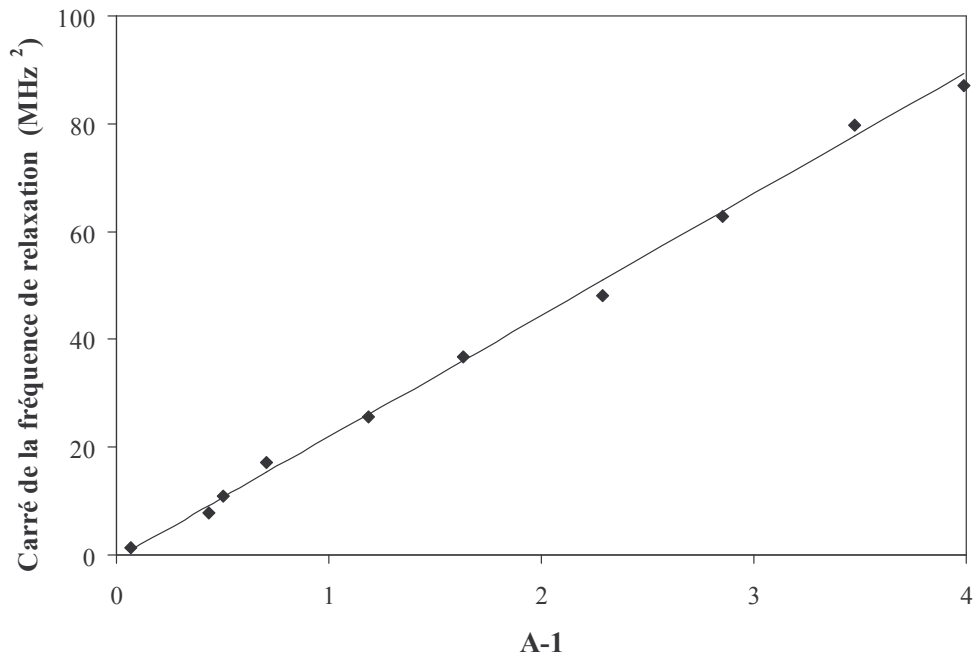
Figure I-10 : Evolution du carré de la fréquence de relaxation du laser en fonction de l'excès de pompe par rapport au seuil ( A-1 ). Les losanges représentent les points expérimentaux tandis que la courbe en trait plein est la droite passant par l'origine ajustée sur les points expérimentaux (pente = 23 \text{ MHz}^2 ).
