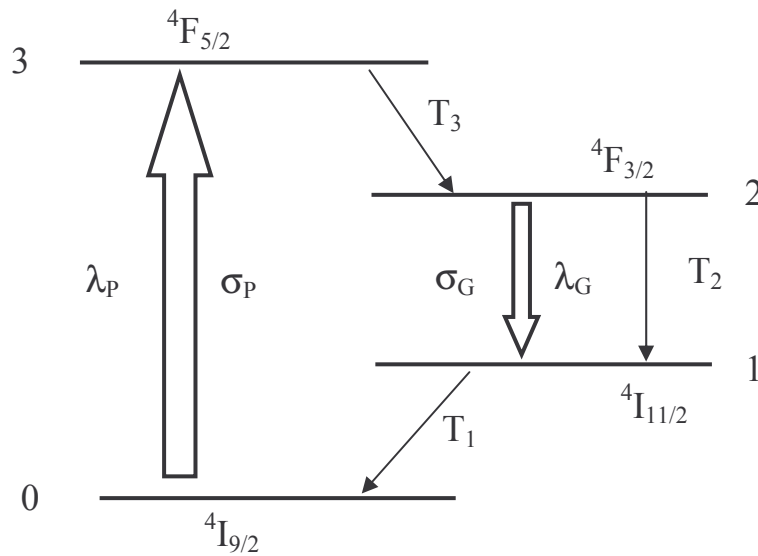
Figure I-3 : Diagramme des 4 niveaux impliqués dans l'effet laser de l'ion néodyme \text{Nd}^{3+}
