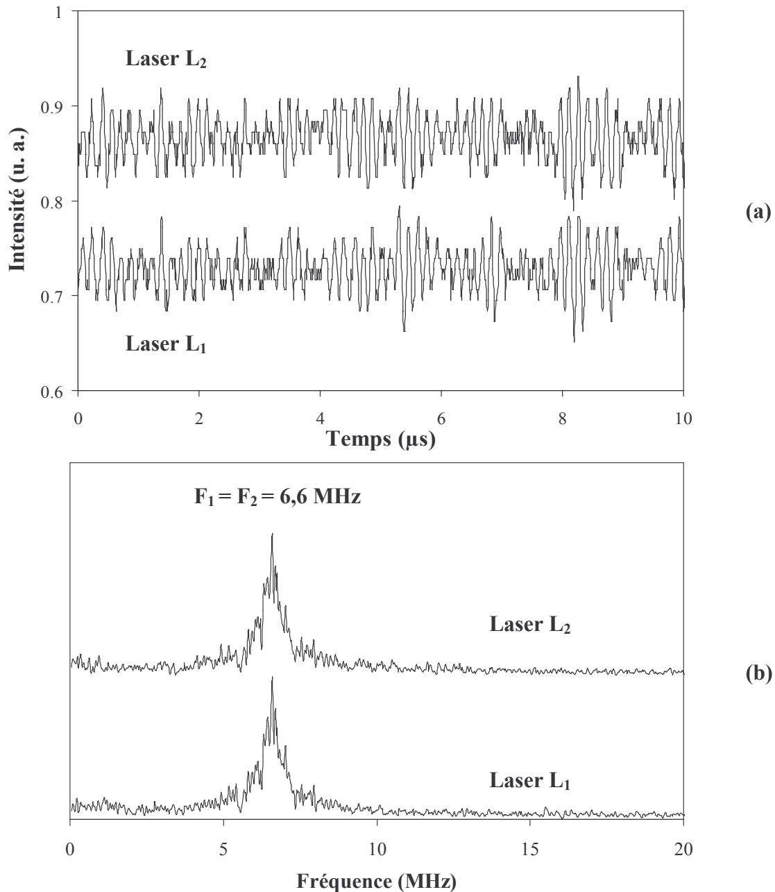
Figure II-5 : Exemple de régimes accrochés a) Evolution temporelle de l'intensité émise par chaque laser et b) spectres basse fréquence associés. Mêmes conditions expérimentales que la Figure II-3.
