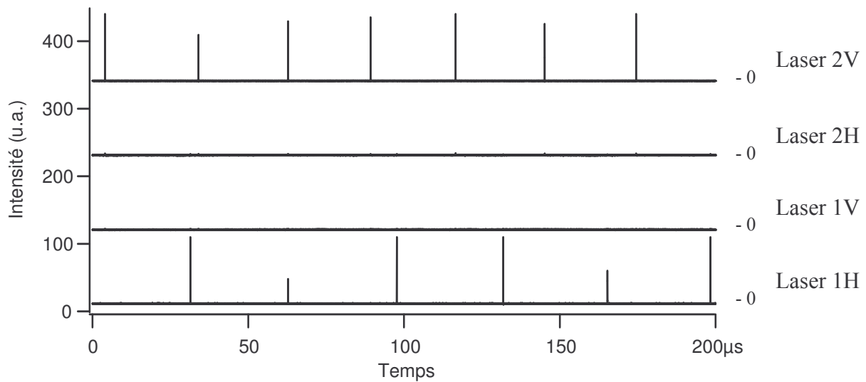
Figure III–14 : Intensité émise pour chaque laser dans les deux directions de polarisations perpendiculaires H et V lorsque les lasers ne sont pas synchronisés.
