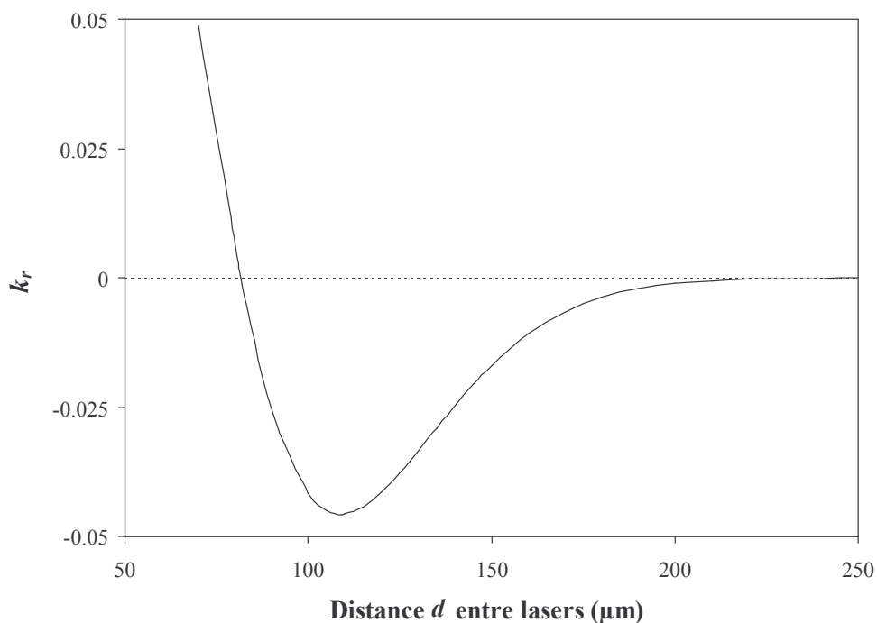
Figure II-26 : Illustration du changement de signe de k_r avec la distance ( w_L = 54,5 \mu\text{m} et w_P = 50 \mu\text{m} ).
