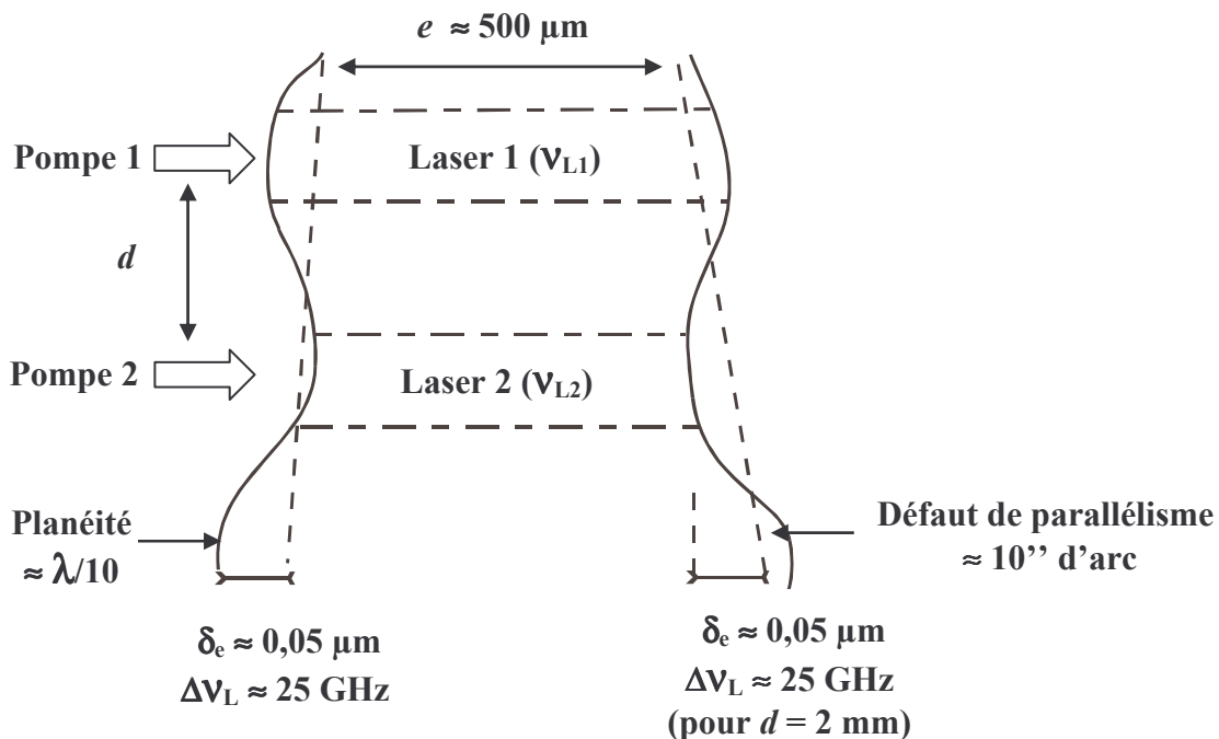
Figure I-2 : Représentation schématique de l'influence des défauts de surface sur les fréquences émises. Pour deux positions différentes sur le cristal, les lasers n'ont pas la même fréquence optique à cause des défauts de planéité et de parallélisme.
