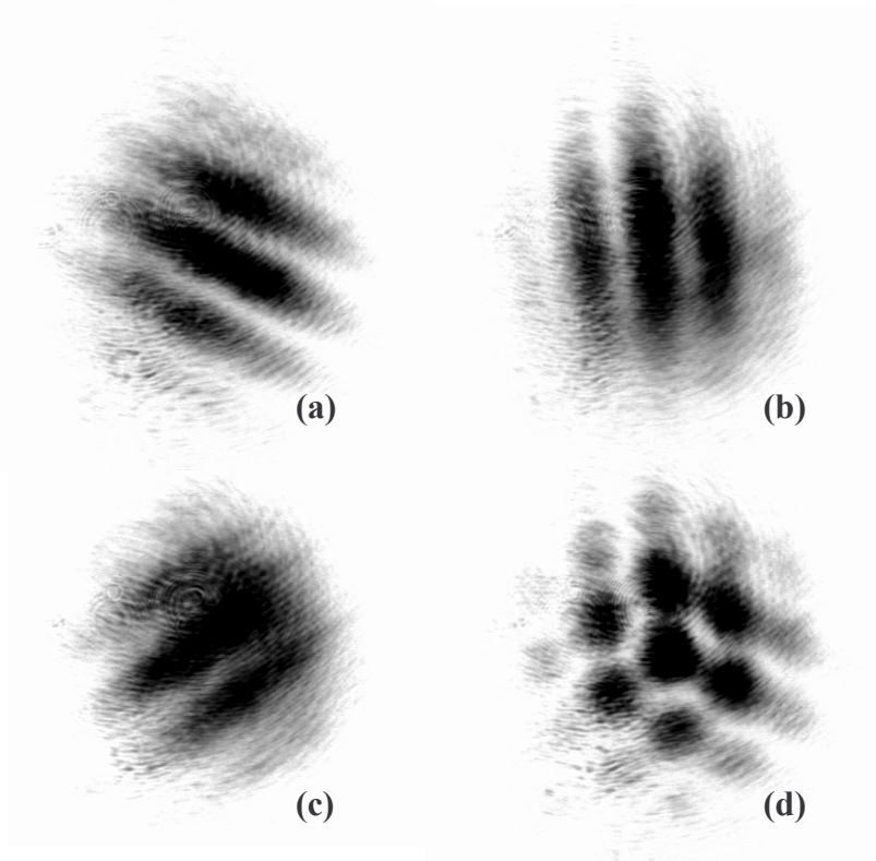
Figure II-28 : Structure du rayonnement en champ lointain dans le cas de trois lasers ( L_1 , L_2 et L_3 ) situés aux sommets d'un triangle équilatéral. Accrochage de deux des trois lasers, a : L_1 , et L_2 ; b : L_2 , et L_3 ; c : L_1 , et L_3 . d : accrochage simultané des trois lasers.
