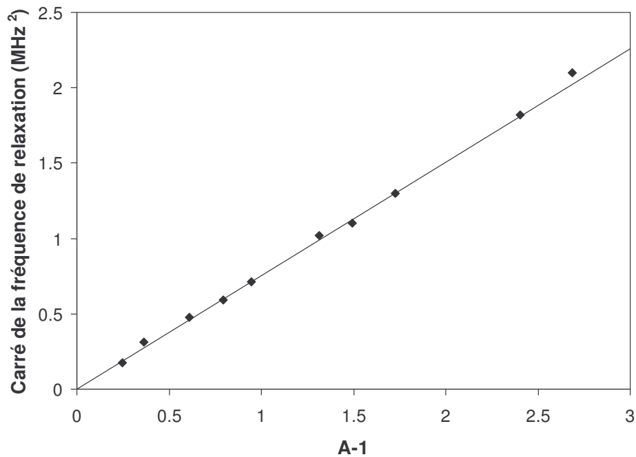
Figure I-13 : Evolution du carré de la fréquence de relaxation en fonction de l'excès de pompage pour le microlaser Nd^{3+} :YAG . Les losanges représentent les résultats expérimentaux alors que la courbe en trait plein est la droite d'ajustement.
