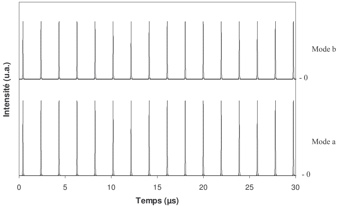
Figure III-12 : Exemple de régime impulsionnel observé selon les modes propres de la cavité pour un désaccord \kappa \Delta / 2\pi = 10 MHz, \Psi_p = 40^\circ et P_p / P_{ps} = 4 .
