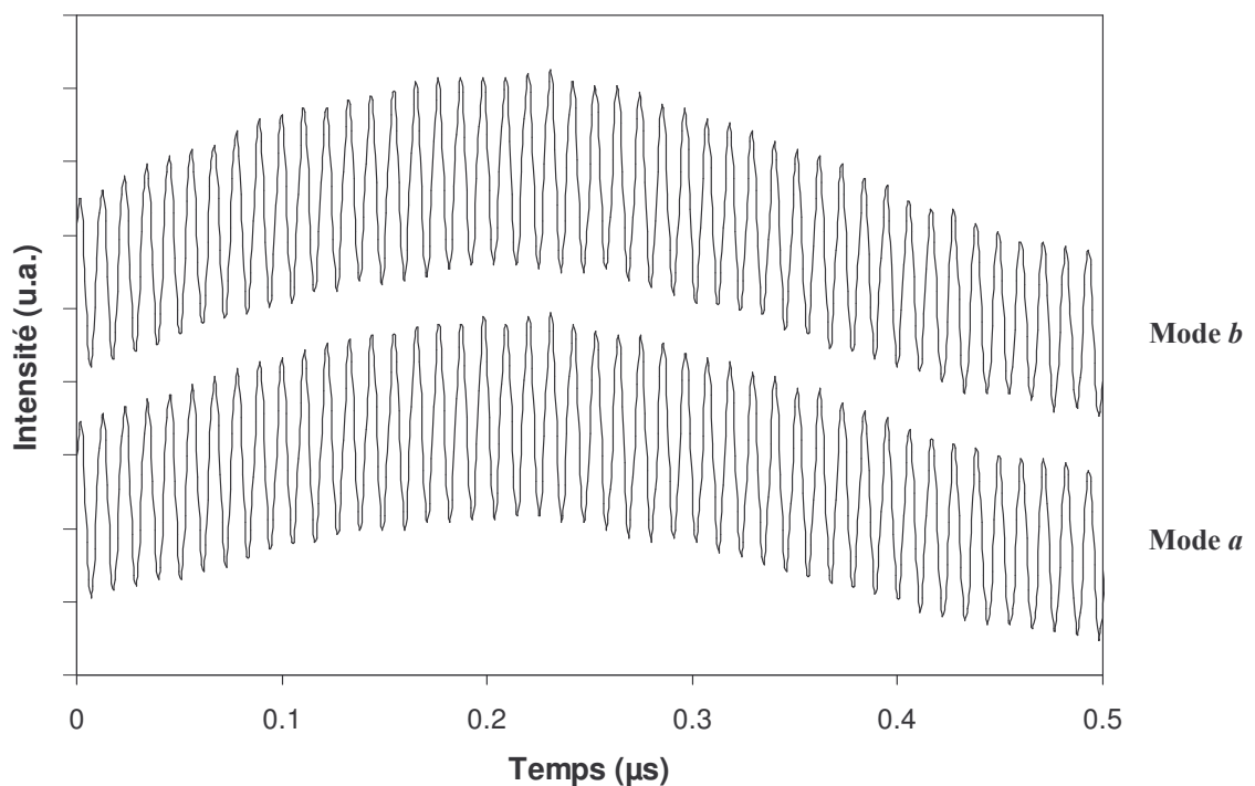
Figure III-5 : Exemple de modulation en phase des intensités de chaque mode à la fréquence du désaccord ici égale à 92 MHz
