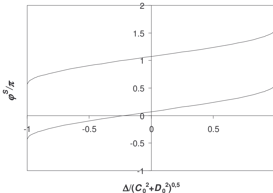
Figure II-12 : Evolution de la phase stationnaire entre les deux lasers en fonction du désaccord. La courbe supérieure est obtenue pour k_r/k_i = 0,8 , E_2^0 = 1,2E_1^0 et k_r < 0 alors que la courbe inférieure est obtenue pour les mêmes paramètres sauf k_r > 0 .
