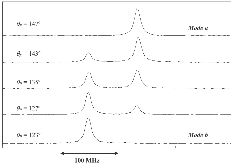
Figure III-4 : Evolution du spectre optique pour différentes valeurs de \theta_p ( P_p/P_{ps} \approx 1,4 ; désaccord entre modes \approx 85 MHz).
