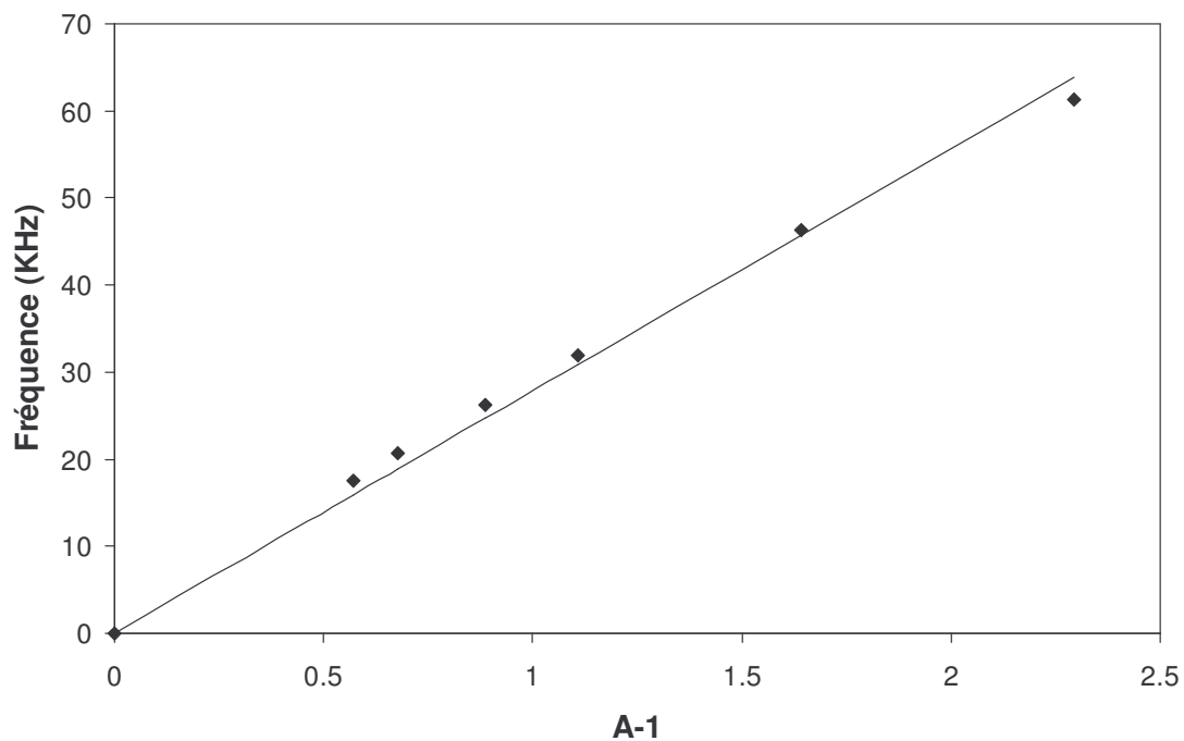
Figure I-16 : Evolution de la fréquence de répétition en fonction de l'excès de pompage.
