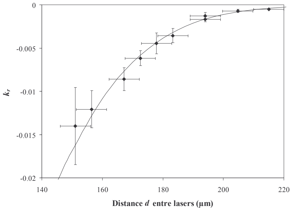
Figure II-25 : Evolution de la partie réelle du coefficient de couplage en fonction de la distance d entre les lasers. \blacklozenge : valeurs expérimentales ; trait continu : valeurs données par l'expression (II-29) avec w_L = 54,5 \mu\text{m} et w_P = 50 \mu\text{m} .
