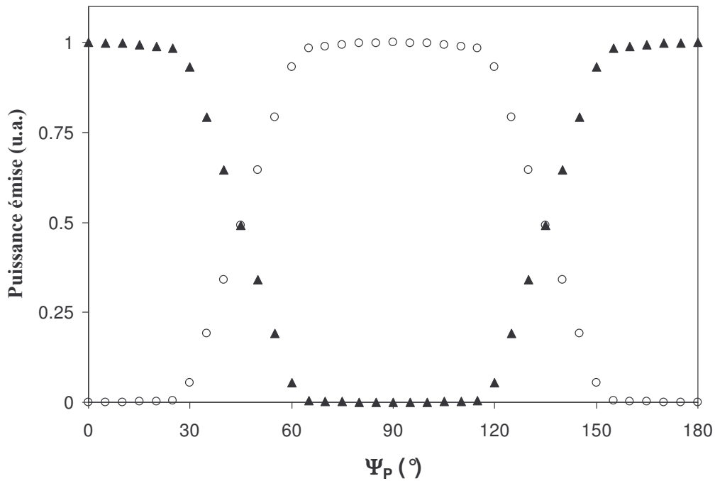
Figure III-10 : Evolution de la puissance émise dans les deux modes propres a (▲) et b (○) de la cavité. \kappa \Delta / 2\pi = 86 MHz, P_p/P_{ps} = 1,4 .
