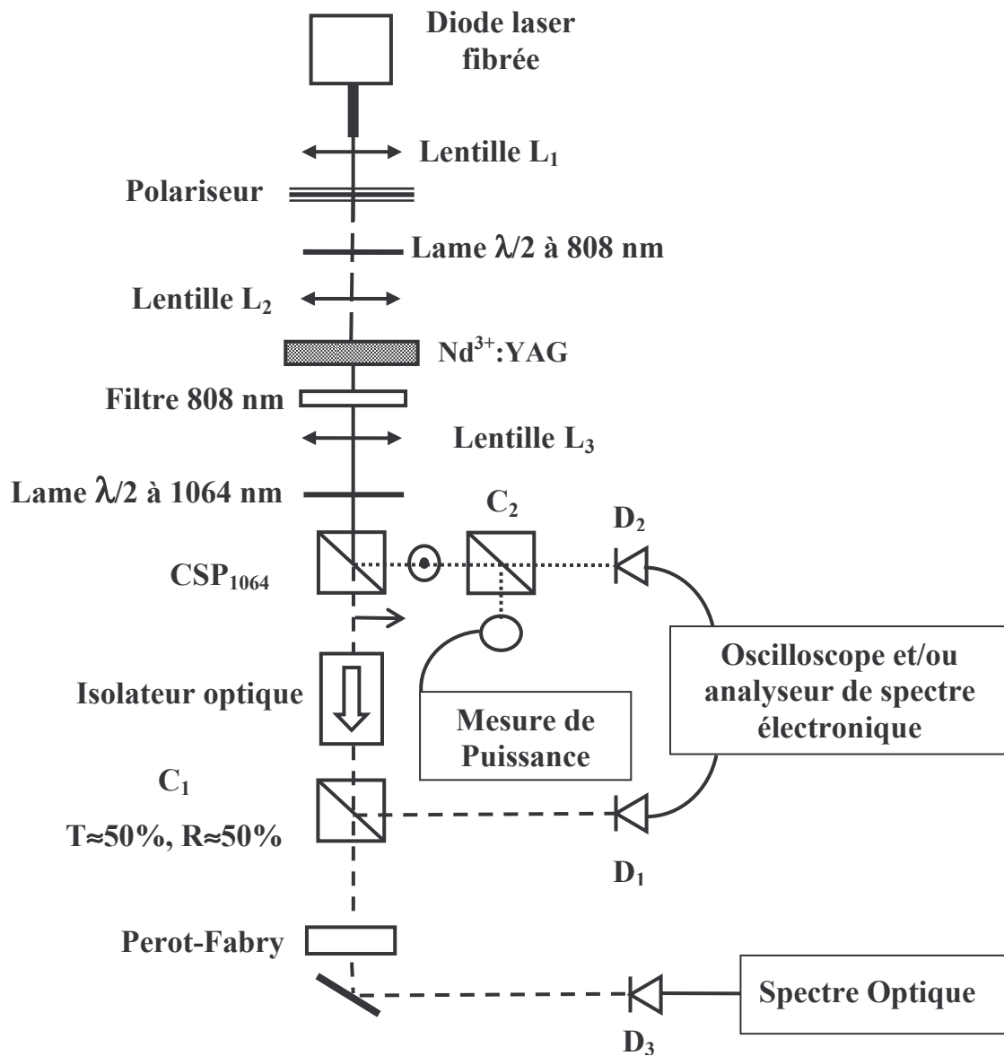
Figure III-1 : Dispositif expérimental permettant l'étude des caractéristiques du rayonnement émis par un Nd 3+ :YAG pompé par un faisceau polarisé
