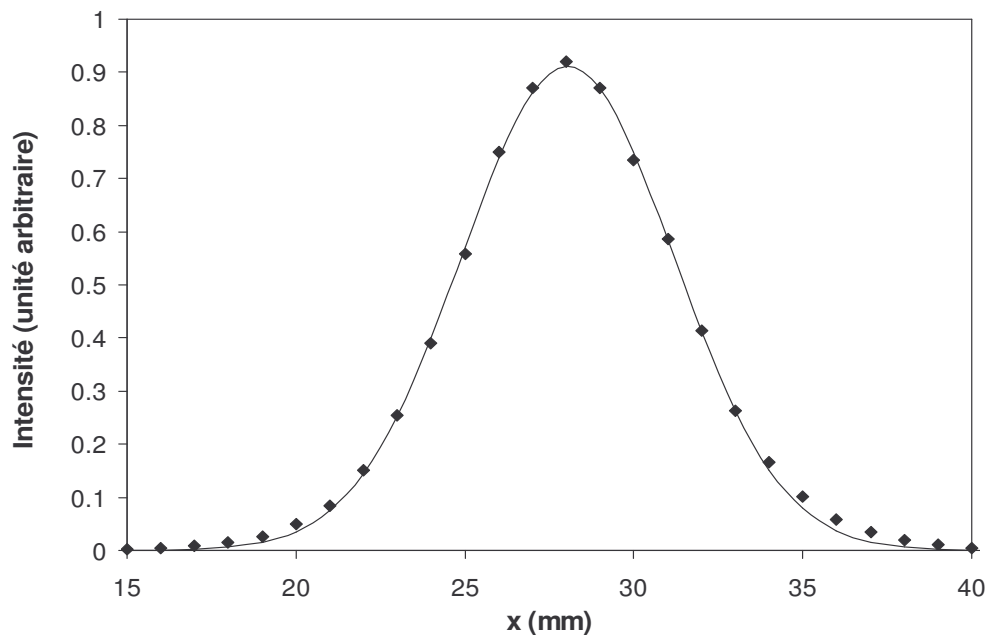
Figure I-7 : Etude du profil transverse du faisceau observé à 90 cm du laser. Les points représentent les valeurs expérimentales, la courbe en trait plein est une gaussienne de largeur 2w=12,6 mm ajustée sur ces points expérimentaux.
