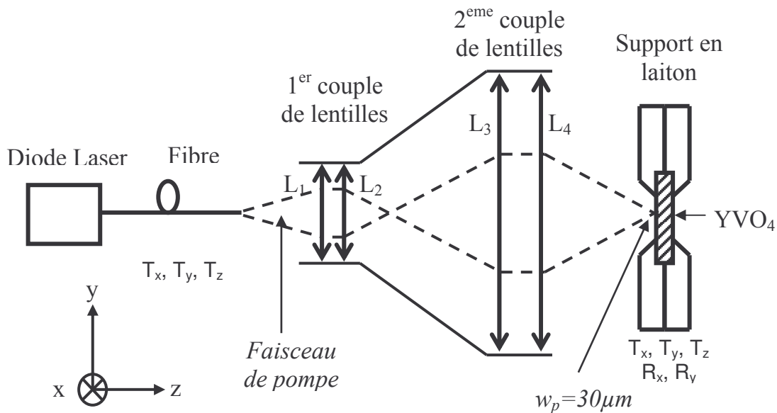
Figure I-4 : Schéma du montage utilisé pour le pompage du microlaser \text{YVO}_4 . L_1 ( L_2 ) est une lentille de focale f_1 ( f_2 ) de 14,5 mm (8 mm) et d'ouverture numérique 0,28 (0,5). L_3 et L_4 sont deux lentilles identiques de diamètre 48 mm et de 120 mm de focale. T_u ( R_u ) symbolise une translation selon l'axe u (rotation autour de u ).
