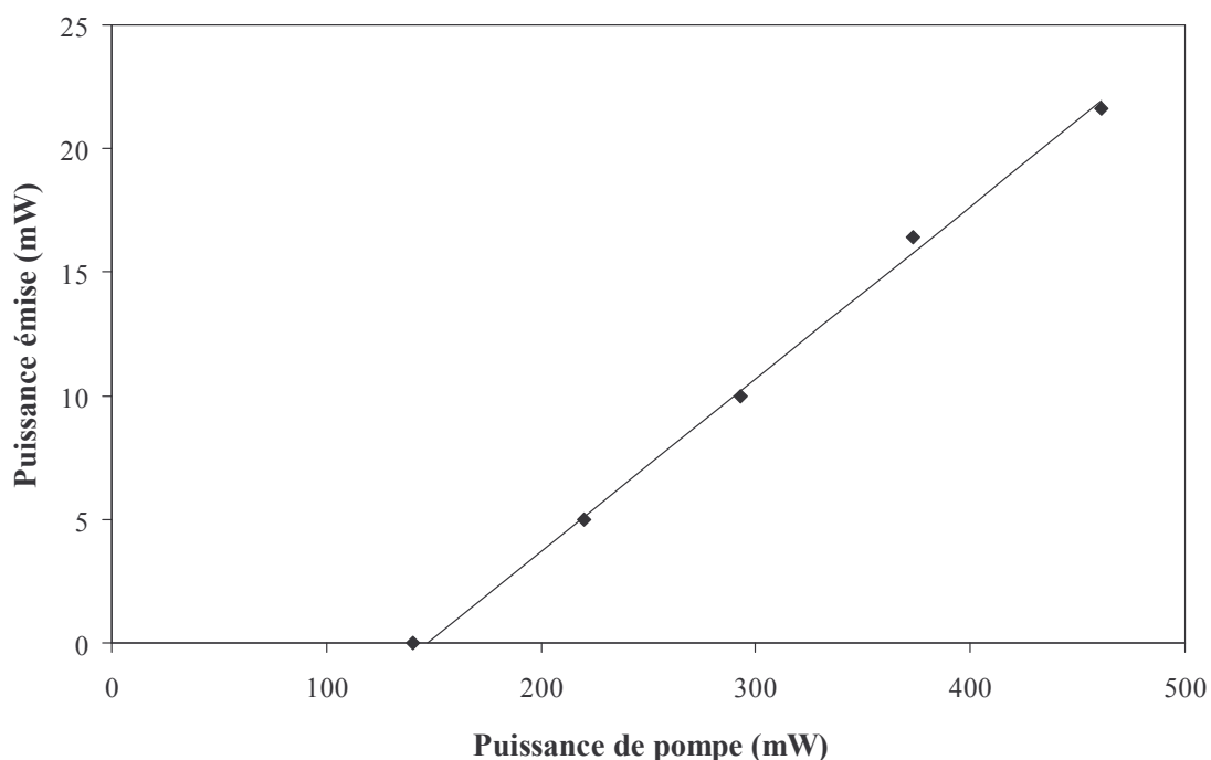
Figure I-15 : Evolution de la puissance émise en fonction de la puissance de pompe.
