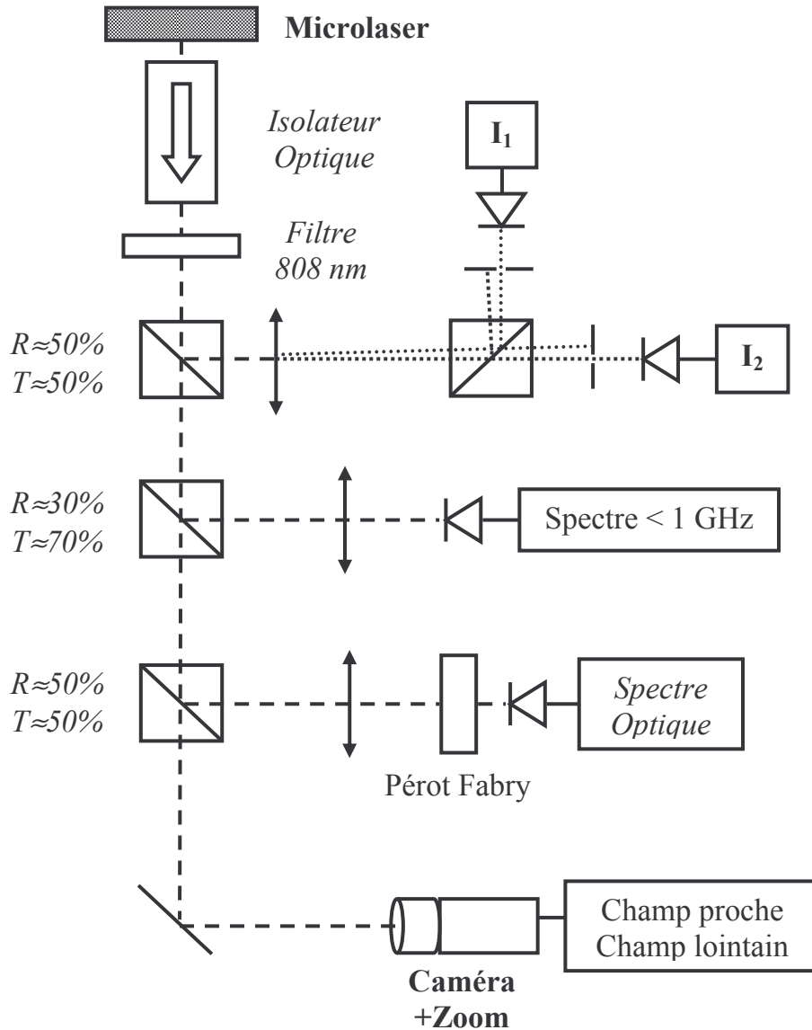
Figure II-2 : Représentation schématique du montage expérimental permettant l'analyse du couplage entre deux microlasers.
