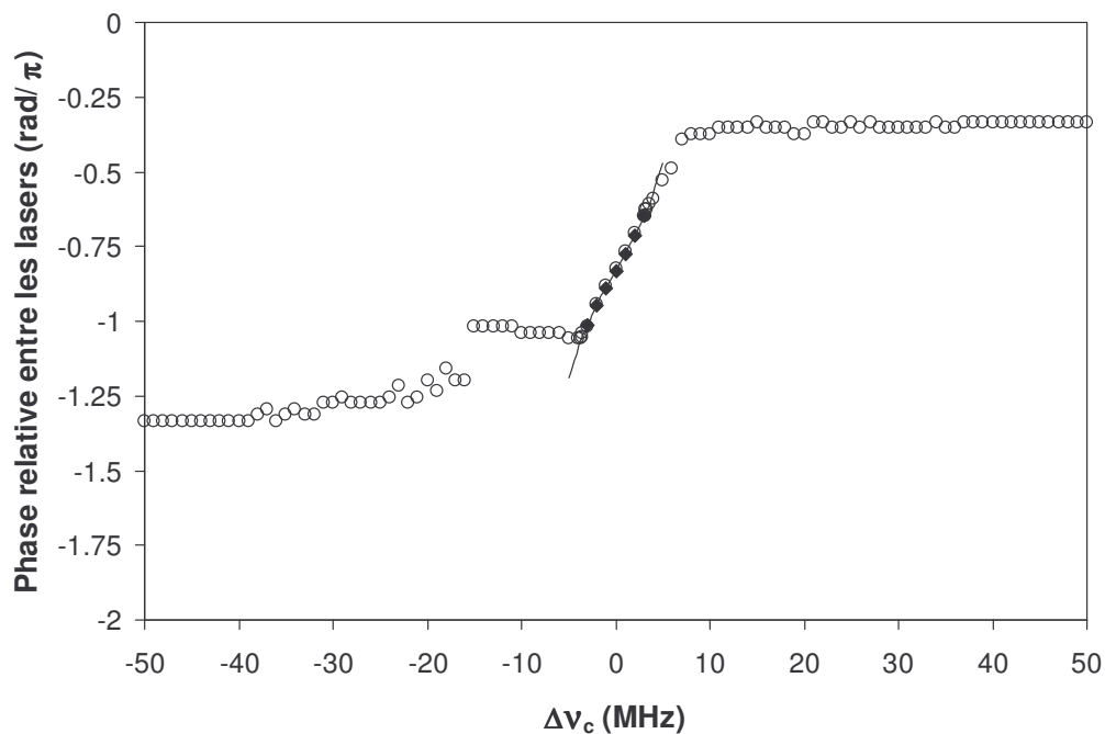
Figure II-18 : Évolution du déphasage moyen entre lasers en fonction du désaccord de fréquence entre cavités (conditions de la Figure II-15).
