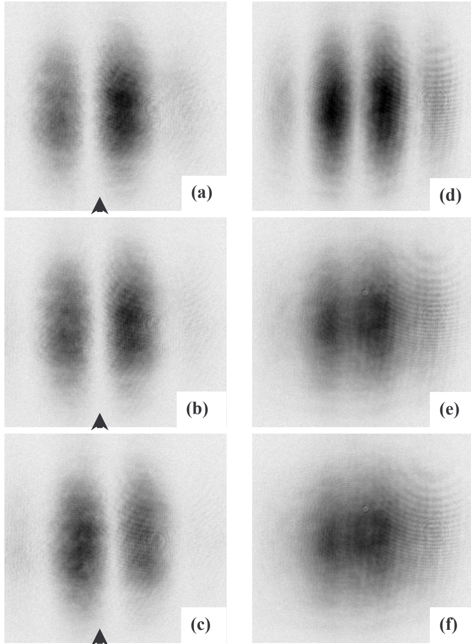
Figure II-9 : Structure du rayonnement en champ lointain pour différents désaccords. a)-c) : lasers accrochés pour d=150 \mu\text{m} , désaccord estimé à -60 \text{ MHz} a), 0 \text{ MHz} b) et 50 \text{ MHz} c). La flèche indique la position de la frange centrale pour un désaccord nul. d)-f) ont été obtenues pour d=194 \mu\text{m} : d) régimes impulsionnels synchronisés (flèche 1 de la Figure II-3), e)-f) ont été obtenus dans le cas de régimes quasi indépendants (flèches 2 et 3 de la Figure II-3).
