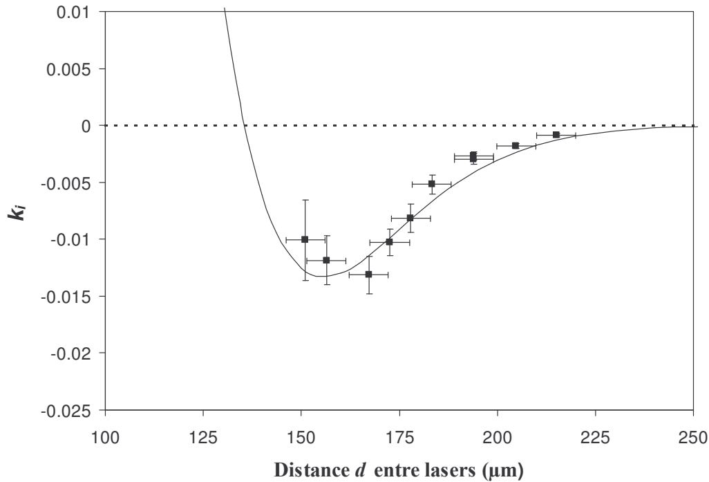
Figure II–27 : Evolution de la partie imaginaire du coefficient de couplage : ■ valeurs mesurées. Trait continu : valeurs calculées ( \Delta T = 33^\circ , w_T = 110 \mu\text{m} , w_L = 54,5 \mu\text{m} )
