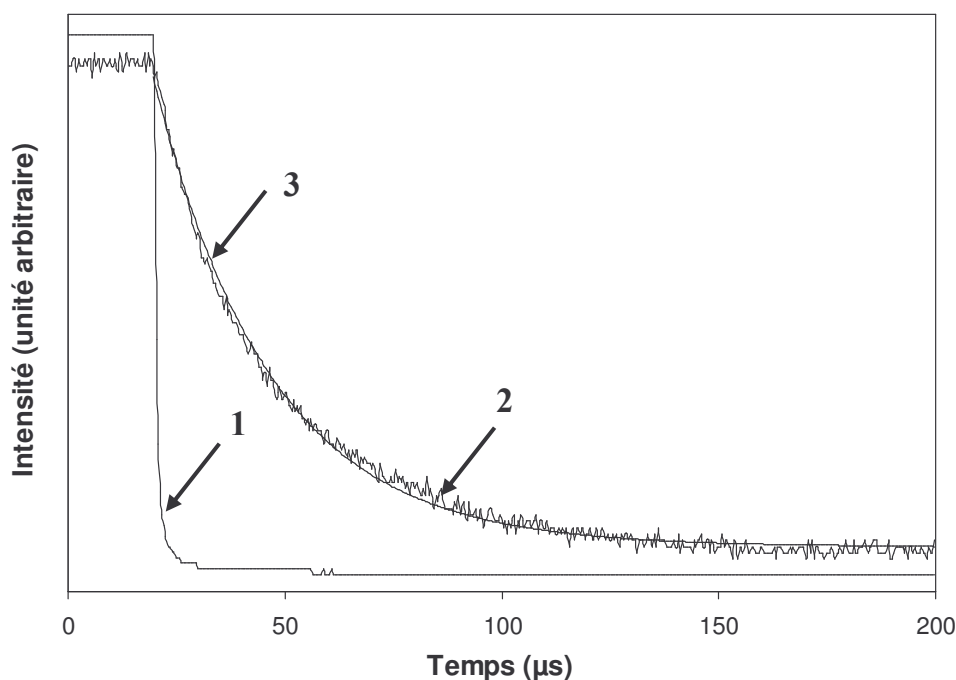
Figure I-5 : Etude de la décroissance de la fluorescence. La courbe 1 (2) représente l'évolution de la puissance de pompe (du signal de fluorescence) en fonction du temps. La courbe 3 est une exponentielle décroissante, ajustée sur la courbe expérimentale 2 dont le temps de décroissance vaut 28\mu\text{s} .
