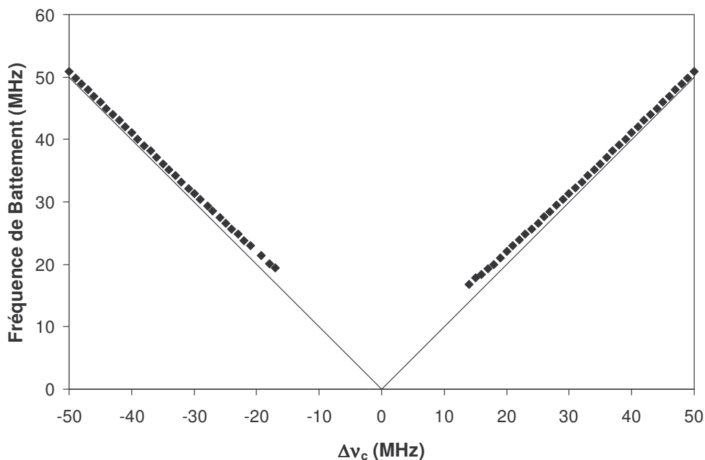
Figure II-16 : Comparaison entre la fréquence de battement (♦) et la valeur absolue du désaccord (trait plein) (conditions de la Figure II-15).
