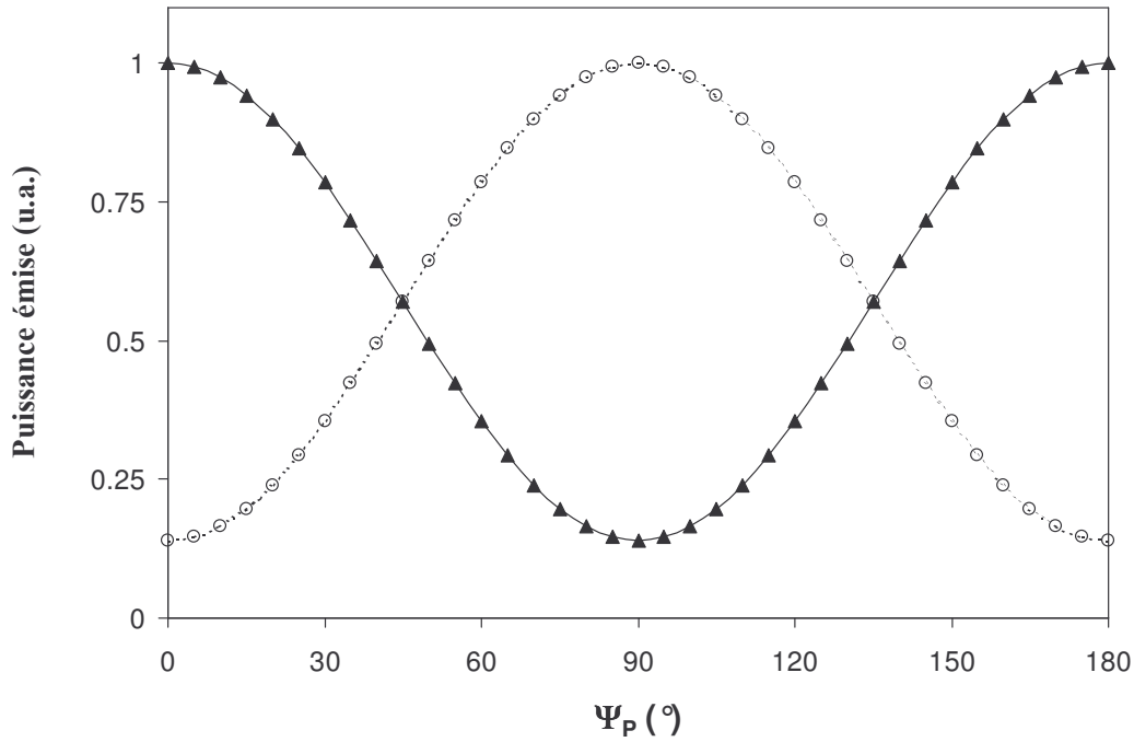
Figure III-9 : Evolution de la puissance émise dans les deux modes propres a (▲) et b (○) de la cavité en fonction de la direction de la polarisation de la pompe. Les courbes en trait plein et en pointillés représentent l'évolution des solutions analytiques données par les équations (III-9-a et b). \kappa \Delta / 2\pi = 86 MHz, P_p/P_{ps} = 2,9
