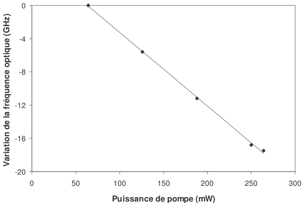
Figure I-11 : Variation de la fréquence optique émise en fonction de la puissance de pompe incidente. Les points représentent les valeurs expérimentales tandis que la courbe en trait plein est une droite ajustée sur les points expérimentaux.
