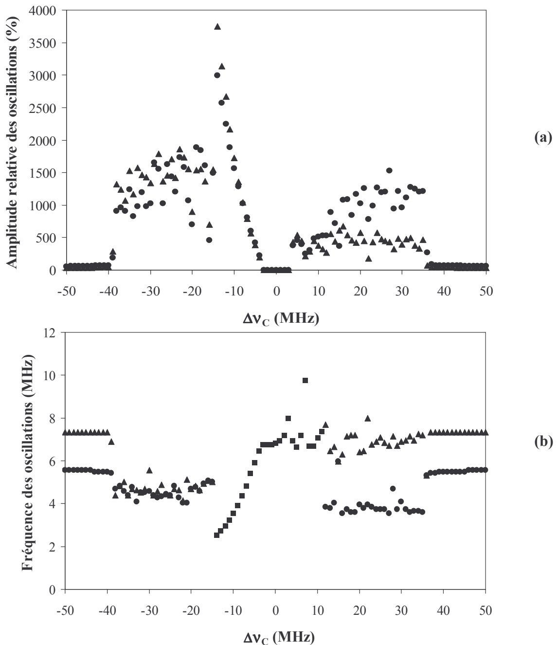
Figure II–15 : Evolution de l'amplitude des oscillations de l'intensité des deux lasers (a), et des fréquences d'oscillation (b) en fonction du désaccord de fréquence entre les cavités.
