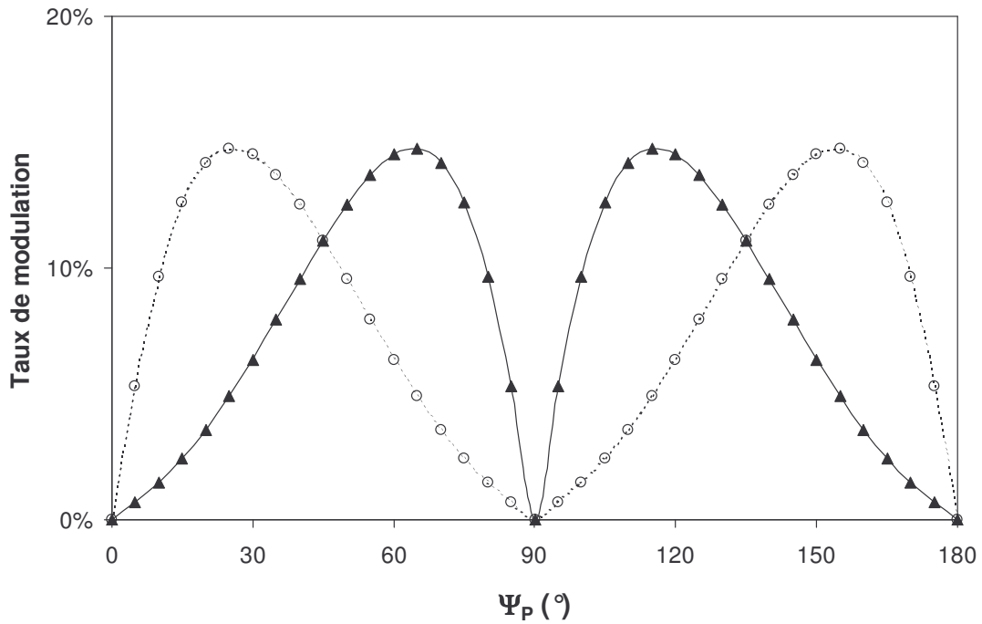
Figure III-11 : Evolution du taux de modulation des modes a (▲) et b (○) à la fréquence du désaccord en fonction de la direction de la polarisation de la pompe. P_p/P_{ps} = 3,8 , \beta_L = 0,69 , \beta_p = 0,81 et \kappa \Delta / 2\pi = 92 MHz
