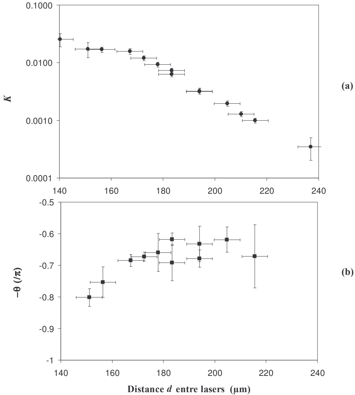
Figure II-13 : Evolution du module K (a) et de l'argument -\theta (b) du coefficient de couplage en fonction de la distance d entre les lasers.
