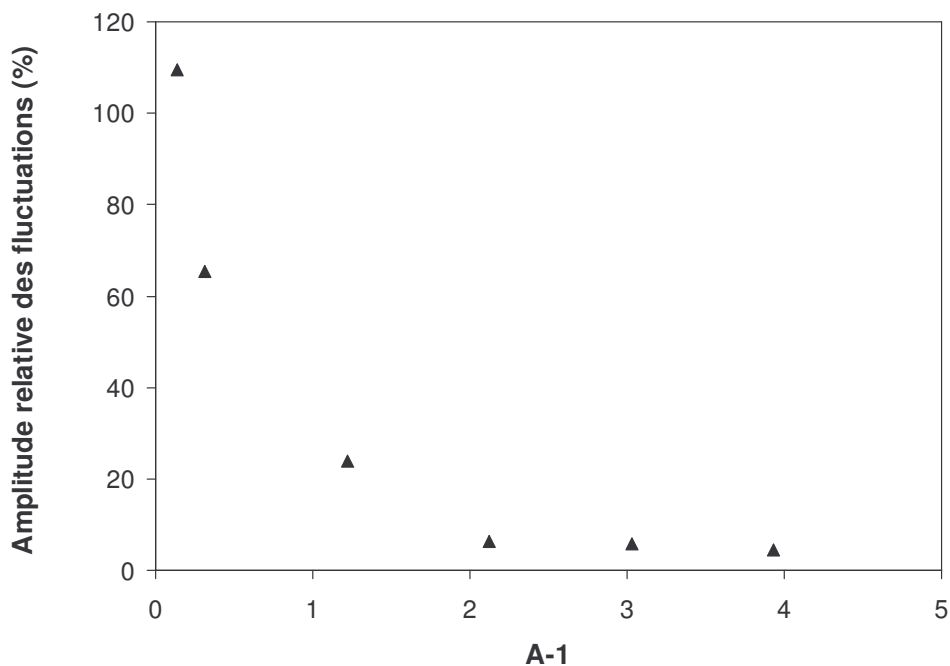
Figure I-9 : Evolution de l'amplitude relative des fluctuations de l'intensité émise en fonction de l'excès de pompage, A-1 .
