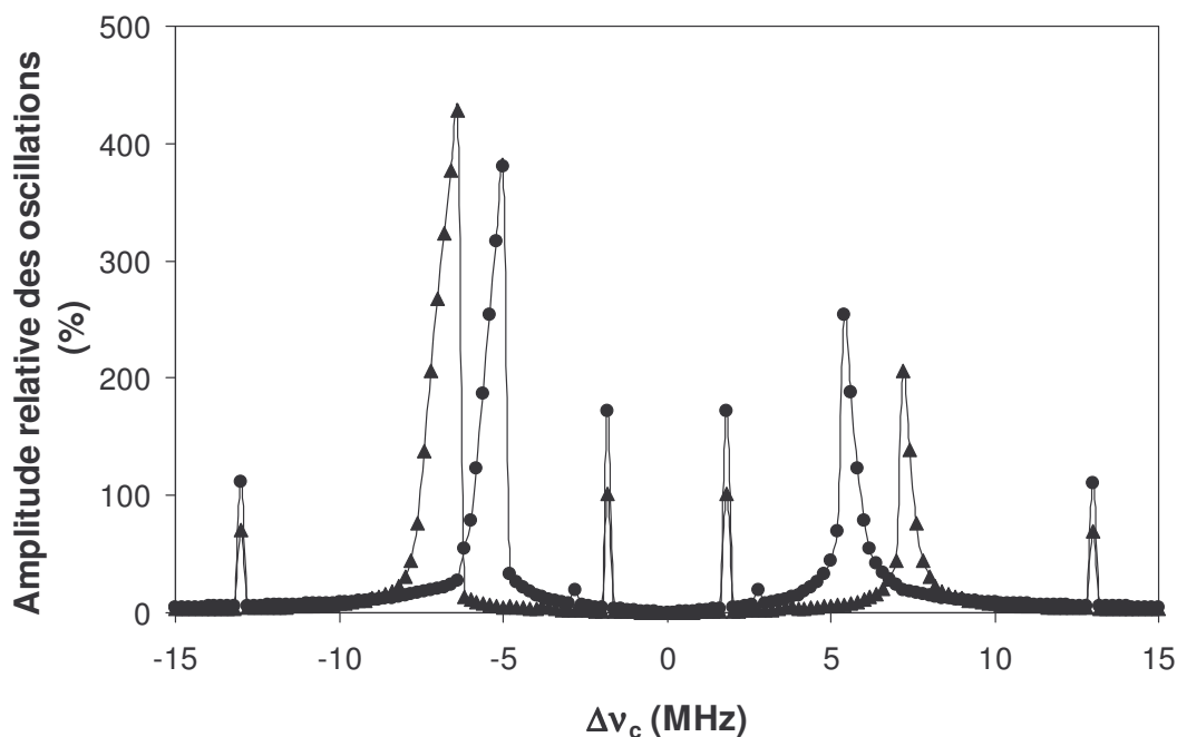
Figure II–23 : Mise en évidence de phénomènes de résonance dans le domaine des lasers quasi indépendants liés aux fréquences de relaxation.
