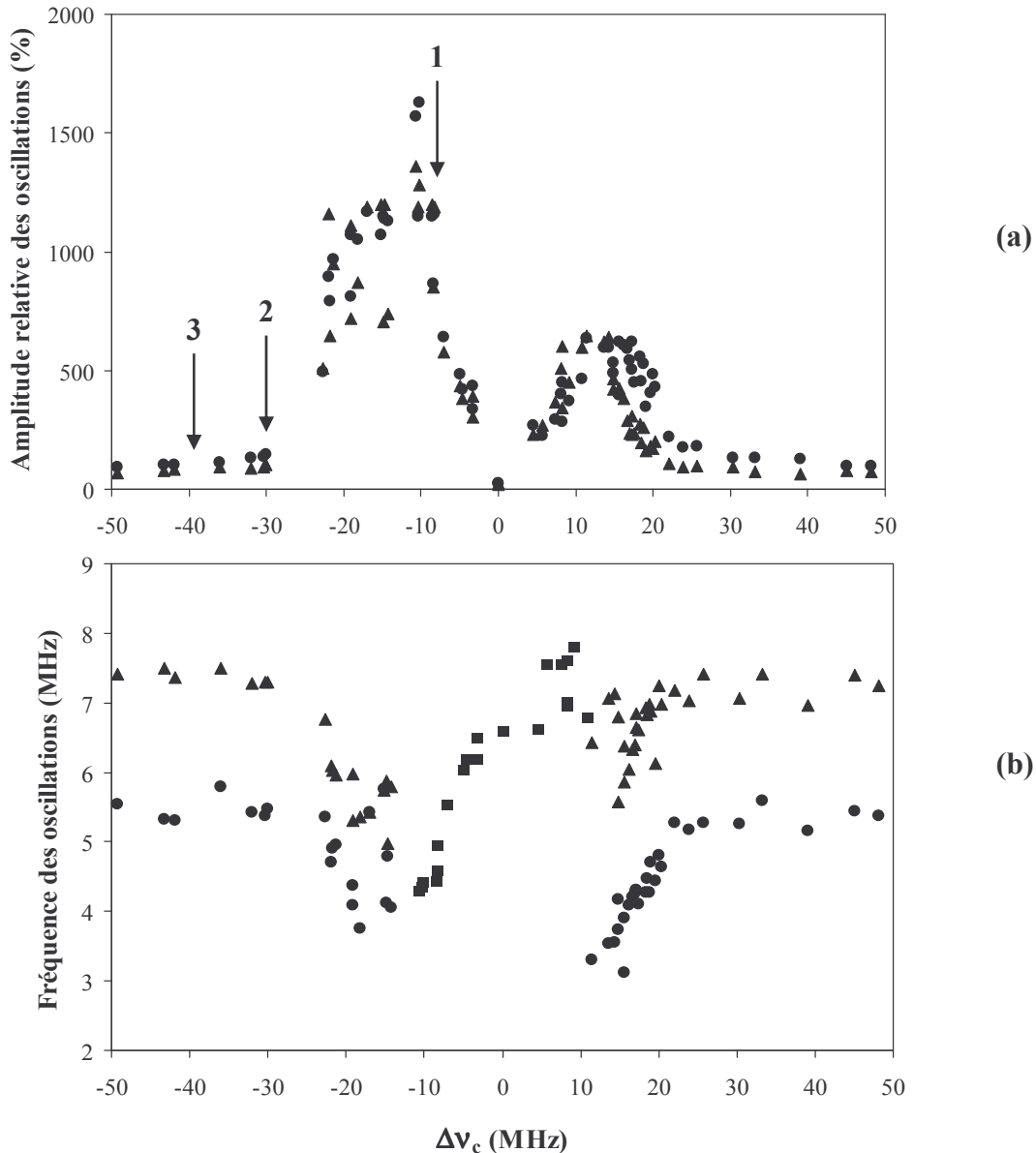
Figure II-3 Evolution en fonction du désaccord de l'amplitude relative crête à crête de l'intensité (a) et du spectre basse fréquence de chacun des deux lasers (b).
