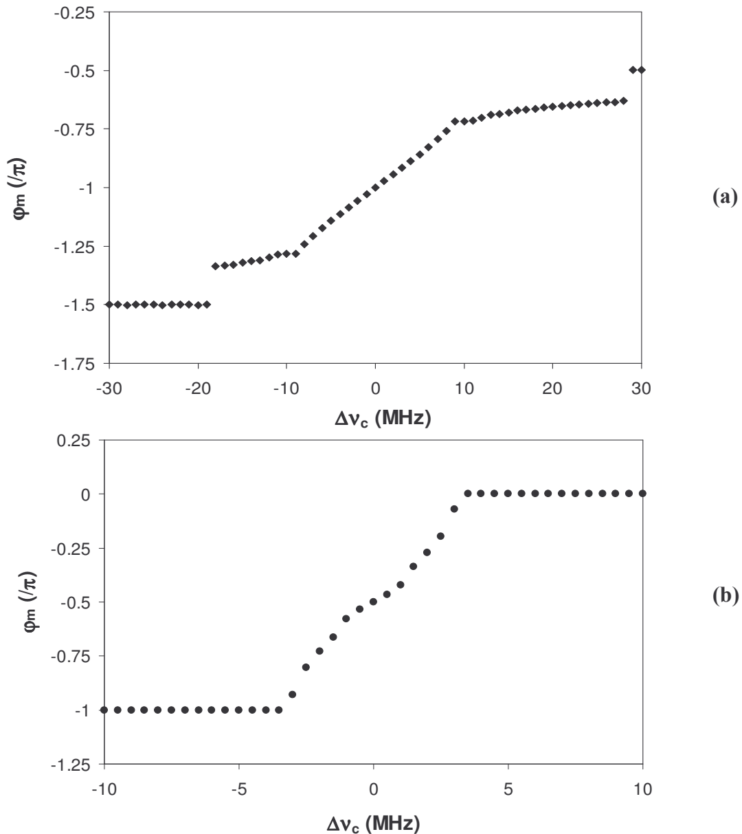
Figure II-22 : Evolution du déphasage au centre de la figure d'interférence en fonction du désaccord des cavités :
