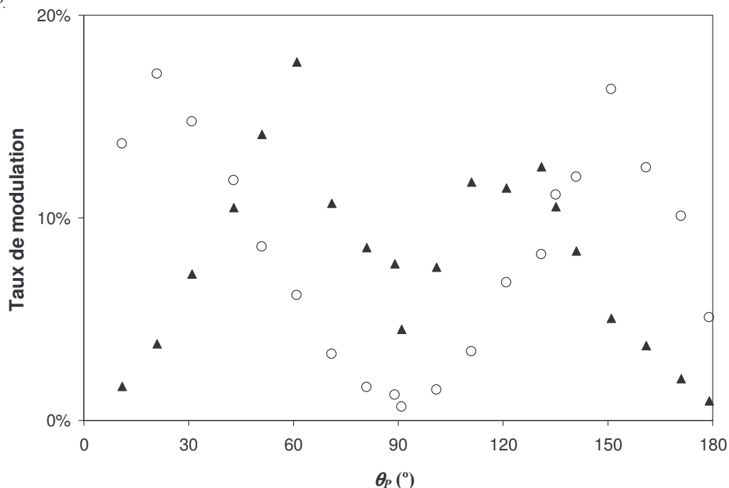
Figure III-6 : Evolution du taux de modulation des modes a (▲) et b (○) à la fréquence du désaccord (92 MHz) en fonction de la direction de la polarisation de la pompe. Même conditions que la Figure III-5.
