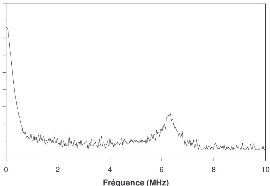
Figure I-8 : Exemple de spectre des fluctuations de l'intensité émise (10 dB/div).
