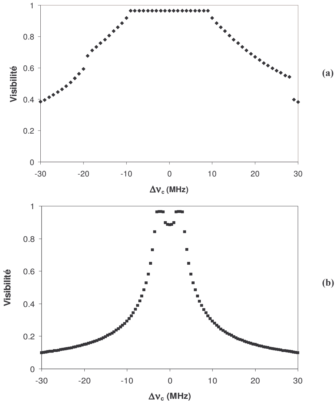
Figure II-21 : Evolution de la visibilité des franges en fonction du désaccord entre cavités : (a) couplage réel, (b) couplage imaginaire (conditions de la Figure II-19).
