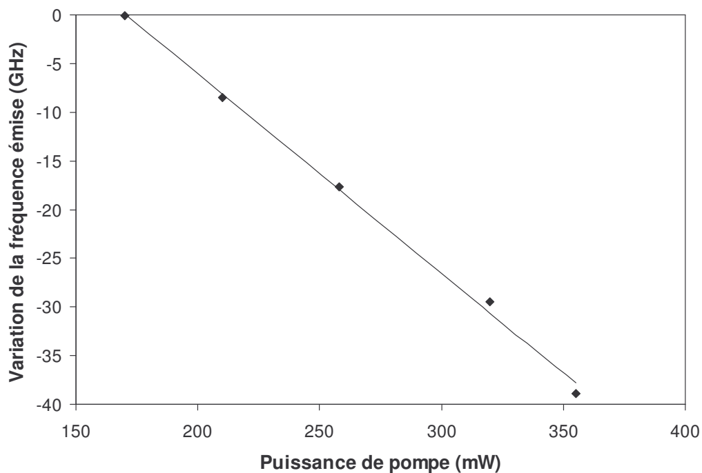
Figure I-17 : Evolution de la fréquence optique du rayonnement en fonction de la puissance de pompe. La courbe en trait plein est une droite de pente 205 \text{ MHz/mW} ajustée sur les points expérimentaux.
