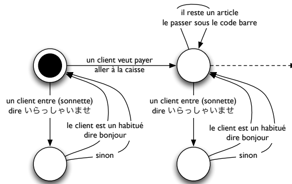
FIG. 6.11 : Modélisation "Mealy" des interactions de l'employé du comбини
