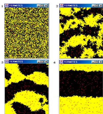
FIG. 2.1: 4 étapes du rassemblement des jetons par les agents “termite”
