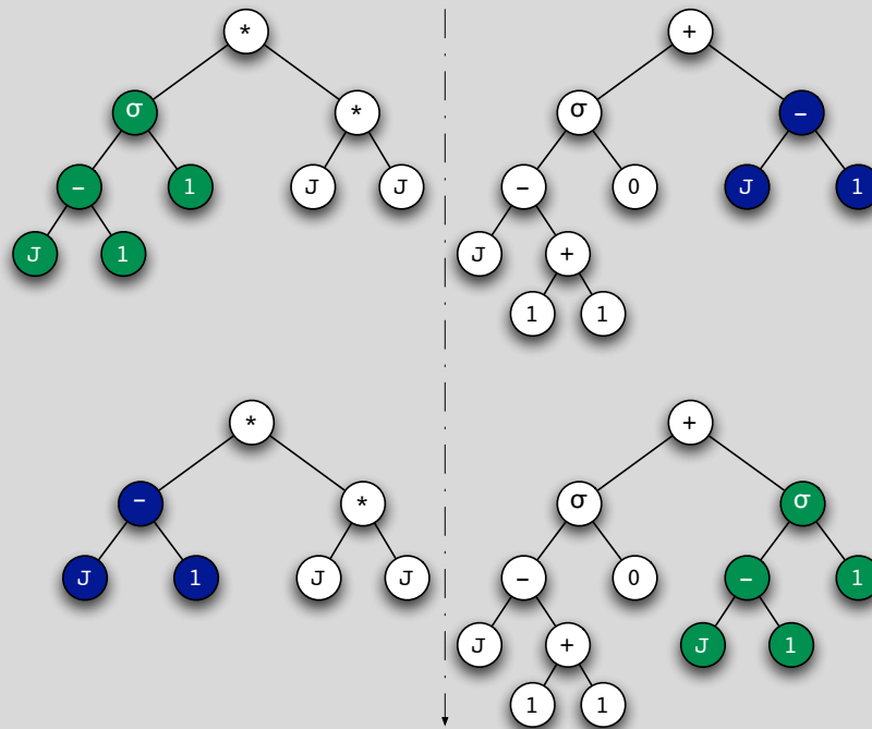
Croisement dans la programmation génétique (d'après Koza [1989])
