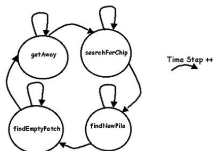
FIG. 2.2: Automate représentant le fonctionnement d'un agent "termite"
