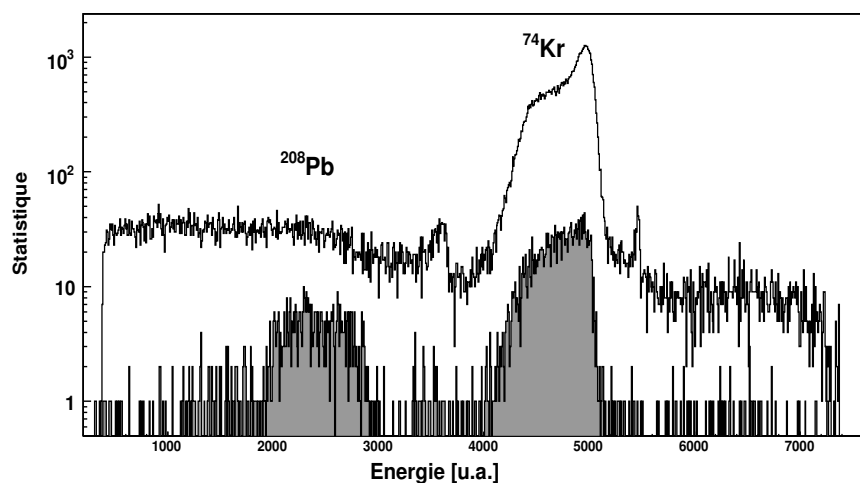
Figure 5.1 Spectre en énergie du premier anneau de silicium en coïncidence (spectre plein) ou non (spectre vide) avec un \gamma dans EXOGAM.
