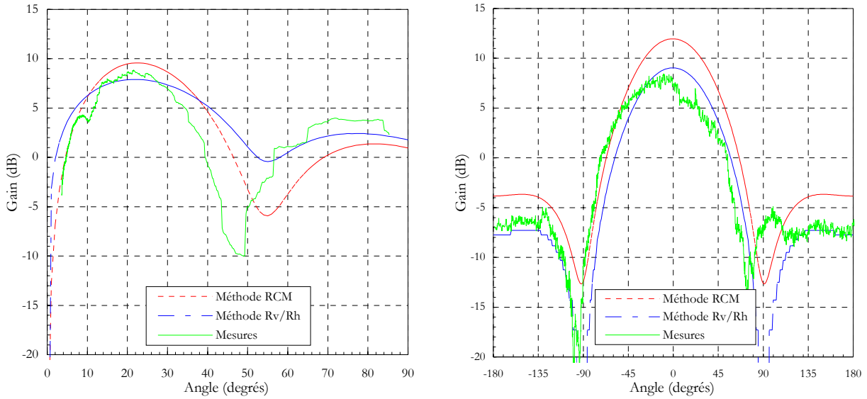
a) diagramme en élévation, azimut = 0°.
