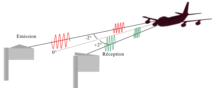
FIG. 4.7 - Principe de mesure de l'ONERA pour un azimut de 0°.
