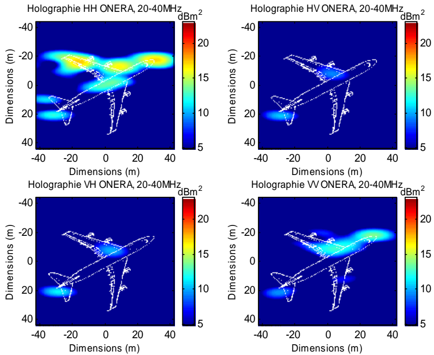
FIG. 4.25 - Holographie sur les données ONERA dans la bande 20-40 MHz, éclaircement autour de 60°.
