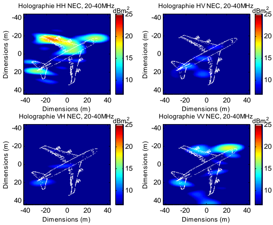
FIG. 4.24 - Holographie sur les données NEC dans la bande 20-40 MHz, éclaircement autour de 60°.
