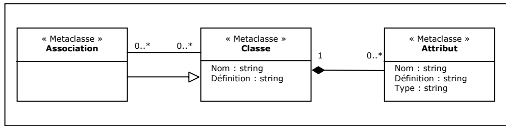
Figure 72. Métaclasse de la BD géographique sur lesquelles s'appuie le modèle des spécifications.
