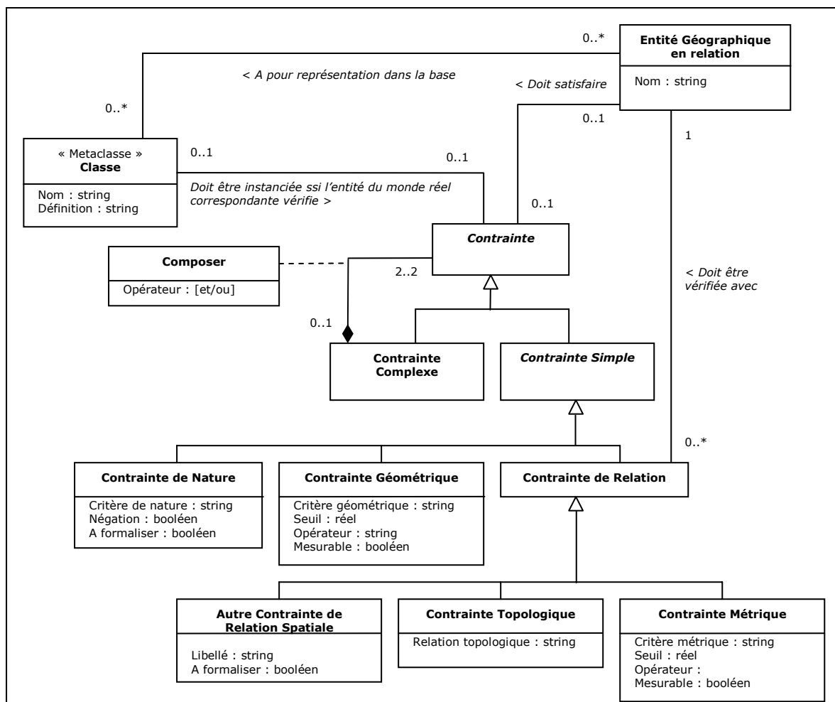
Figure 75. Extrait du modèle des spécifications : les contraintes élémentaires géométriques, de relation et de nature.
