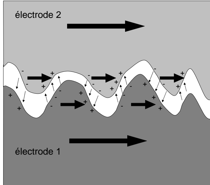
FIG. 5.5 – Représentation schématique (et exagérée!) d'une barrière conduisant à un couplage peau d'orange. La rugosité entraîne l'apparition de masses magnétiques (symbolisées par les signes "+" et "-") de part et d'autre de la barrière. Un couplage dipolaire entre électrodes apparaît donc.
