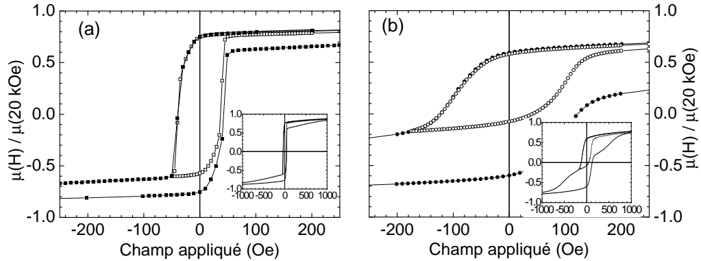
FIG. 6.15 – Cycles d’hystérésis majeurs (symboles pleins) et mineurs (symboles évidés) de tricouches \text{Fe}_3\text{O}_4 ( t nm)/ \gamma\text{-Al}_2\text{O}_3 (5 nm)/ Fe (10 nm). (a) : t = 15 nm le cycle mineur est étroit ( H_c = 40 Oe) et centré. (b) : t = 50 nm le cycle mineur est large ( H_c = 100 Oe) et l’on observe un léger décalage du cycle ( H_d = 5 Oe). Les inserts montre les cycles d’hystérésis aux champs plus élevés.
