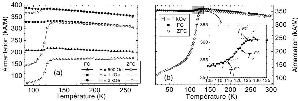
FIG. 4.10 – Courbes M(T) réalisées après refroidissement sous champ (FC) et à champ nul (ZFC) (a) échantillon de 25 nm d'épaisseur, effet du champ appliqué. (b) échantillon de 50 nm d'épaisseur, mesure FC et ZFC par SQUID à partir de 20 K sous 1 kOe. L'insert montre le détail de la courbe FC autour de la température de transition et la définition des températures T_V^{FC} , T_i^{FC} et T_f^{FC} .
