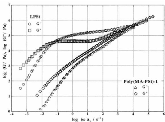
Figure I-8 Tracé de G' et G'' en fonction de \omega pour un PS linéaire de DP_n = 3700 et un PM de \overline{DP}_{n \text{ tronc}} = 400 et \overline{M}_{w \text{ branche}} = 3450 \text{ g.mol}^{-1} à T_{\text{ref}} = 160^\circ\text{C}
