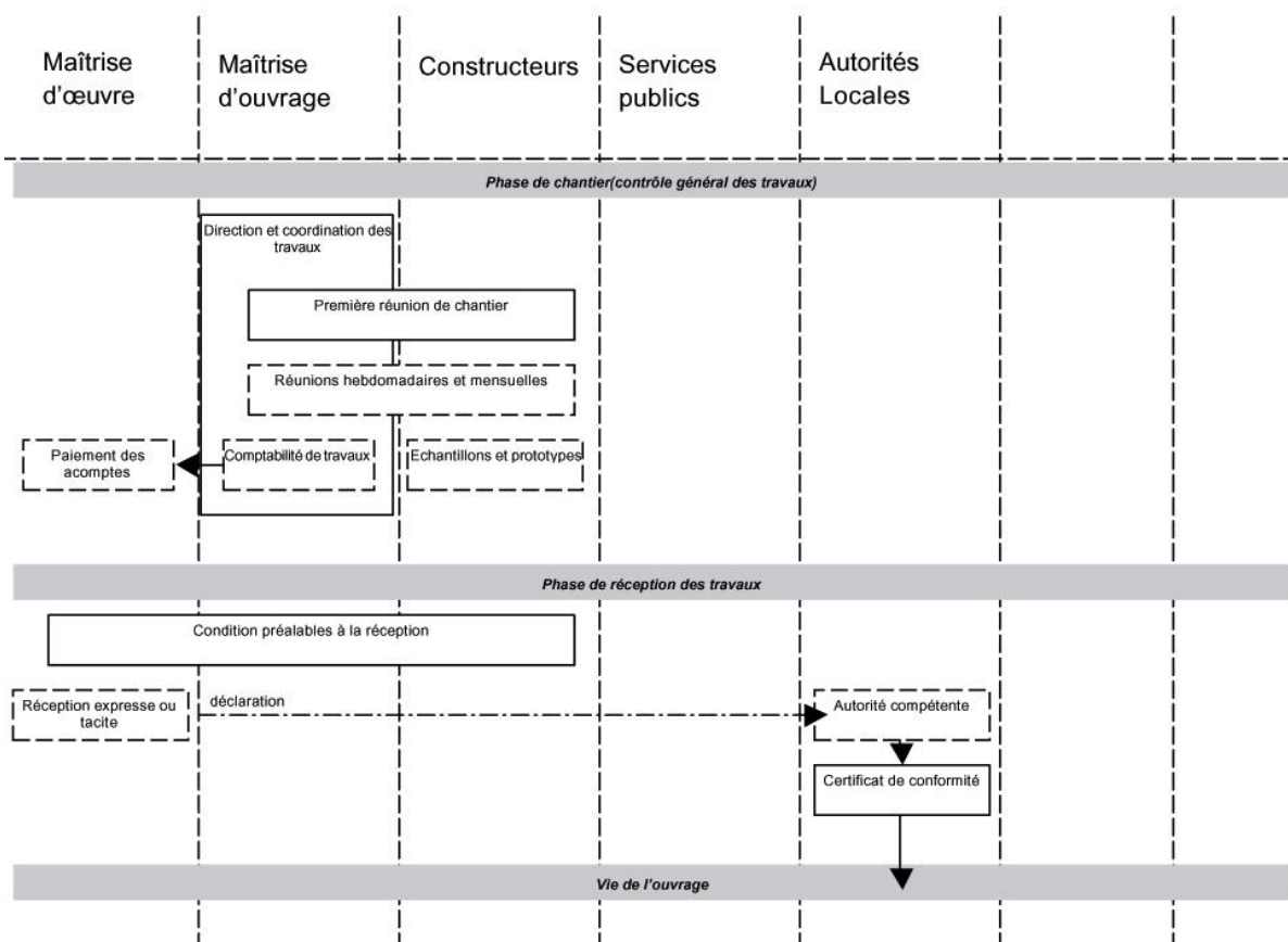
Figure 91 : Etape de chantier (2).
