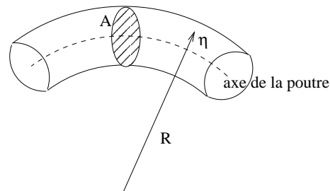
Fig. B.2 — Poutre en flexion.
