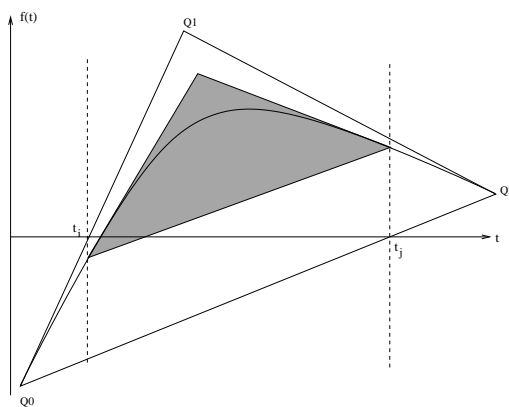
Fig. 1.5 — Calcul du zéro d'une courbe de Bézier quadratique : les segments à gauche de t - i et à droite de t_j sont éliminés. La partie contenue dans l'enveloppe grise est conservée pour l'itération suivante.
