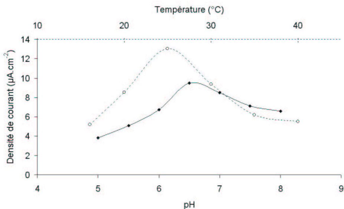
Figure IV.11. Influence de la température (-----) [pH de travail = 6,5] et du pH (—) [température de travail = 25°C] sur la réponse en densité de courant d'une électrode PEDT/PPO met A. Conditions opératoires : 5 \mu\text{M} catéchol, solution tampon phosphate 0,1 M contenant 0,1 M KCl, -0,2 V/ECS, système sous agitation.
