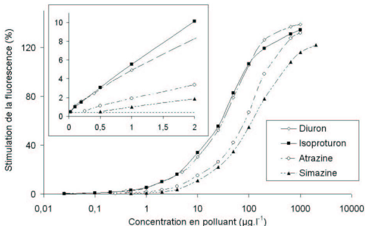
Figure III.22. Courbes de doses-réponses des herbicides anti-PSII. Agrandissement : réponse aux polluants pour des concentrations proches du ppb, (----) limite de détection. Conditions : tampon phosphate (10 mM ; pH 7), 20°C, débit = 2 ml.min -1 .
