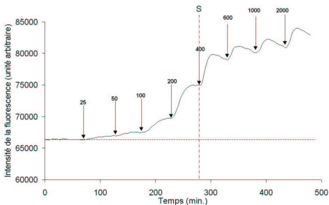
Figure III.25. Réponse du biocapteur à des doses cumulées d'ioxynil ( \mu\text{g.l}^{-1} ). Le seuil S délimite le changement de comportement du biocapteur. (----) Niveau de base de la fluorescence. Conditions : tampon phosphate (10 mM ; pH 7), 20°C, débit = 2 ml.min -1 .
