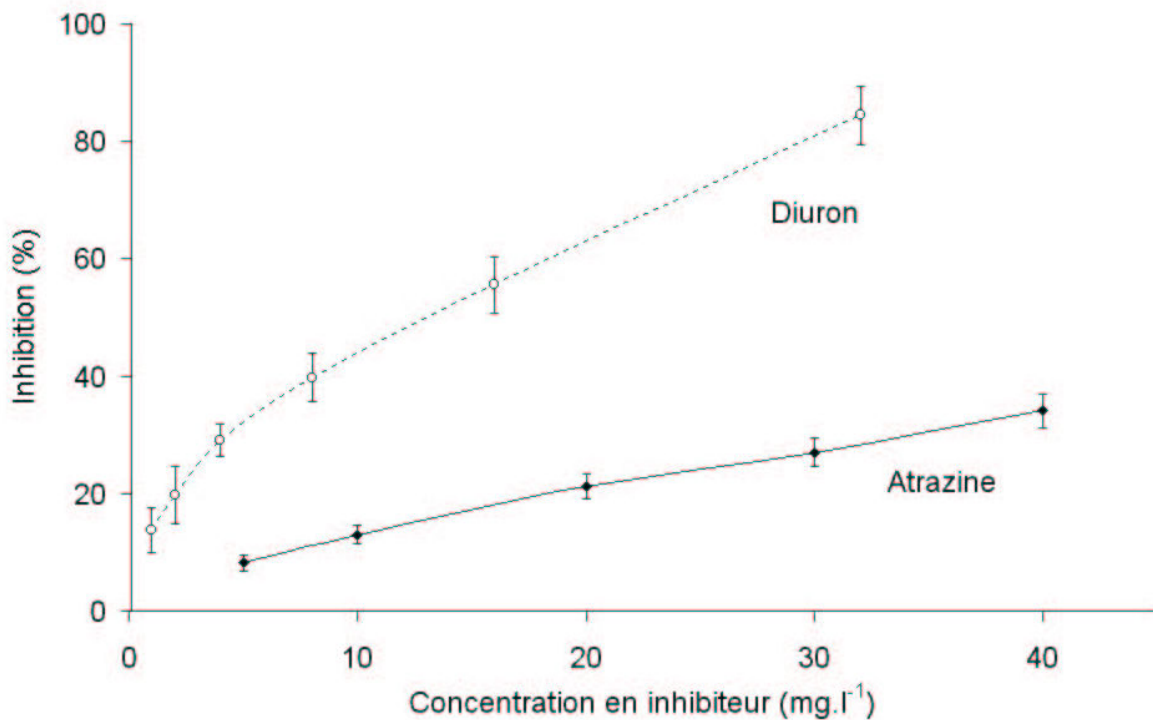
Figure IV.19. Courbes de doses-réponses de l'atrazine et du diuron obtenues par inhibition de l'électrode PEDT/PPO met B en présence de 25 \mu M de dopamine. Conditions opératoires : solution tampon phosphate (0,1 M ; pH 6,5), température 25°C, -0,2 V/ECS, système sous agitation.
