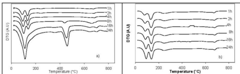
figure 122. Evolution des courbes DTG de a) C 2 et b) C 2 +AM 2
