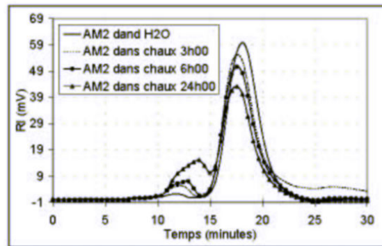
figure 72. Chromatogrammes de AM_2 dispersés dans la chaux
