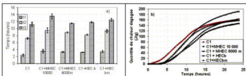
figure 84. Comparaison de l'hydratation des formules "C 1 +éthers de cellulose" : a) temps caractéristiques b) quantité de chaleur dégagée
