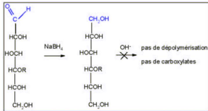
figure 77. Réduction des polysaccharides par \text{NaBH}_4 , R : Chaîne polymérique
