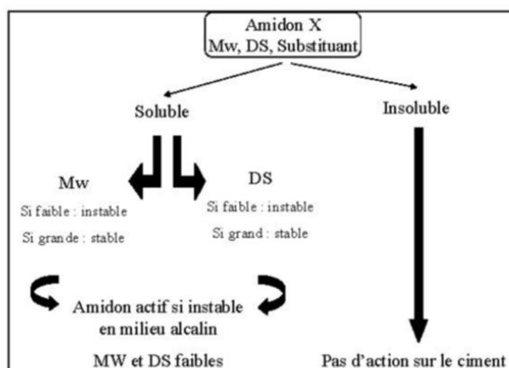
figure 114. Paramètres déterminant l'action de l'amidon sur le ciment
