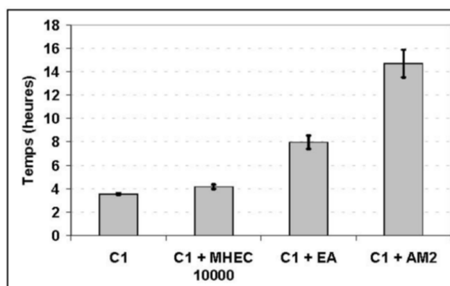
figure 41. Temps correspondant au maximum de la courbe conductimétrique ( t_{max} )
