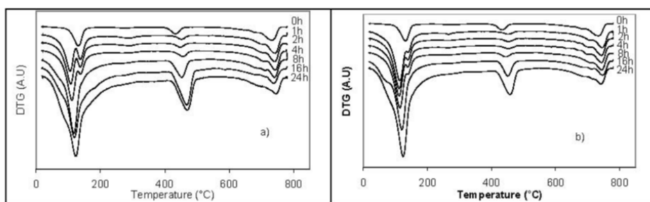
figure 121. Evolution des courbes DTG de a) C 1 +EC et b) C 1 +AM 2
