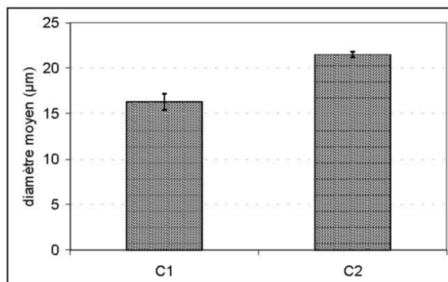
figure 21. Diamètre moyen des ciments C_1 et C_2
