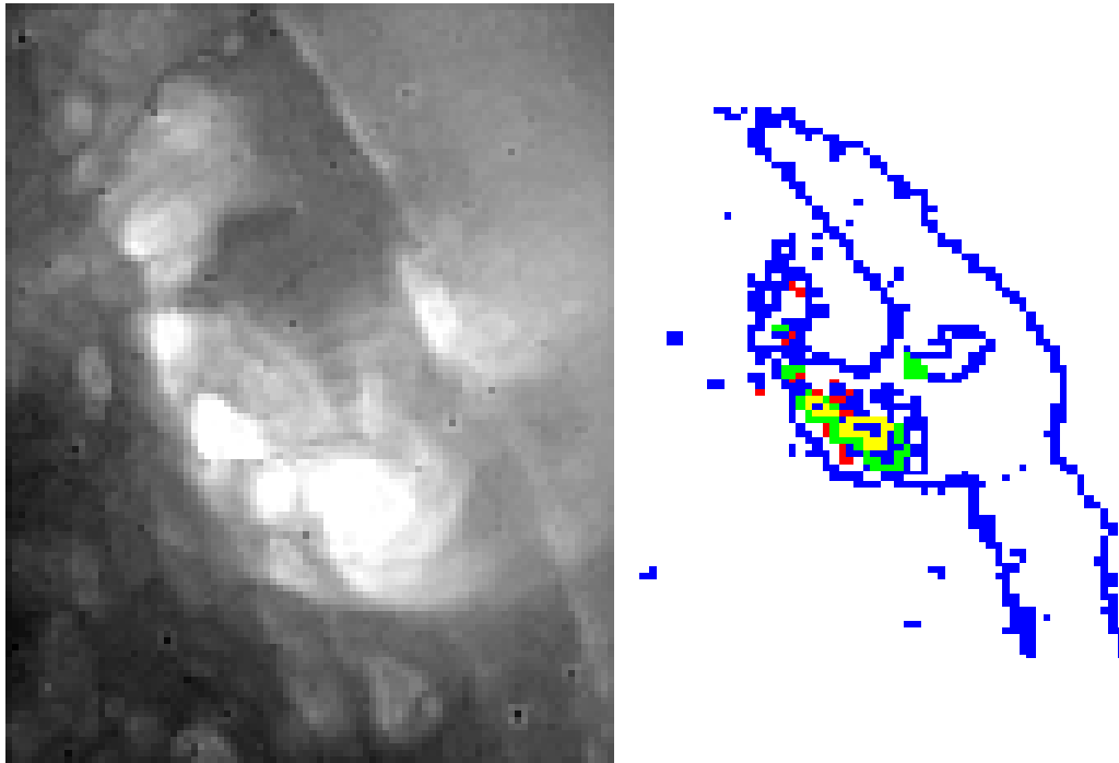
Figure IV.2: SOHO/EIT 08 Aout 1998 : A gauche, une image EIT en Fe XII. A droite : Superposition du contour transverse des boucles à différentes températures. A cause de la position de la région active, on obtient en fait une coupe en tranche en température : Le rouge correspond au contour de la boucle en He II, le bleu en Fe IX/X, le vert en Fe XII, le jaune en Fe XV. On notera que le centre des tubes de flux magnétiques de l'ARL coincide avec les boucles les plus chaudes.
