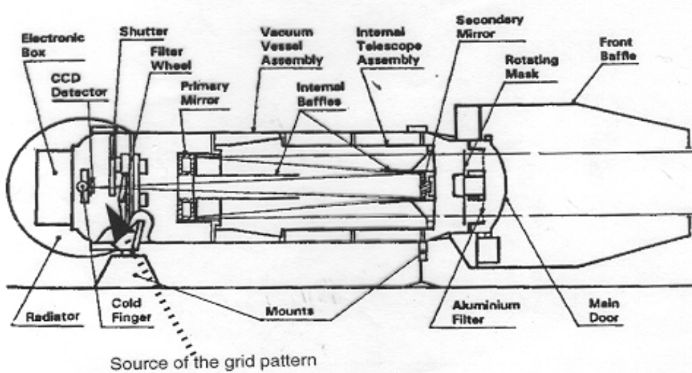
Figure III.3: Schéma de l'instrument EIT
