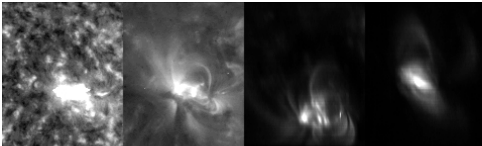
Figure IV.3: Comparaison d'images SOHO/EIT et CDS : (collaboration avec P. Young) De gauche à droite par température croissante (cf. Fig. II.12). Respectivement He II et Fe IX/X d'EIT; Mg IX et Fe XVI de CDS
