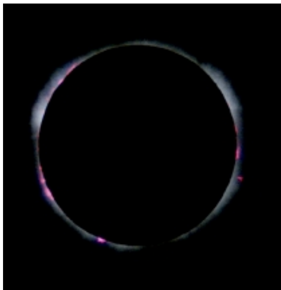
Figure II.1: Eclipse du Soleil du 11 Aout 1999 à Vouziers (France) : La Lune a caché pendant 2 minutes 14s la photosphère, rendant visible la couronne en blanc, des protubérances en rouge. Noter la forte activité coronale présente et la haute protubérance au Sud Ouest ( Photo personnelle ©Association NOVAE)
