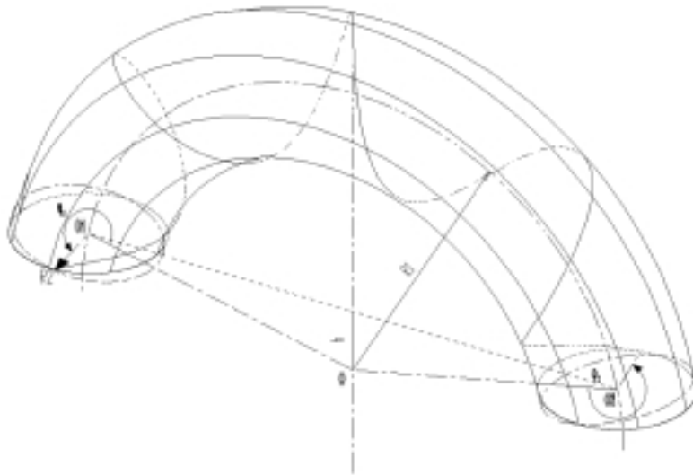
Figure IV.16: Définition des paramètres des boucles torsadées : r_0 le rayon principal du tore, h la hauteur du centre du tore par rapport à la surface, r_1 le rayon secondaire du tore, \Phi_1 et \Phi_2 les angles par rapport à une origine arbitraire de la position de la boucle par rapport à la coupe horizontale.
