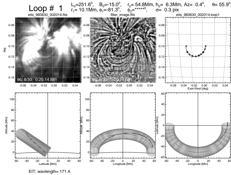
Figure IV.17: SOHO/EIT le 96-08-30 à 00h 20mn 14s (UT) boucle 1, Les parametres d'ajustement sont l_0 = 251.62 , b_0 = -15.02 , r_0 = 54.84 Mm, h_0 = 6.28 Mm, az = 0.45 , th = 55.86 , r_1 = 10.05 Mm, \phi_1 = -81.33 degrés, \phi_2 = -197.10 degrés. L'erreur mesurée entre le modèle et l'ajustement est \text{dev} = 0.32 pixel
