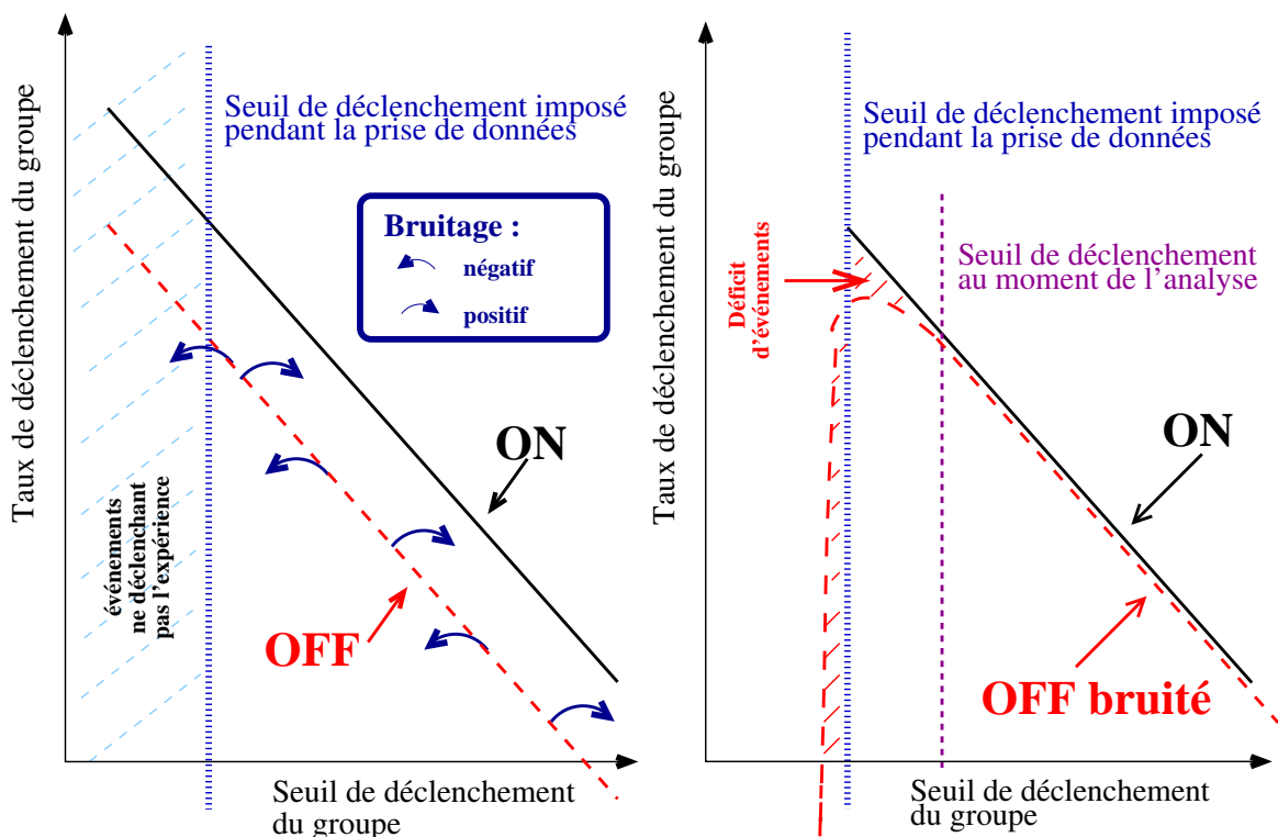
FIG. III.4 – Taux de déclenchement en fonction du seuil de déclenchement imposé [125]. On se place dans la partie Tcherenkov de la courbe (voir figure I.23 p. 38). À gauche : bruitage des données OFF. À droite : redéclenchement logiciel.
