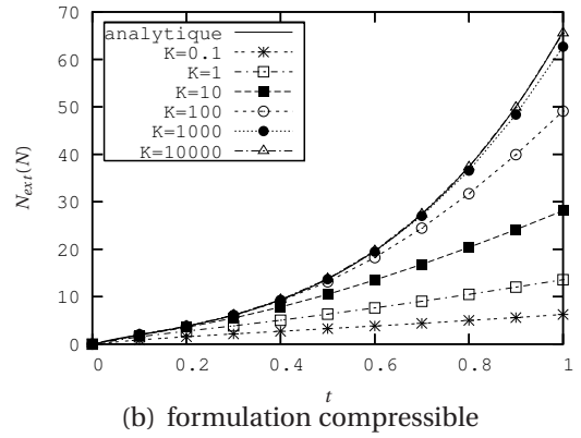
Figure 2.4 – Effort d'extension en fonction du paramètre de charge (Q9P3)
