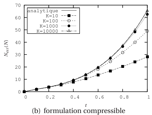
Figure 2.6 – Effort d'extension en fonction du paramètre de charge (H20P4)
