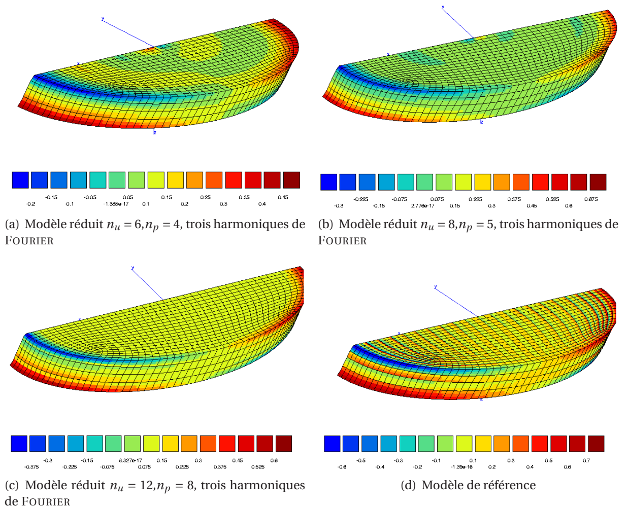
Figure 3.45 – Pression hydrostatique, cisaillement d'une lamelle tridimensionnelle
