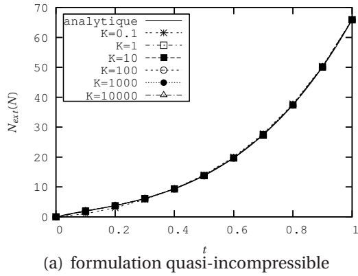
Figure 2.4 – Effort d'extension en fonction du paramètre de charge (Q9P3)
