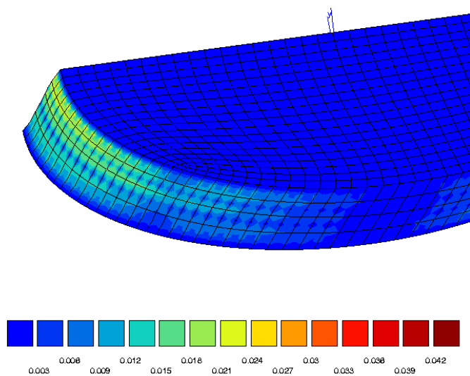
Figure 3.28 – Écart local er_u^{loc} , pour le modèle réduit 3D1D ( n_u = 9 , n_p = 3 , n_{\theta_u} = 3 , n_{\theta_p} = 3 )
