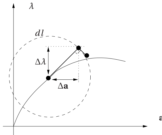
Figure 4.9 – Méthode à longueur d'arc linéarisé
