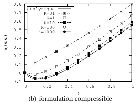
Figure 2.5 – Déplacement du bord externe en fonction du paramètre de charge (Q9P3)
