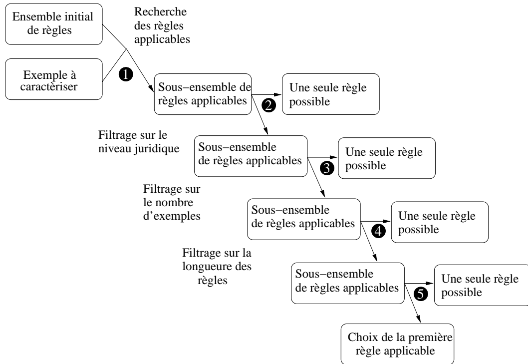
FIG. 9.4 – Procédé de gestion des règles.
