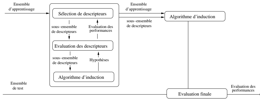
FIG. 5.3 – La méthode wrapper pour la sélection de descripteurs ([Kohavi & John, 1998]).
