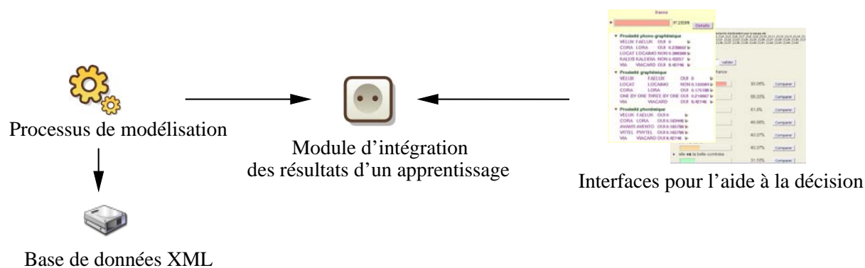
FIG. 11.18 – principe d'intégration à la plate-forme CATMIInE des résultats d'un apprentissage réalisé avec n'importe quel algorithme de modélisation.
