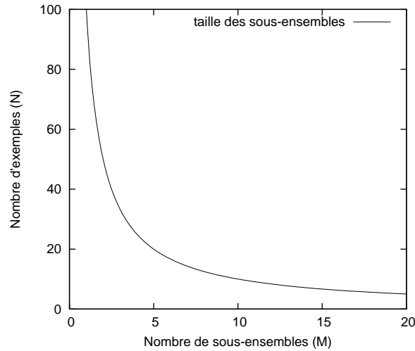
FIG. 3.1 – Évolution de la taille des ensembles d'apprentissage en fonction du nombre de paquets produits.
