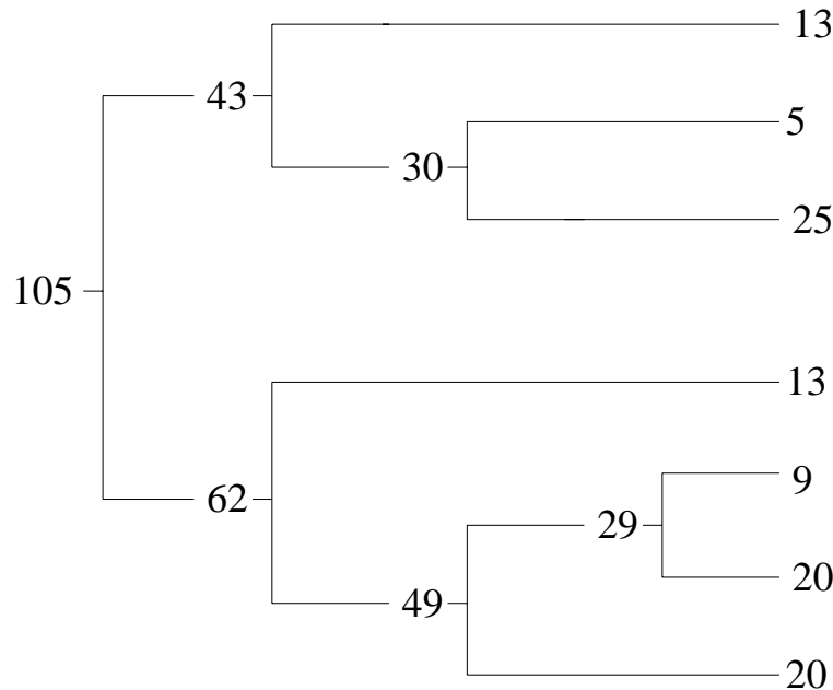
FIG. 3.3 – Dendrogramme des partitions associées aux regroupements obtenus sur la base de données de CATMIInE.
