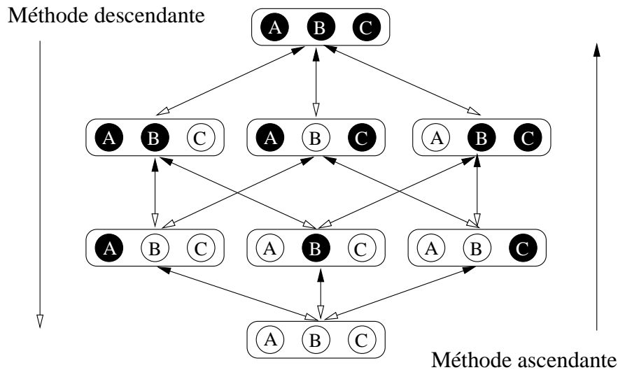
FIG. 5.2 – Principe ascendant ou descendant de sélection de descripteurs
