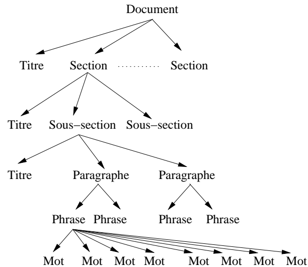
FIG. 1.2 – Exemple d’une structure logique d’un document dit “structuré”.
