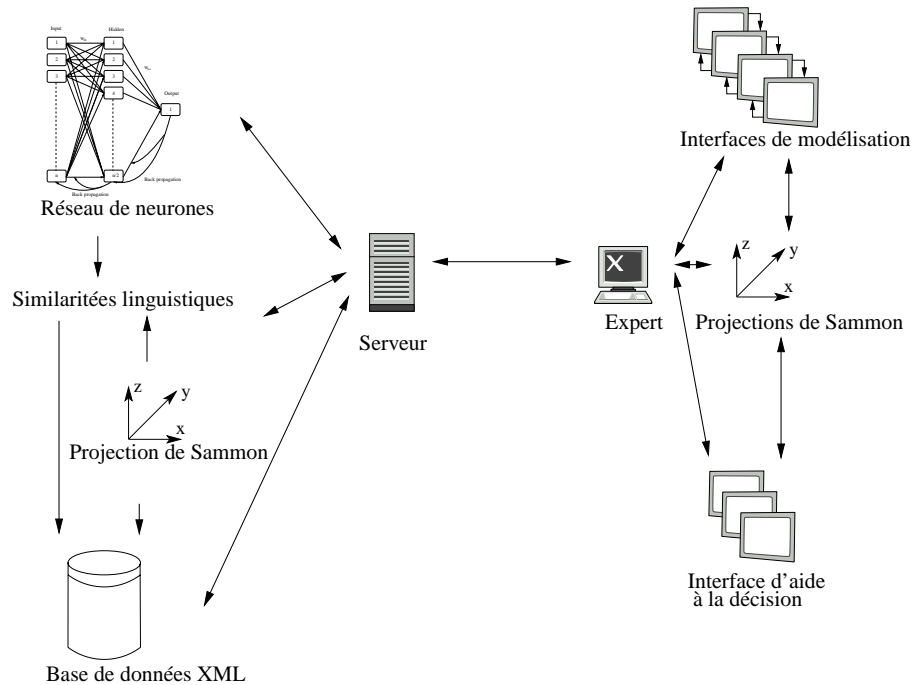
FIG. 11.2 – Architecture client serveur de CATMIInE
