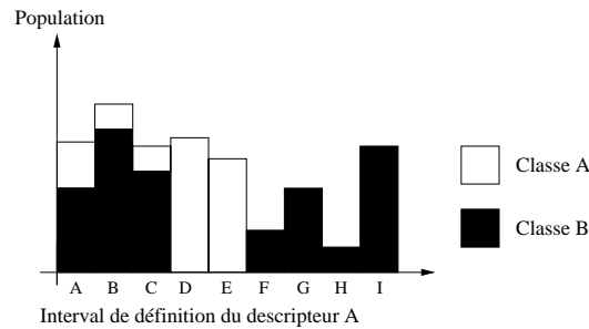
FIG. 4.2 – Étude de la répartition d’un descripteur A prenant ses valeurs dans le domaine de définition \{A; B; C; D; F; G; H; I\} .
