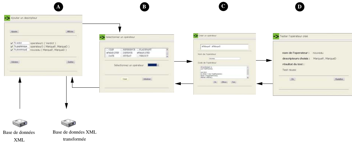
FIG. 11.9 – Processus de création d'une base de données intégrant le savoir-faire de l'expert.
