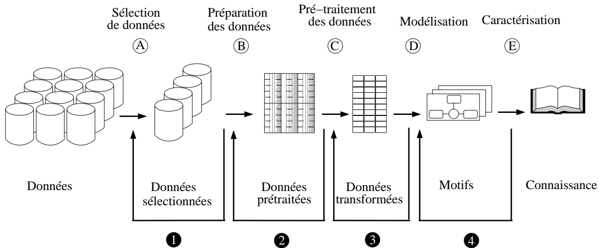
FIG. 8.2 – Principe de correction par retour sur le processus de fouille de données.
