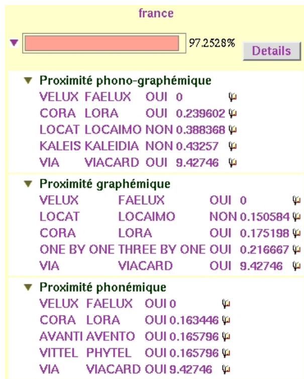
FIG. 11.3 – Résultats détaillés de la comparaison entre les marques Velux et Faelux pour la jurisprudence française
