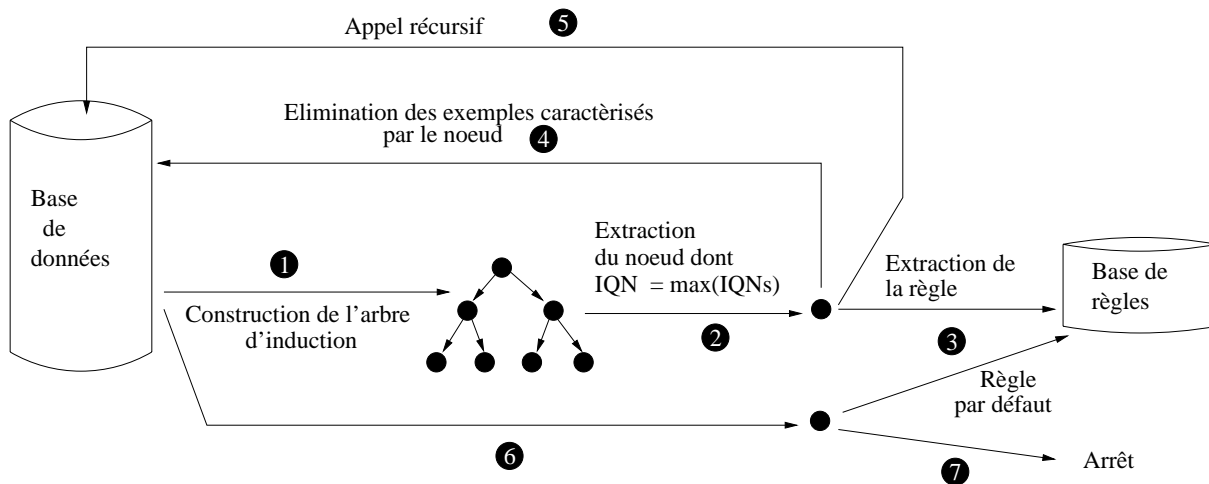
FIG. 9.2 – Principe récursif de DeTTMInE
