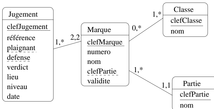
FIG. 11.14 – Modèle relationnel appliqué dans CATMI n E
