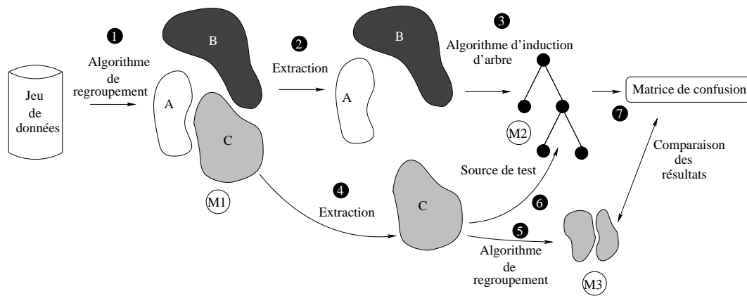
FIG. 7.2 – Processus d'évaluation de la connaissance dans CATMI n E.
