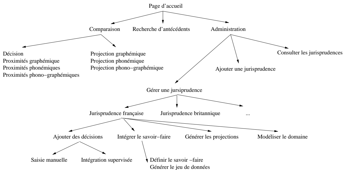
FIG. 11.6 – Vue d'ensemble de la plate-forme de modélisation CATMIInE.
