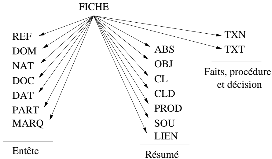
FIG. 4.3 – DTD de JURINPI.
