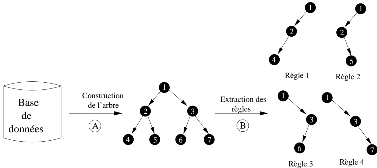
FIG. 6.1 – D'une base de données à des branches unaires.
