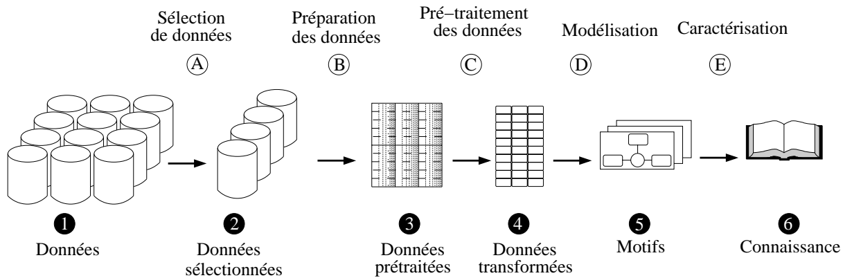
FIG. 2.1 – Vue d'ensemble des différentes étapes constituant la processus de fouille de données et d'extraction de connaissances.
