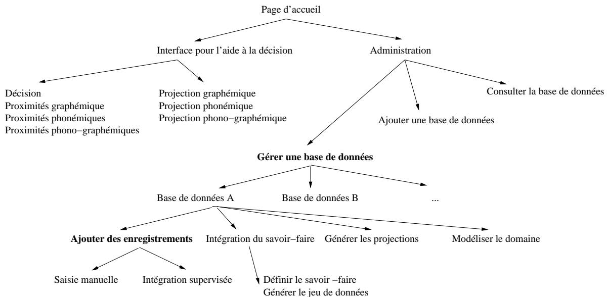
FIG. 11.16 – Vue générique de la plate-forme de modélisation CATMIInE.
