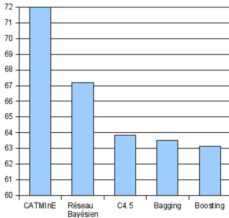
FIG. 9.1 – Taux de réussite sur une validation croisée
