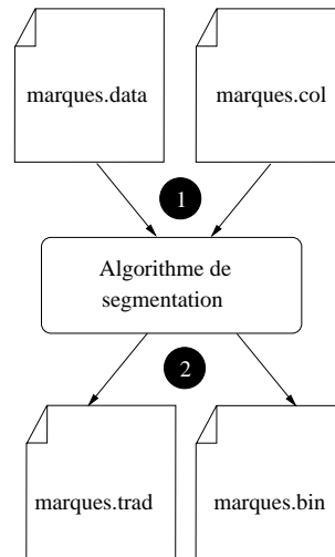
FIG. 10.4 – Principe de la segmentation des descripteurs d’une base de données.
