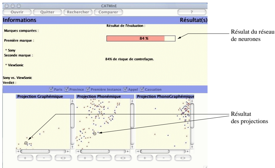
FIG. 11.1 – Résultats détaillés de la comparaison entre les marques Sony et Viewsonic pour la jurisprudence française
