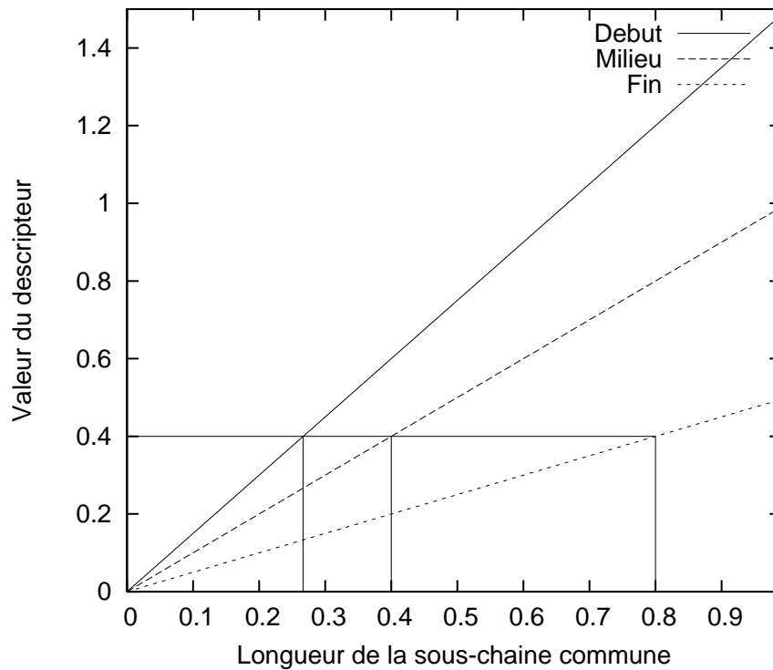
FIG. 10.3 – courbes représentatives des descripteurs présentés
