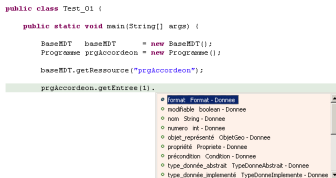
FIG. 6.7 – Saisie d'une expression en notation de type DOM avec Eclipse
