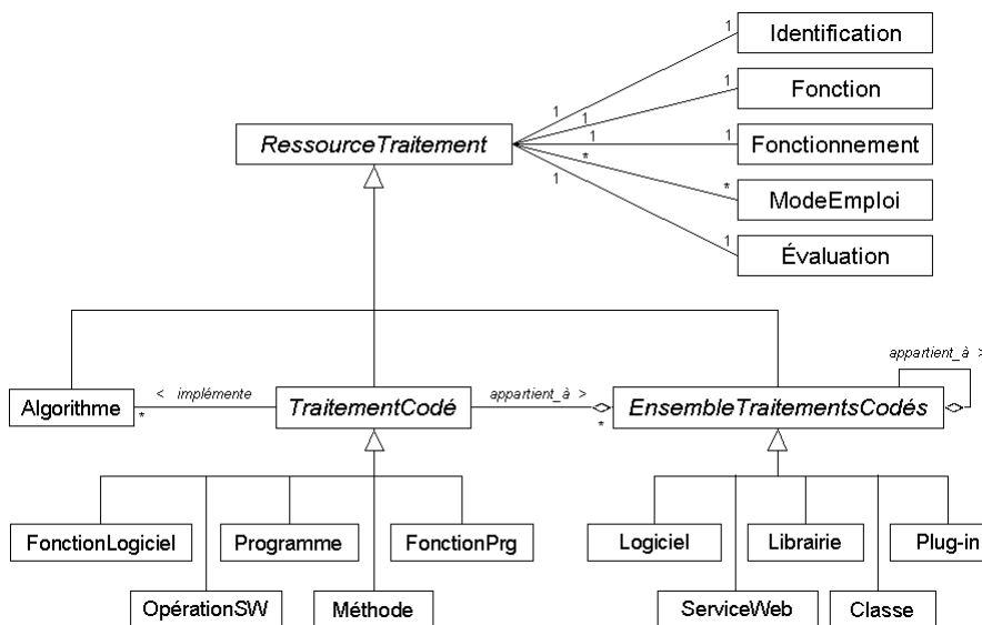
FIG. 2.18 – Classes principales du modèle de métadonnées
