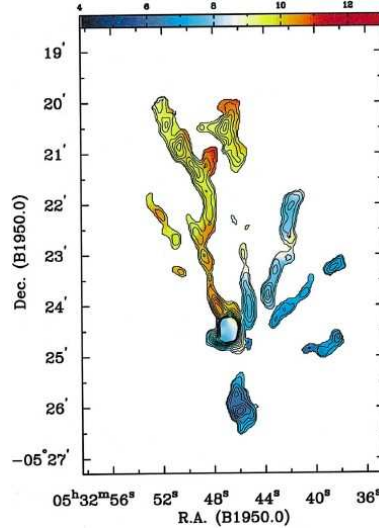
Fig. 2.8 – Les filaments d’ammoniac du flot moléculaire centrés sur la source IRC2 par Wiseman & Ho (1998). Les contours sont obtenus à partir des transitions de \text{NH}_3(\text{J,K})=(1,1) et (2,2) . L’échelle de couleurs indique la vitesse en \text{km s}^{-1} .
