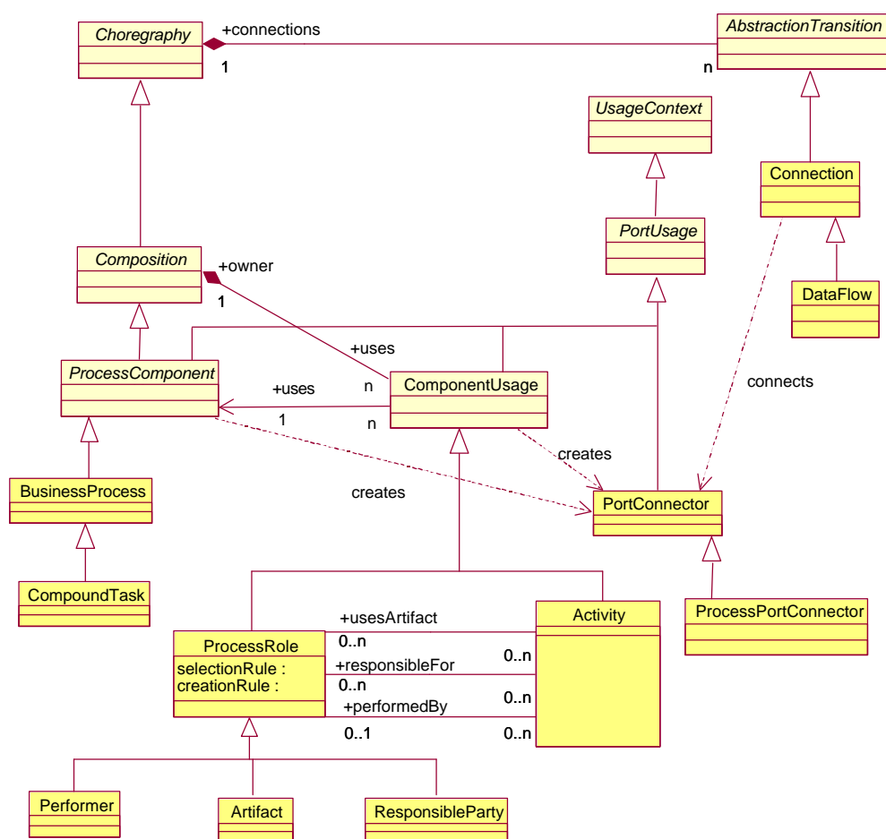
Figure 68 : Eléments extraits de la structure du méta-modèle du profil UML [(OMG/ECA 2004), figures 3-6 et 3-48]
