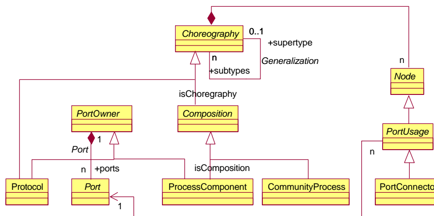
Figure 65 : Éléments extraits de la structure du méta-modèle du profil UML [(OMG/ECA 2004), figure 3-4]
