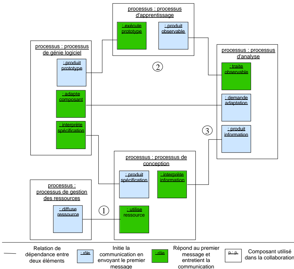
Figure 48 : Diagramme de collaboration UML de l'exemple 1
