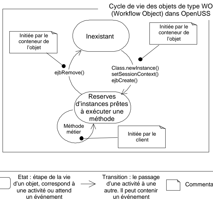
Figure 44 : Diagramme état-transition UML de l'objet considéré pour OpenUSS [(Monson-Haefel 2002), figure 12-1]
