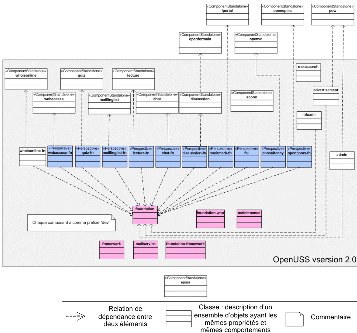
Figure 56 : Diagramme UML de classe des composants d'OpenUSS 51
